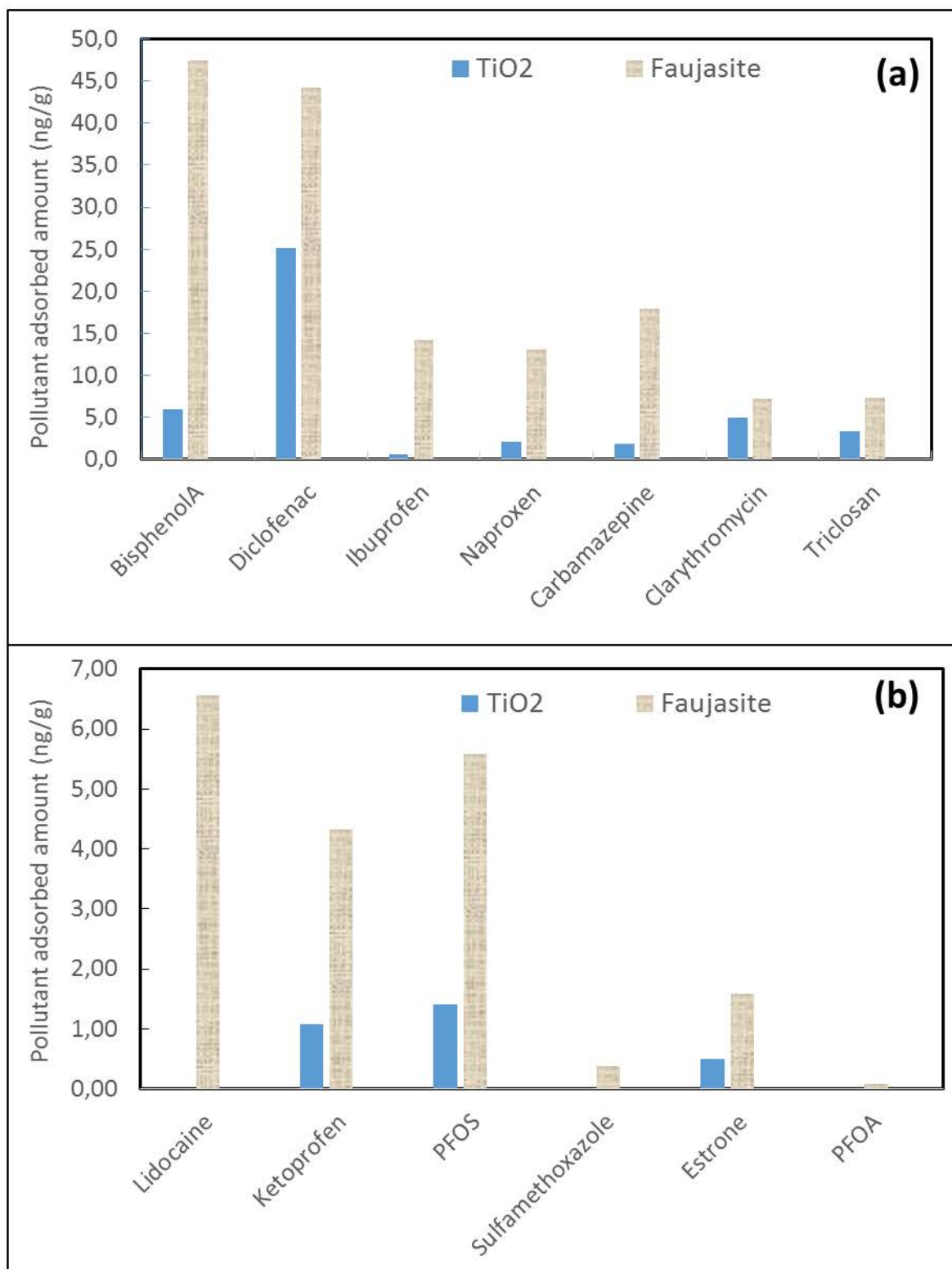
Fig. 14. Comparaison des quantités de micropolluants adsorbées sur le TiO 2 et la Faujasite modifiée.
