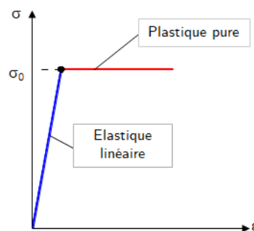
Figure 41 : Modèle de comportement élastoplastique des grains
