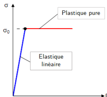
Figure 41 : Modèle de comportement élastoplastique des grains
