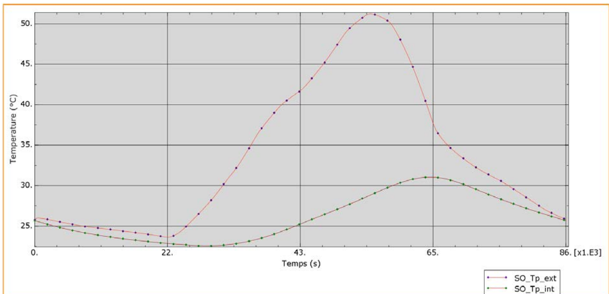
Figure 72 : Variation de température à travers l'épaisseur de paroi _ Sud-Ouest
