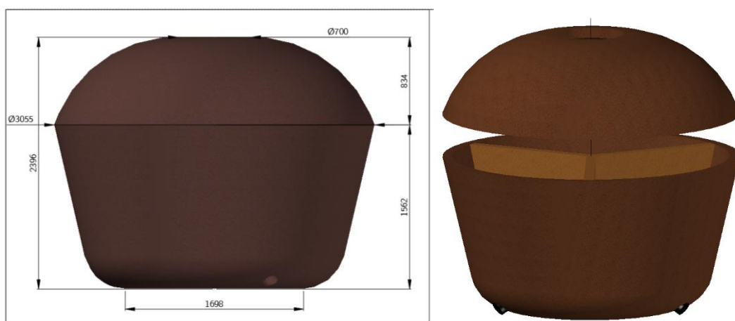
Figure 29 : Géométrie du grenier
