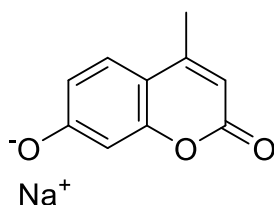
Ombelliférone
