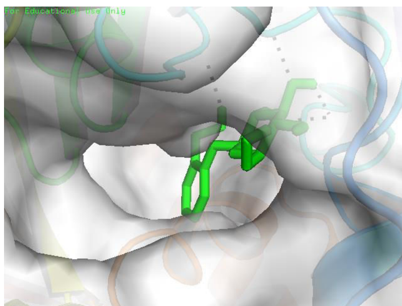
Figure 78: représentation des liaisons hydrogène formées par la molécule salicin et l'enzyme en noire. (Pymol)
