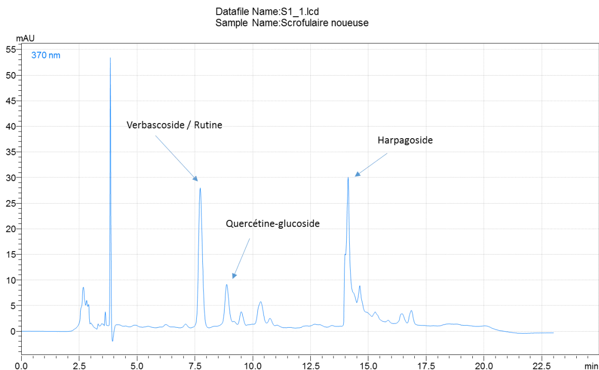
Figure 66 : Chromatogramme UV de la fraction 50-100 µm.
