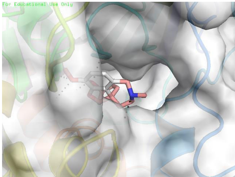
Figure 74: Représentation des liaisons d'hydrogènes formées entre la molécule galantamine et l'AChE en noire. (Pymol)
