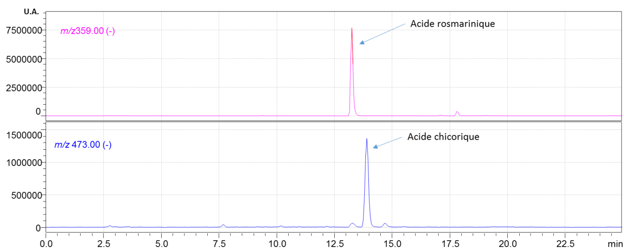
Figure 53 : Chromatogramme Acide rosmarinique et Acide chicorique, LC-ESI / MS en mode négatif (NT).
