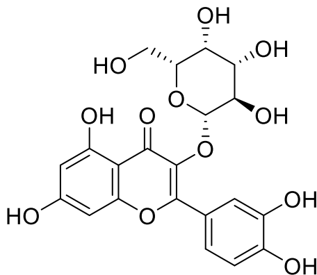
Hypéroside
