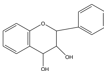
Flavandio
