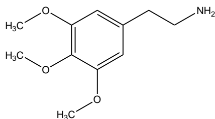
Mescaline
