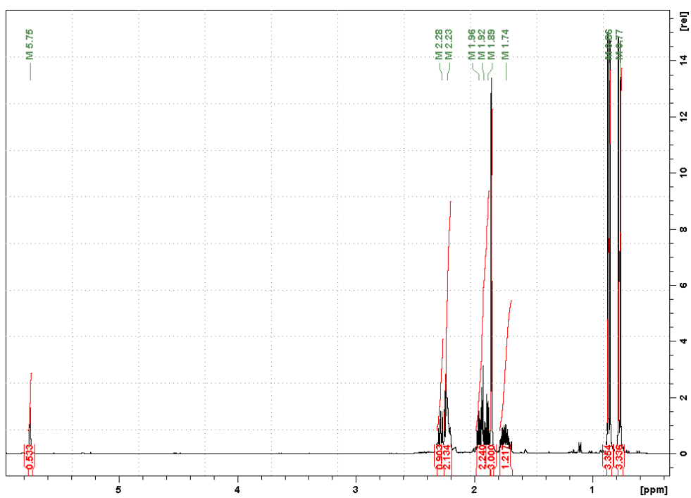
Figure D : Spectre du proton 1 H de la piperitone dans CDCl 3 à 400 MHz
