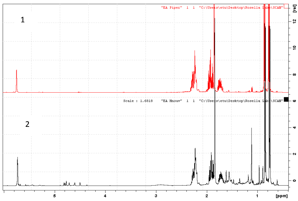
Figure 84 : Comparaison des spectres du proton 1 H entre la piperitone (1) et de l'huile essentielle C. commutatus (2) dans CDCl 3 à 400 MHz.
