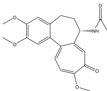
Colchine
