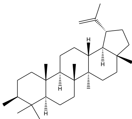
Lupéol
