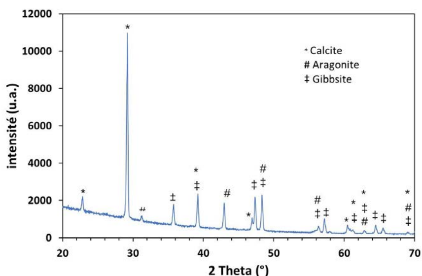
Figure IV-23 : diffractogramme RX du dépôt cathodique pour la solution CA
