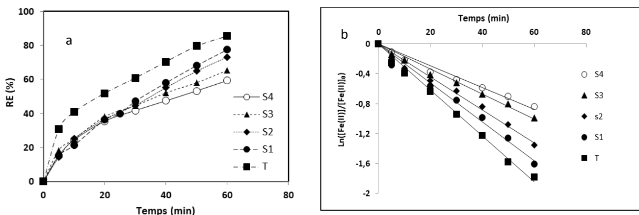
Figure II-8: Variation du (a) rendement d'élimination du Fe(II) et (b) \ln([Fe(II)]/[Fe(II)]_0) en fonction du temps pour les solutions T, S1, S2, S3, S4
