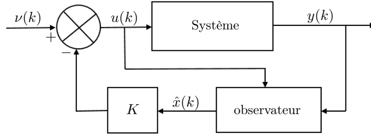
FIGURE 1.2 – Commande basée-observateur
