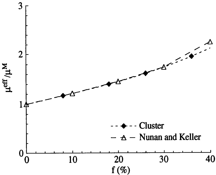
Figure III.1 : Module de cisailment normalisé dans la direction principale de symétrie cubique pour une distribution cubique simple de sphères rigides. Les résultats obtenus par la méthode du cluster sont comparés avec les résultats analytiques de Nunan et Keller (1984).
