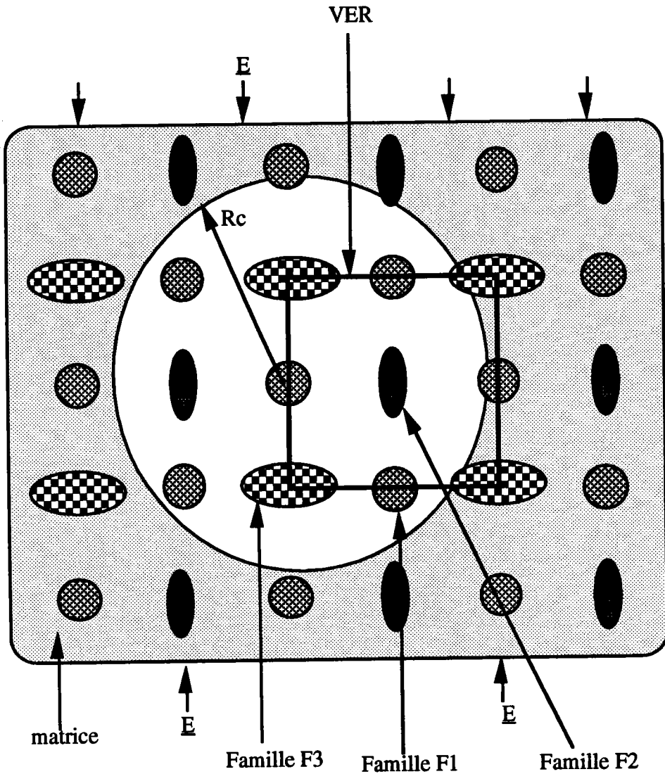
Figure II.5 : Représentation schématique du cluster de rayon R_c dans le cas d'une distribution de trois familles d'inclusions et du volume élémentaire représentatif (VER).
