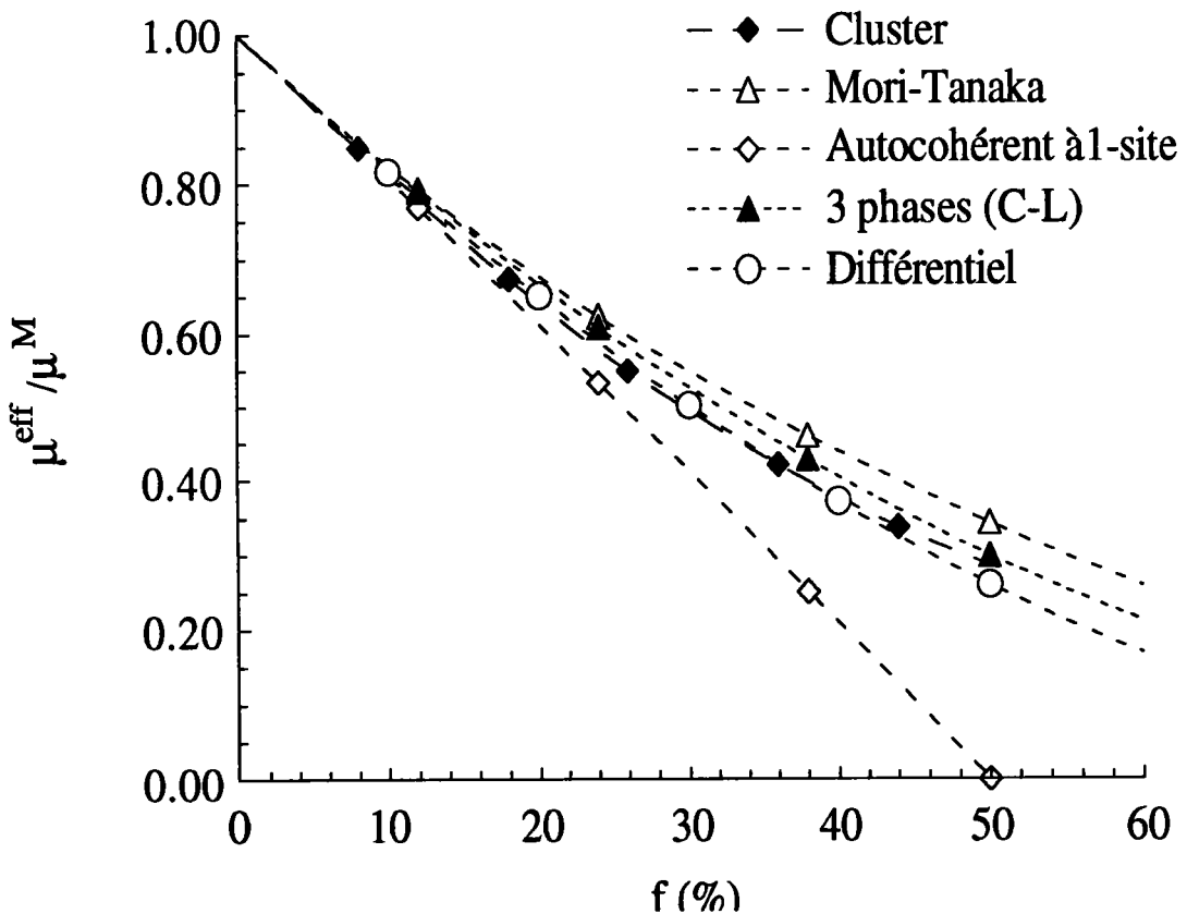
Figure III.6 : Comparaison des résultats de la méthode du cluster, pour une distribution de vides sphériques sur un réseau cubique simple, avec les modèles de Mori-Tanaka, autocohérent à 1-site, à trois phases et différentiel.
