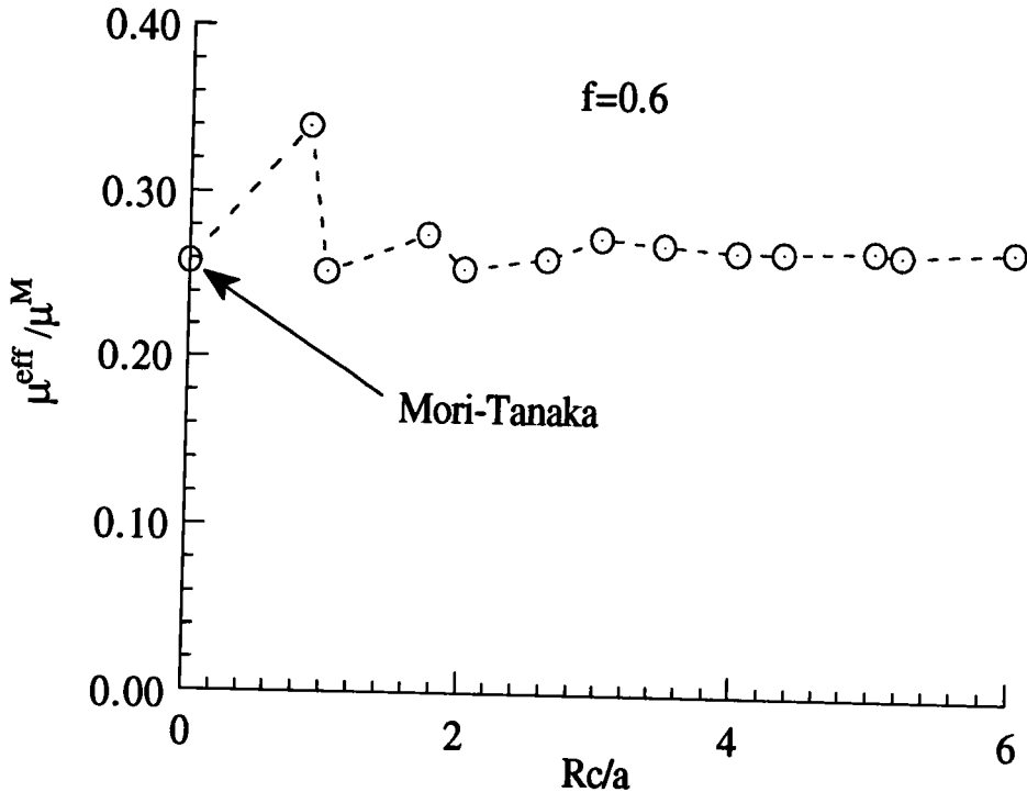
Figure II.10 : Convergence de la méthode du cluster pour des valeurs croissantes du rayon R_c du cluster. On considère une distribution de vides sphériques sur un réseau cubique centré.
