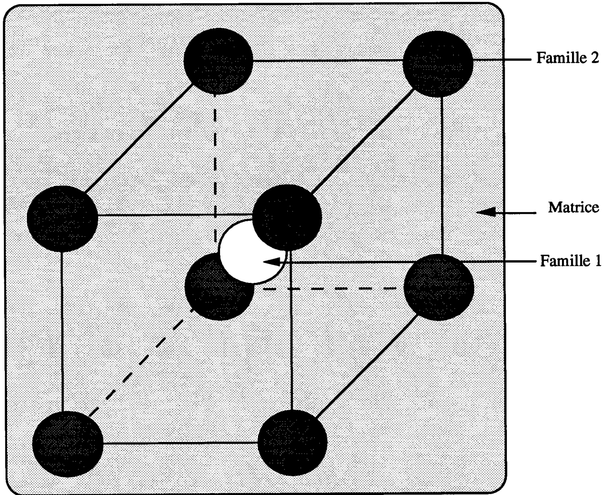
Figure II.14 : Représentation d'une distribution de deux familles d'inclusions F_1 et F_2 sur un réseau cubique centré présenté sur la figure II.17.
