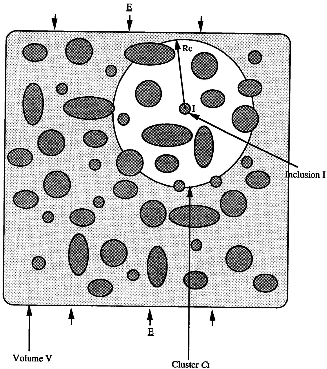
Figure II.16 : Représentation schématique d'un milieu inclusionnaire non périodique, et du cluster de rayon R_c .
