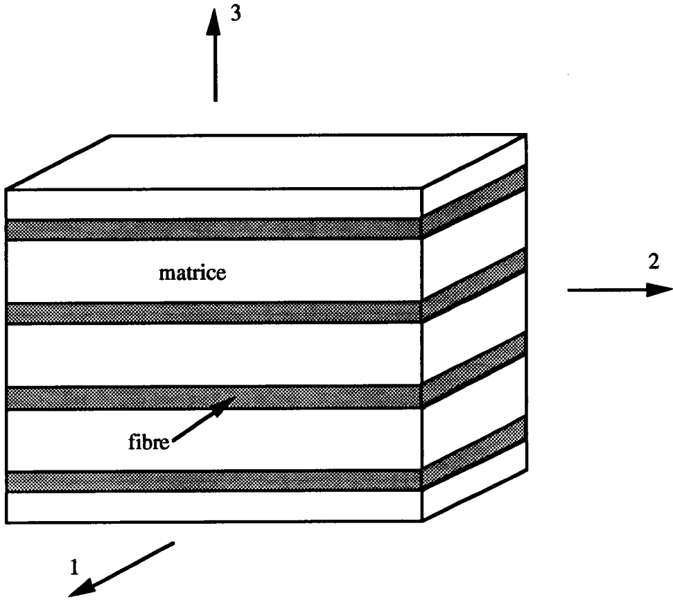
Figure II.25 : Représentation schématique par couches d'un composite unidirectionnel.
