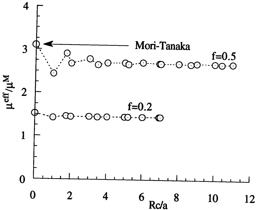
Figure II.9 : Convergence de la méthode du cluster pour des valeurs croissantes du rayon R_c du cluster. On considère une distribution de sphères rigides sur un réseau cubique simple.
