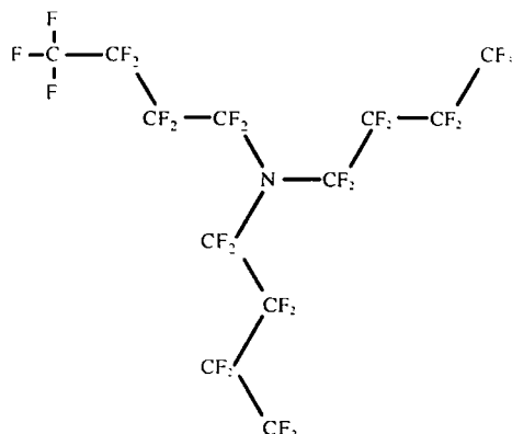
Figure 3 : PFTBA
