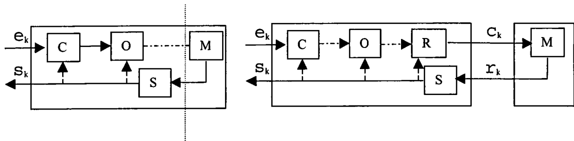
Figura 3.2: Partes Lógica e Física do Chão de Fábrica
