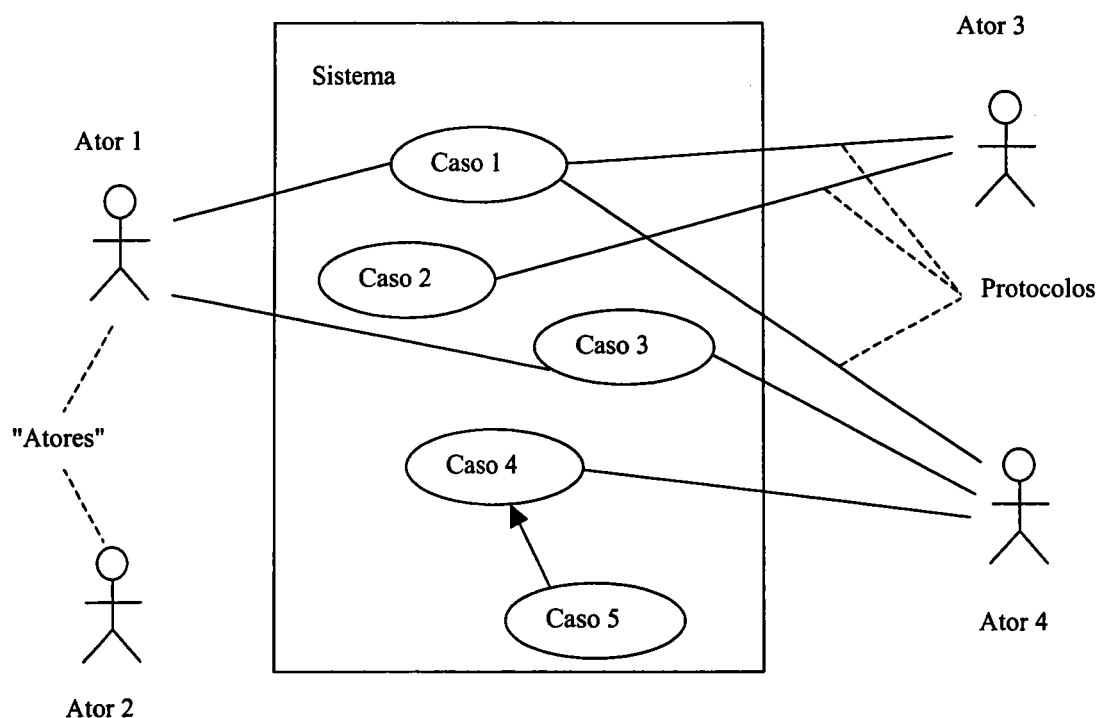
Figura 3.9: Diagrama de Uso : [Douglass 98]
