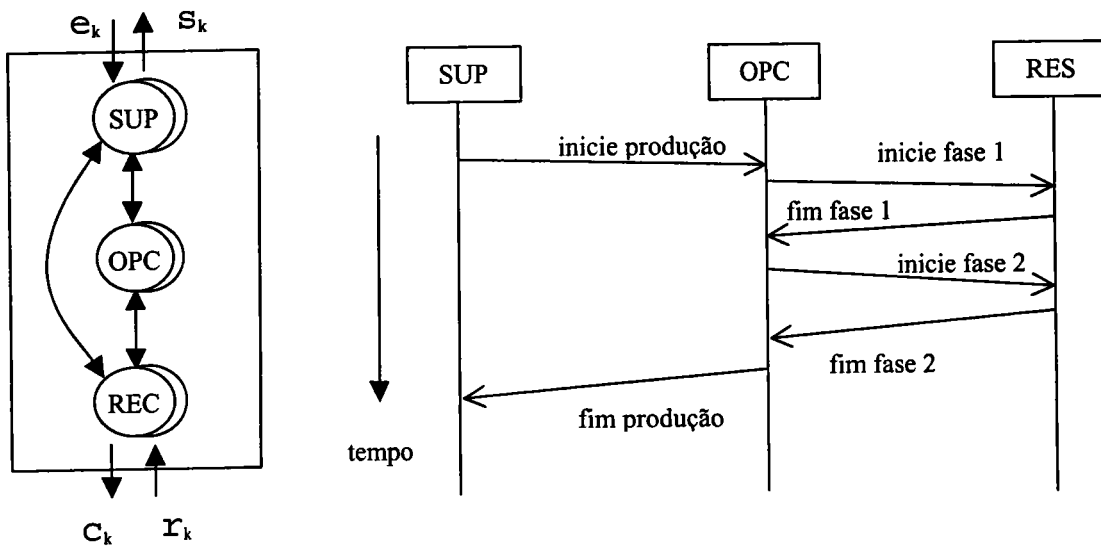
Figura 3.10: Diagrama de Seqüência
