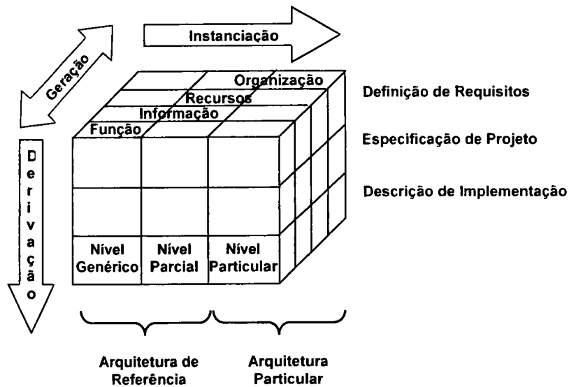
Figura 2.9: Quadro de Modelagem CIMOSA: [Vernadat 96]
