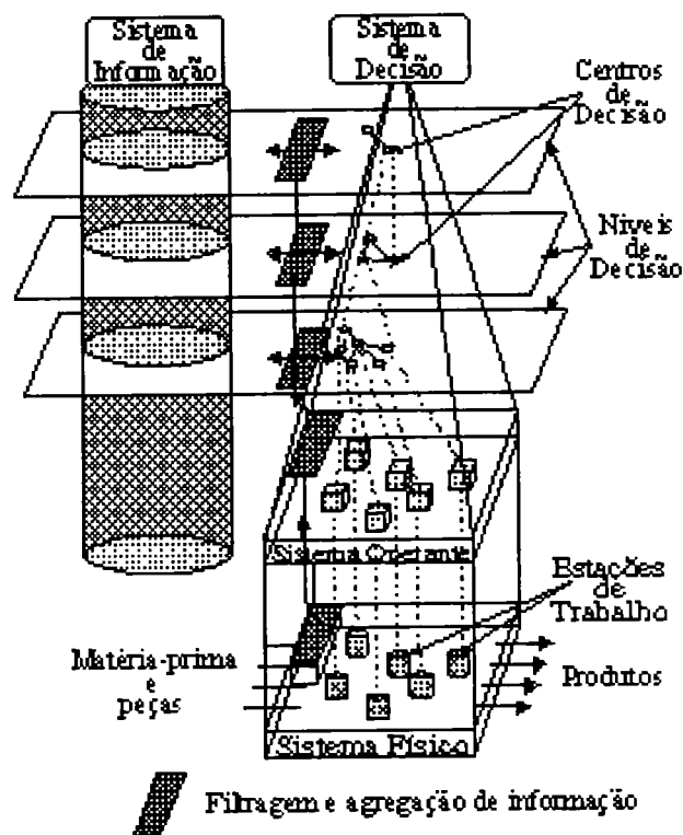
Figura 2.3: Modelo de Referência GRAI [Doumeingts 95]
