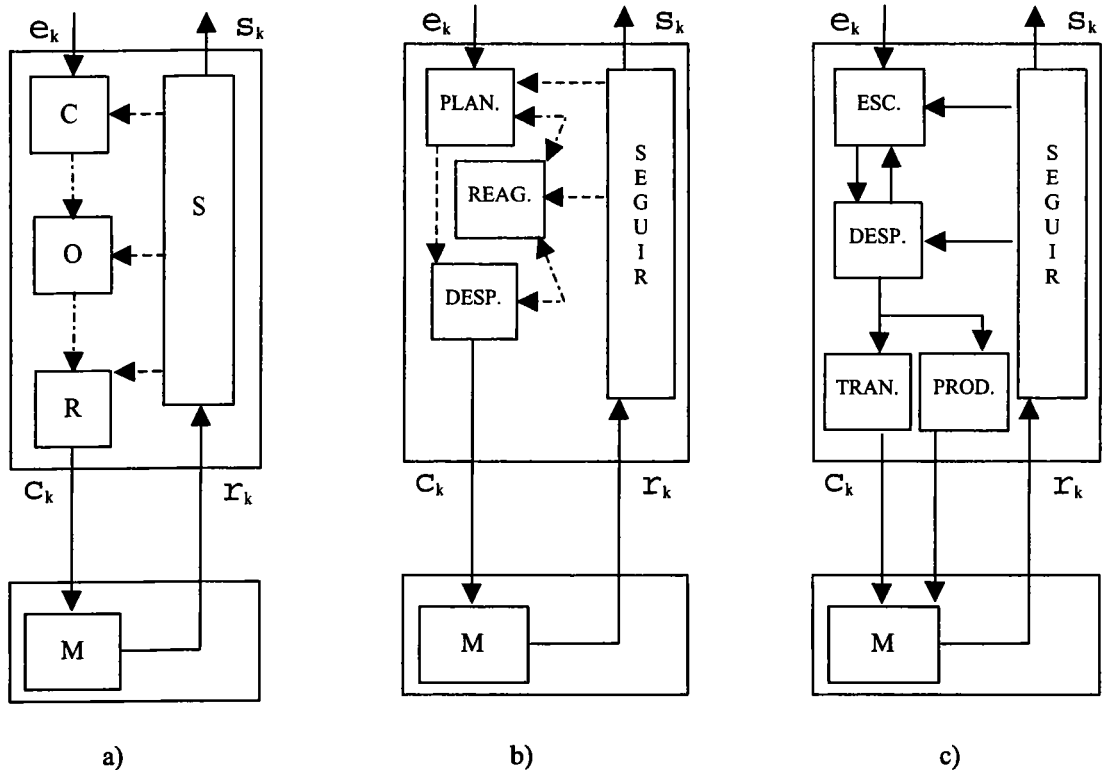
Figura 3.3: Arquitetura Lógica X PAC [Huguet 95] X PAC [Bauer 94]
