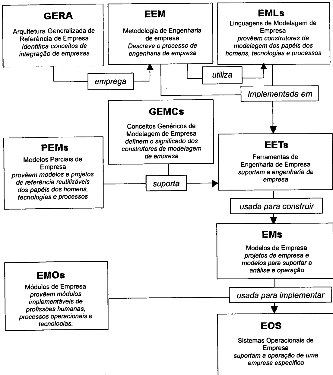
Figura 2.11: Componentes de GERAM : [ISO 98]
