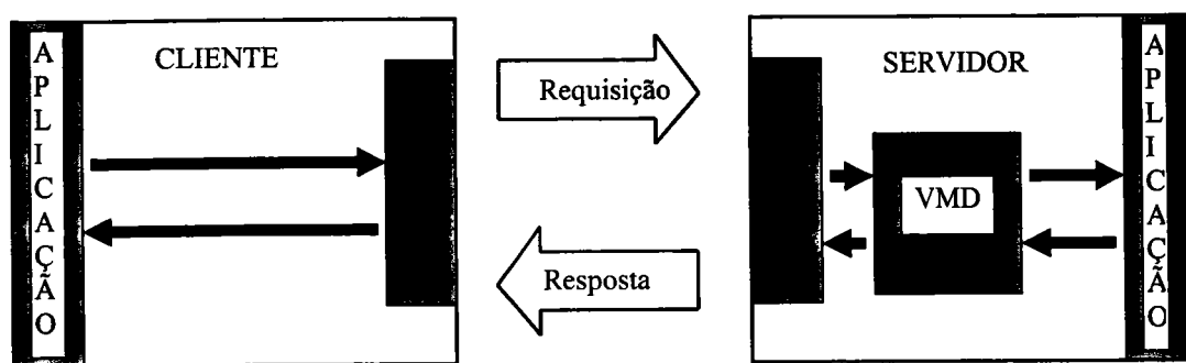
Figura 2.12: Relação Cliente/Servidor no MMS
