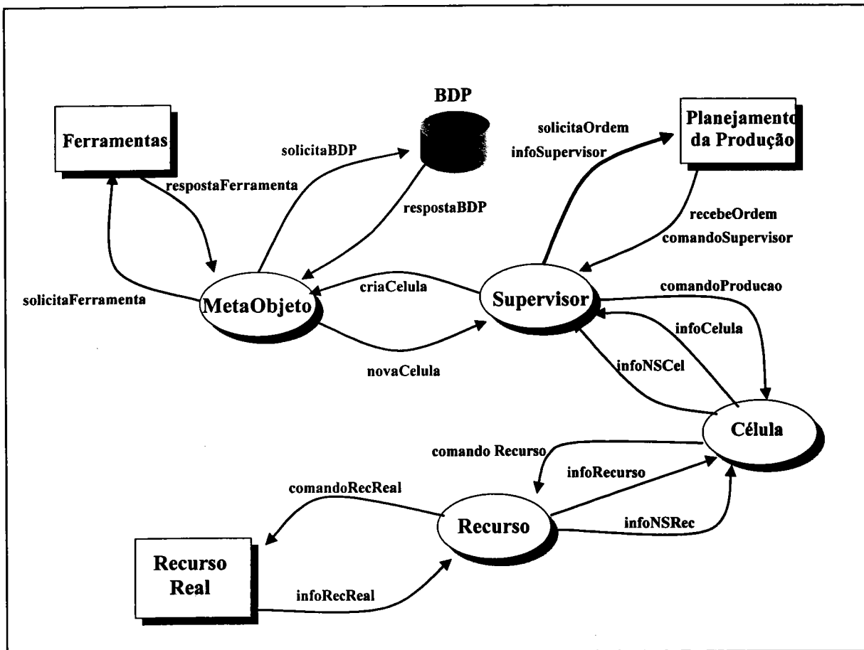
Figura 4.4: Diagrama Geral de Syroco-2
