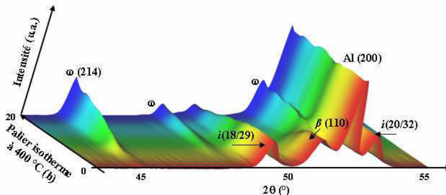
Figure II.14 : Vue en perspective des diffractogrammes de l'alliage Alpur/(30 % vol. \text{Al}_{59}\text{Cu}_{25,5}\text{Fe}_{12,4}\text{B}_3 )p compacté à froid pendant un maintien isotherme à 400 °C. La durée totale du palier correspond à 20 h. La transformation ( i et \beta ) + Al \rightarrow \omega est visualisable par la diminution progressive des pics principaux des phases i et \beta associée à l'apparition puis l'augmentation de ceux de la phase isostructurale à \omega - \text{Al}_{70}\text{Cu}_{20}\text{Fe}_{10} . Les couleurs ne servent qu'à faciliter la visualisation.
