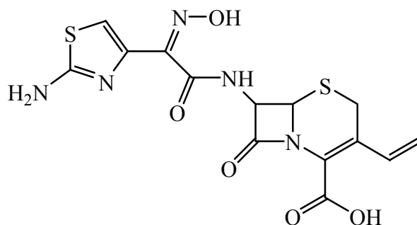
Fig. 3 Cefdinir
