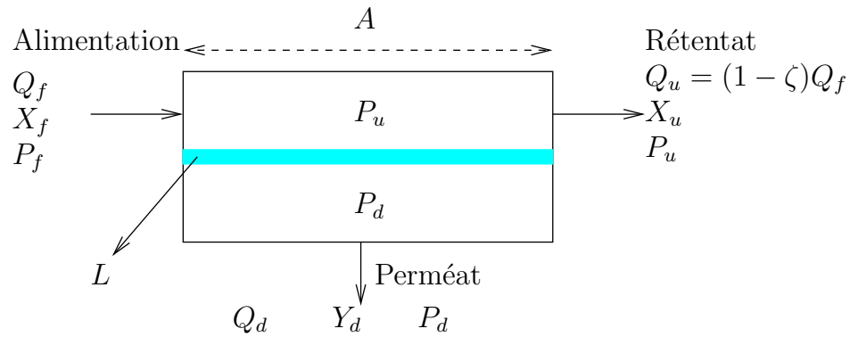
Figure E.1: Schéma d'un procédé membranaire conventionnel pour la séparation gazeuse
