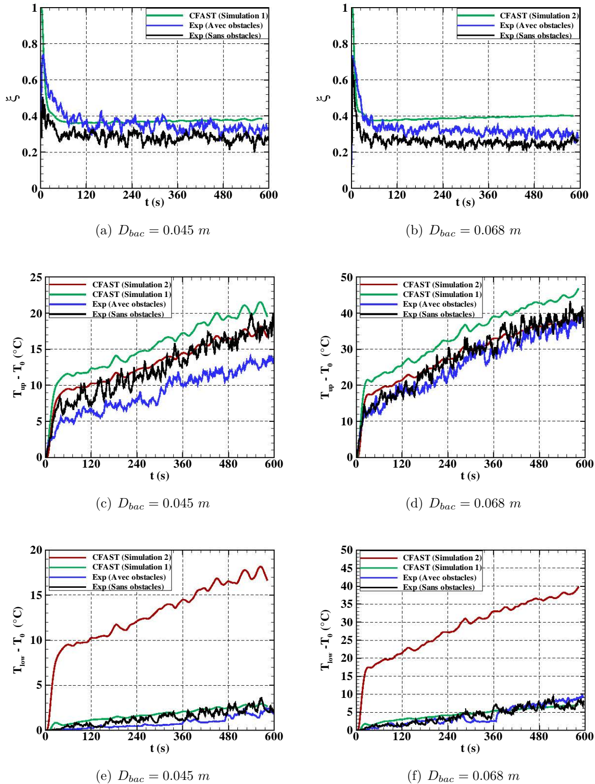
FIGURE 5.21 – Comparaison des résultats de CFAST aux résultats expérimentaux obtenus dans la cage d’escalier.
