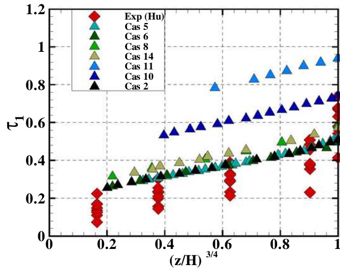
FIGURE 3.15 – Variation du temps adimensionné de montée du front de panache en fonction de (z/H)^{3/4} .
