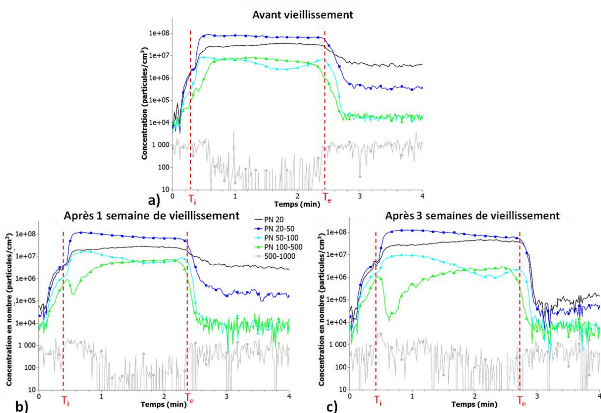
Figure 120 : Concentration en particules fines émises au cours de la combustion d'échantillons M 50/50 avant (a) et après 1 (b) et 3 semaines de vieillissement (c)
