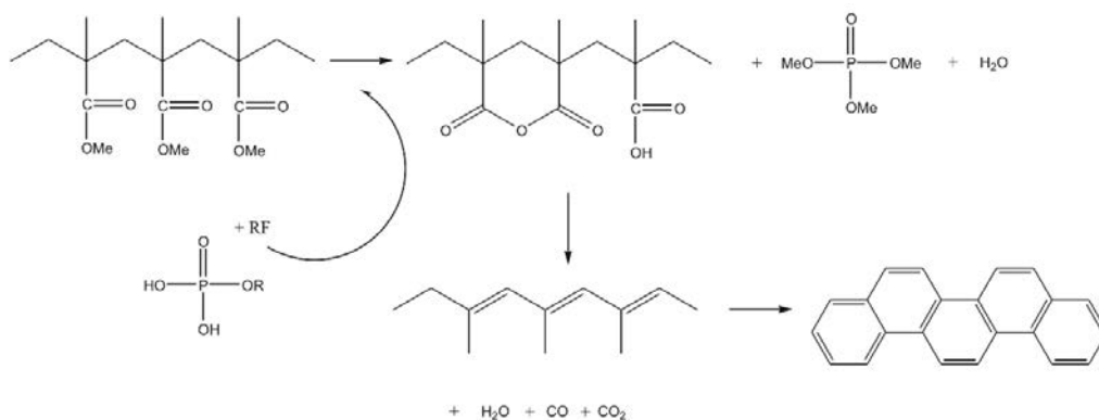
Figure 48 : Mécanisme de formation du char
