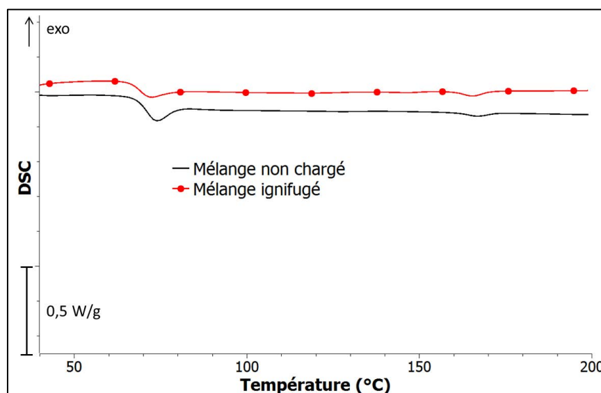
Figure 90 : DSC des mélanges 50/50 mis en œuvre par injection (1 er scan)
