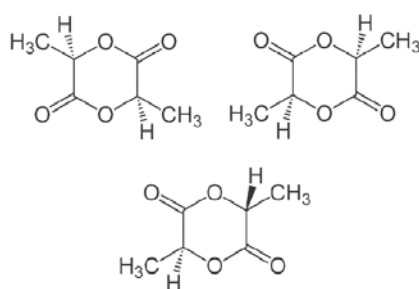
Figure 26 : Les trois stéréo-isomères du lactide (haut gauche : D-Lactide, haut droite : L-Lactide, bas : Mésolactide)
