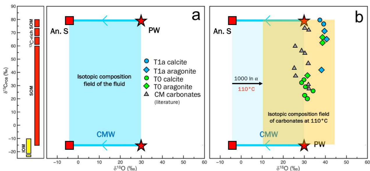
Fig. 4-1 a) & b) Simplification du modèle isotopique proposé lors de cette étude pour expliquer la variabilité des compositions en \delta^{18}\text{O} - \delta^{13}\text{C} mesurées dans les carbonates des chondrites CM. An. S : silicates anhydres, CMW : l'eau des CM, PW : l'eau primordiale, SOM : la matière organique soluble, IOM : la matière organique insoluble.
