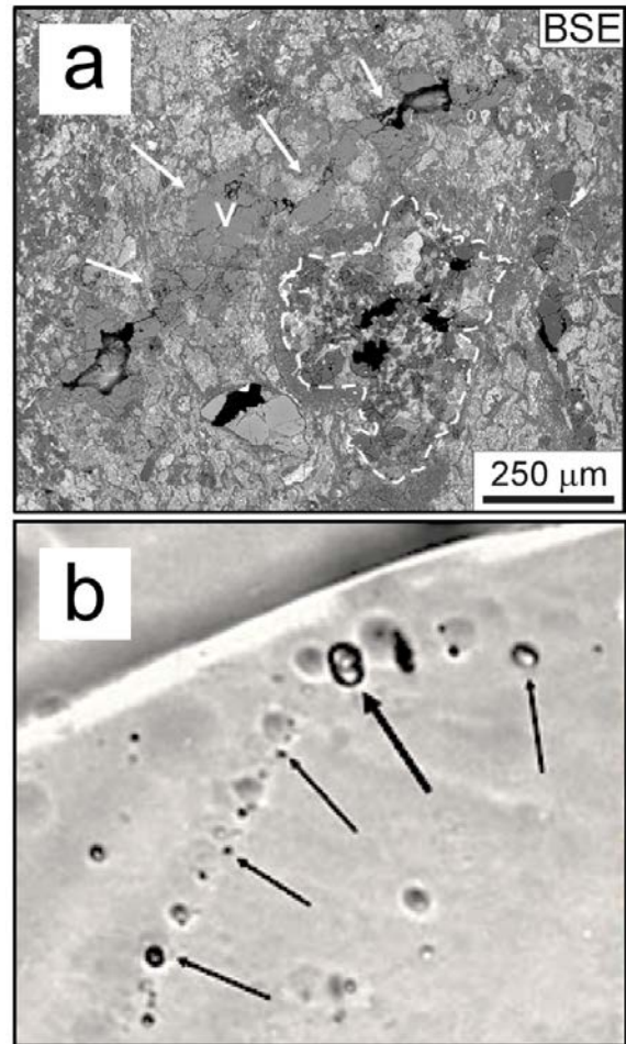
Fig. 1-17 a) Image MEB d'une veine de calcite (V) dans la chondrite CM LON 94101 (Lingren et al., 2011). b) Photographie d'inclusions fluides piégées dans un carbonate d'une chondrite CI (Zolensky, 2010).
