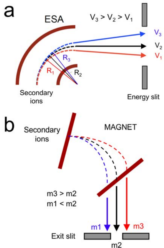
Fig. 2-14 Représentation schématique de la trajectoire des ions secondaires accélérés dans le secteur (a) électrostatique et (b) magnétique ((a) : figure modifiée source : www.geoscience.wisc.edu ).
