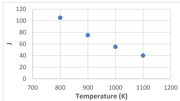
Figure 98 : Evolution de J avec la température (P=1,067 bar, temps de passage de 2 s, gaz vecteur : hélium, traceur : argon)
