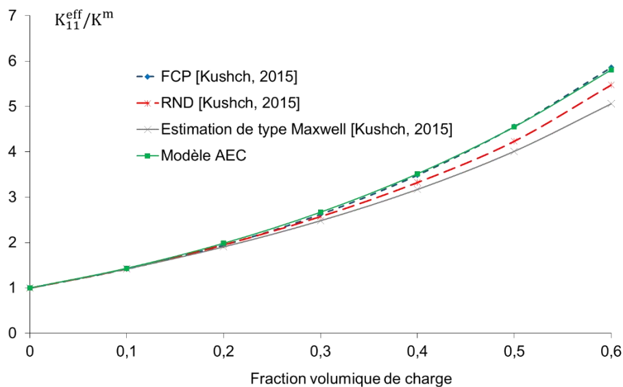
Figure 26 : Comparaison du modèle AEC avec interface imparfaite aux modèles de Kushch (Kushch et al. 2015)
