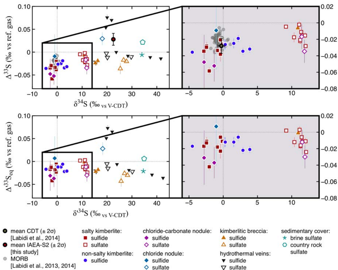
Figure V-2: Compositions multi-isotopiques des échantillons, reportées dans les espaces \delta^{34}\text{S} - \Delta^{33}\text{S} (haut) et \delta^{34}\text{S} - \Delta^{33}\text{S}_{\text{eq}} (bas).
