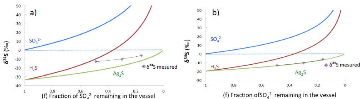
Figure II-8: Modèles de distillation de Rayleigh appliqué à des tests d'extraction de sulfates avec des rendements variables (d'après D'Eyrames, 2014). (a) Un fractionnement isotopique de 34‰ en \delta^{34}\text{S} , calculé pour un fractionnement isotopique à l'équilibre isotopique entre \text{SO}_4^{2-} et \text{H}_2\text{S} (Miyoshi et al., 1984, Ohmoto & Rye, 1979) à \sim 180^\circ\text{C} (température du chauffage) ne reproduit pas les compositions isotopiques mesurées. (b) Un fractionnement isotopique de 20‰ en \delta^{34}\text{S} entre \text{SO}_4^{2-} et \text{H}_2\text{S} correspond aux compositions isotopiques mesurées.
