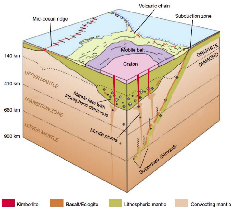
Figure B: Coupe schématique montrant les relations entre un craton continental, sa racine lithosphérique, la zone de stabilité du diamant et le manteau convectif. Des portions de croûte océanique recyclée (basalte / éclogite) sont présentes dans la racine cratonique où les diamants sont stables, et peuvent être échantillonnées par les éruptions de kimberlites. Référence: Shirey et al. (2013).
