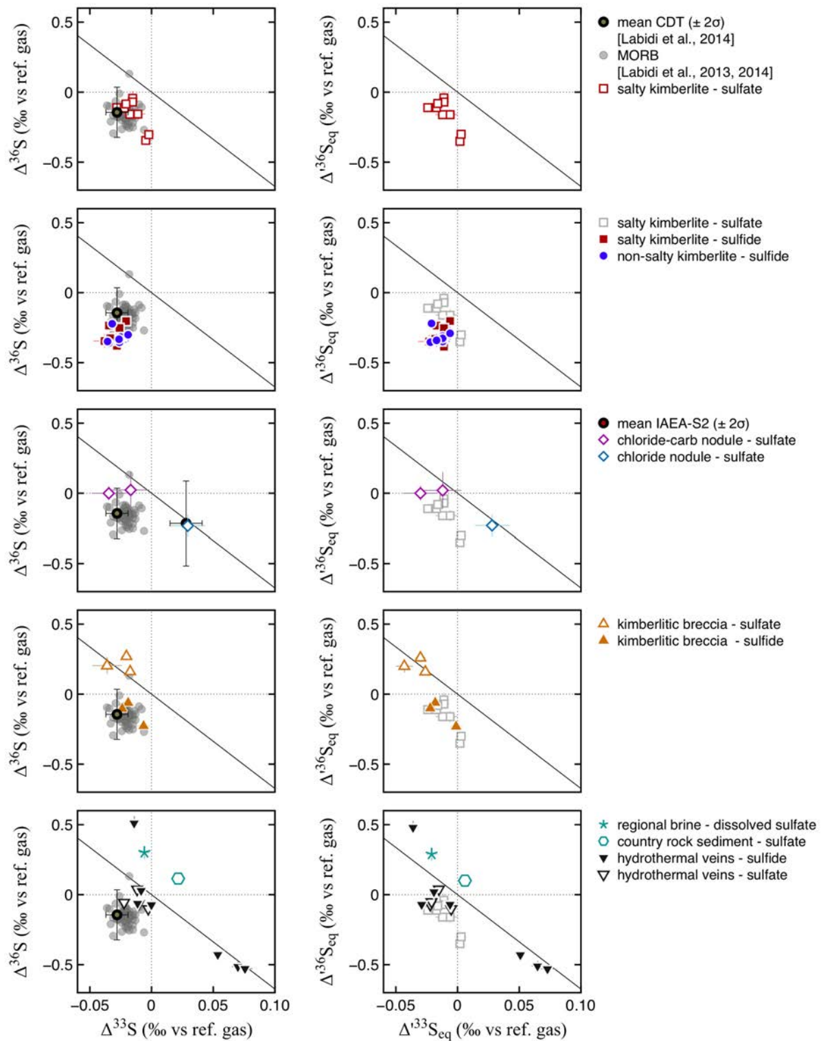
Figure V-3: Compositions multi-isotopiques des échantillons, reportées dans les espaces \Delta^{36}S - \Delta^{33}S (gauche) et \Delta^{36}S_{eq} - \Delta^{33}S_{eq} (droite). La droite noire passant par l'origine indique la pente de \sim -7 , caractéristique des fractionnements dépendants de la masse.
