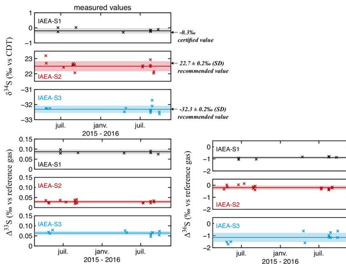
Figure II-10 : Mesures sur le long terme (2015-2016) des trois standards internationaux de sulfure d'argent, pour les périodes où nous avons effectué nos mesures, soit entre avril et septembre 2015 et 2016. Les lignes de couleur représentent les moyennes des mesures pour chaque standard et les plages de couleur l'écart-type ( 1\sigma ) autour des moyennes.
