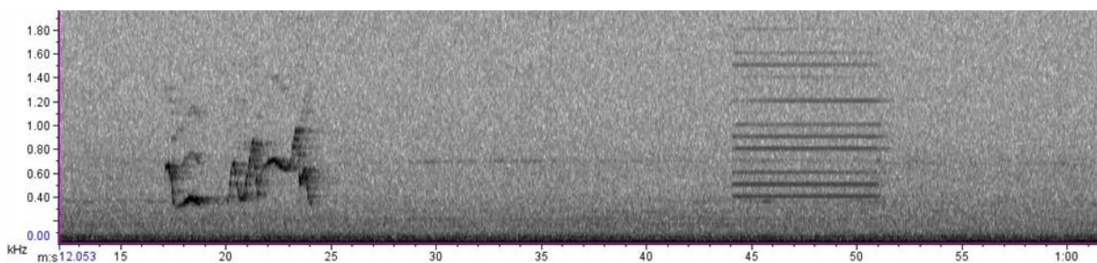
Figure 7 : Spectrogramme représentant les deux sons synthétiques émis puis enregistrés par un SM3 en milieu de plaine ; à gauche : son modulé ; à droite : son plat (logiciel Raven Pro – Charif et al. 2010).
