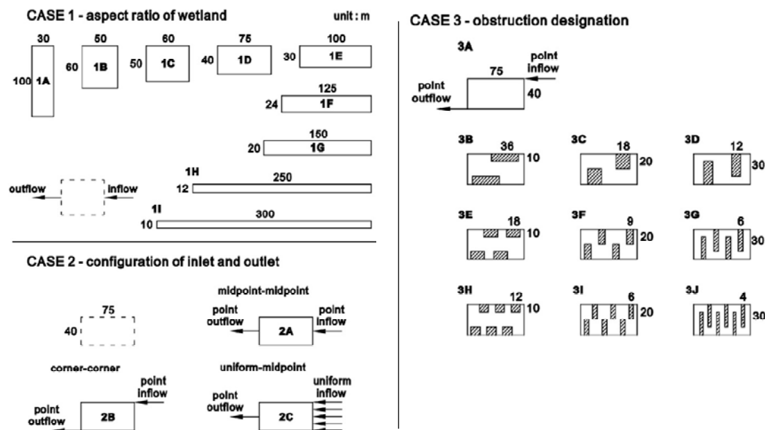
Figure A-10: Détails des différents cas étudiés par l'étude de Su et al. (2009) concernant : le ratio longueur/largeur de la ZTVA (case 1), la configuration entrée/sortie de l'eau dans la ZTVA (case 2) et les différentes configurations des obstacles dans la ZTVA (case 3).
