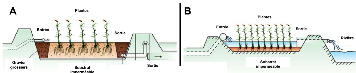
Figure A-5: Configuration d'une zone tampon à (A) écoulement de subsurface vertical et à (B) écoulement de surface libre (Kadlec et Knight, 1996).
