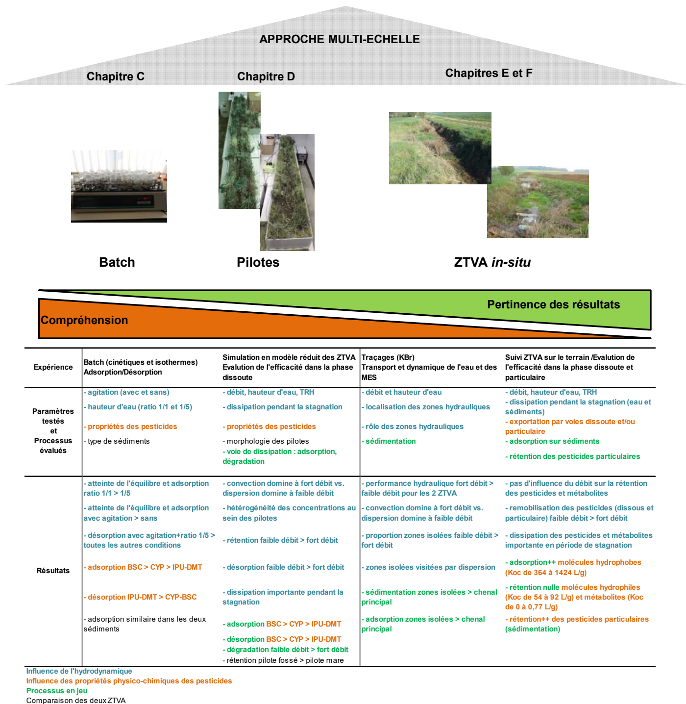
Figure F-1: Résumé de l'approche expérimentale utilisée et des résultats obtenus lors du suivi des deux ZTVA sur le terrain pendant trois années.
