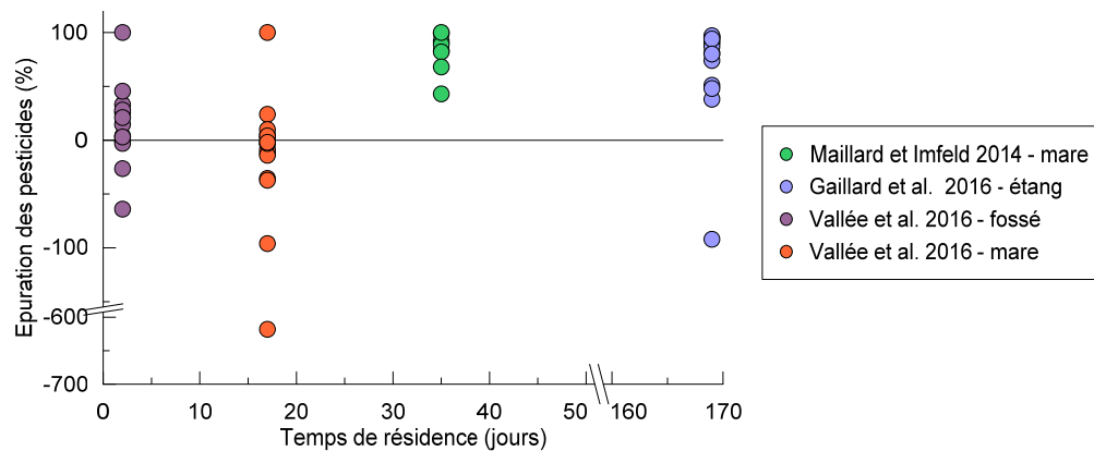
Figure A-11: Pourcentage d'épuration des pesticides mesuré dans 4 ZTVA en fonction du temps de résidence hydraulique maximale mesurée (TRH).
