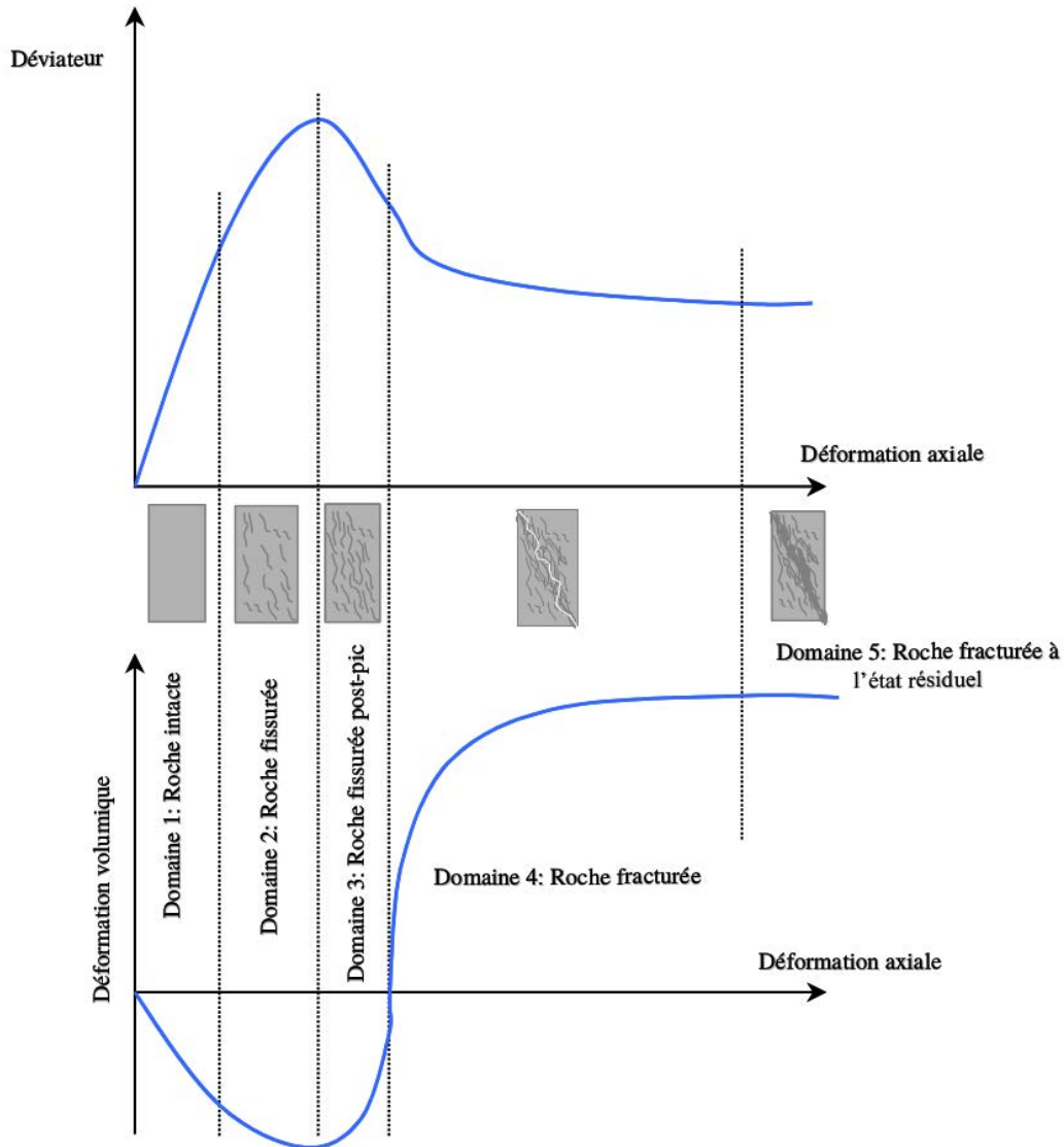
FIGURE 4.8 – Évolution du déviateur des contraintes et de la déformation volumique en fonction de la déformation axiale - [Laigle, 2004].
