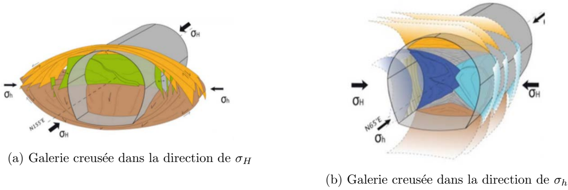
FIGURE 1.5 – Schéma des zones de fracturations induites après excavation - [Guayacan-Carrillo et al., 2017].
