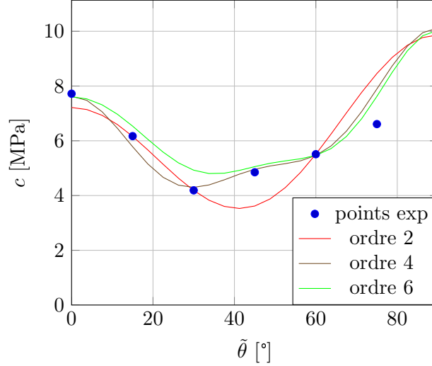
FIGURE 3.8 – Évolutions de c selon l'orientation du plan de stratification \tilde{\theta} pour l'argilite de Tournemire. Les données expérimentales proviennent de [Niandou, 1994].
