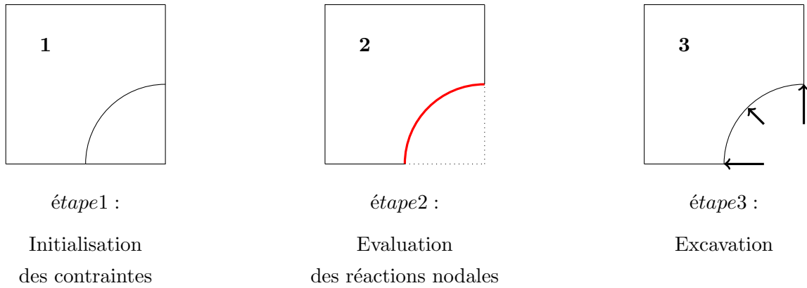
FIGURE 3.13 – Étapes du calcul numérique d'excavation.
