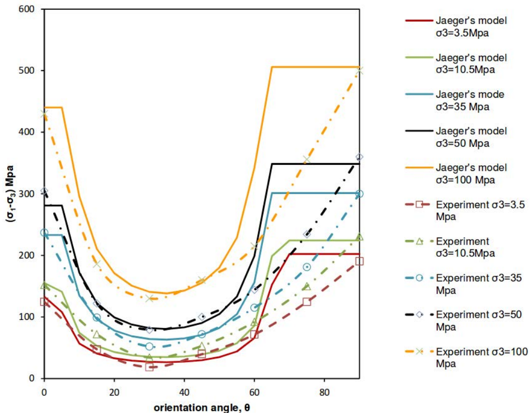
FIGURE 2.28 – Comparaison de l'évolution du seuil de résistance prédit par la théorie de Jaeger avec des résultats de laboratoire suivant l'orientation du plan de stratification - [Kassa and Nordal, 2016].
