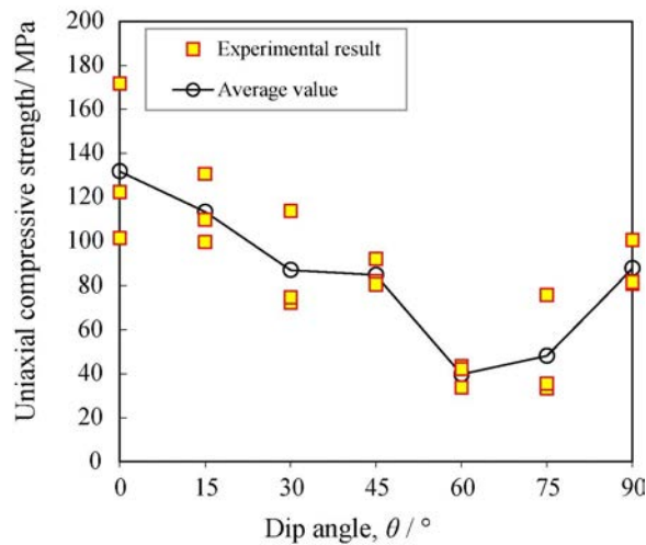
FIGURE 2.21 – Évolution de la résistance en compression simple pour les granulites (l'angle 0^\circ correspond à une éprouvette verticale) - [Wang et al., 2018].
