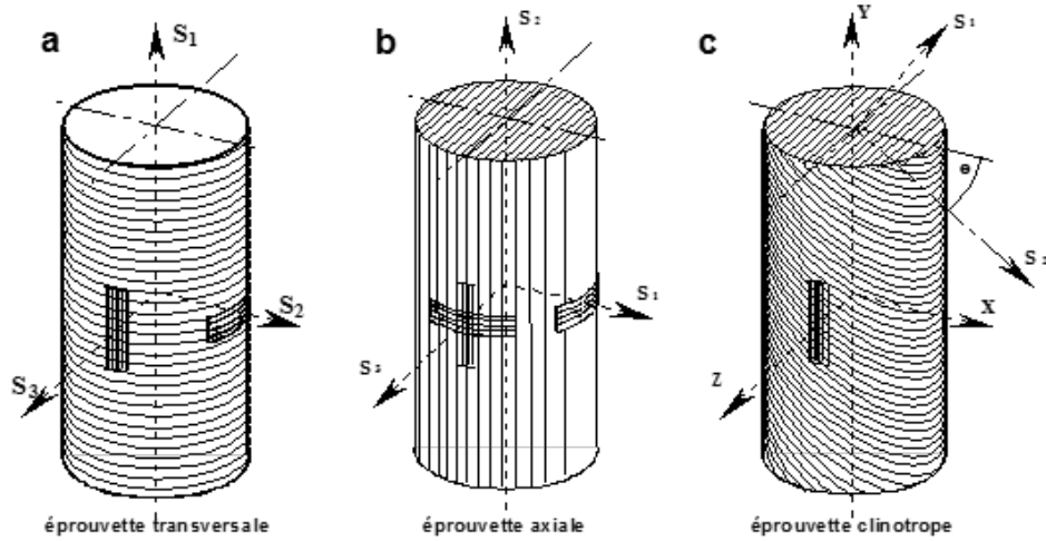
FIGURE 2.17 – Schéma d'éprouvettes orientées à 0^\circ appelée horizontale, 90^\circ appelée verticale et 45^\circ appelée clinotrope ou transverse.
