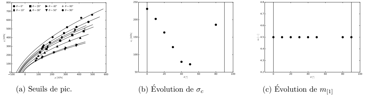
FIGURE 4.27 – Calage du paramètre \sigma_c avec m_{[1]} fixé pour l'ardoise d'Austin, pour différentes orientations.
