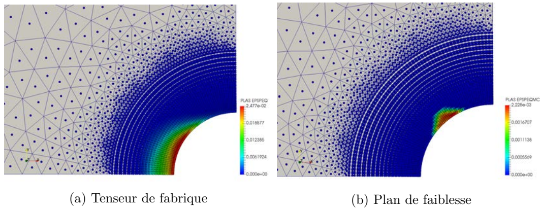
FIGURE 3.16 – Evolution de la déformation plastique.
