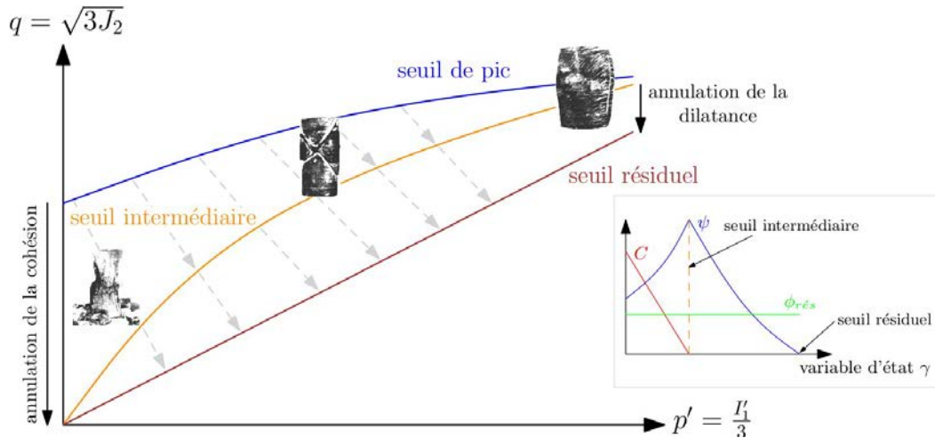
FIGURE 4.7 – Évolution des seuils pour le mécanisme élastoplastique en phase post-pic et évolution de la cohésion c , de l'angle de dilatance \psi et de l'angle de frottement \Phi_{res} - [Raude, 2015].
