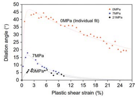
FIGURE 4.9 – Mesures et modélisation de la dilatance en fonction de la déformation pour différents confinements sur des calcaires - [Zhao and Cai, 2010].
