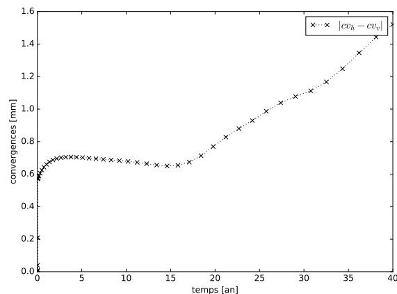
FIGURE 5.10 – Écart entre les convergences verticale et horizontale des parois, pour une galerie orientée dans la direction de la contrainte majeure \sigma_H - LKR anisotrope.
