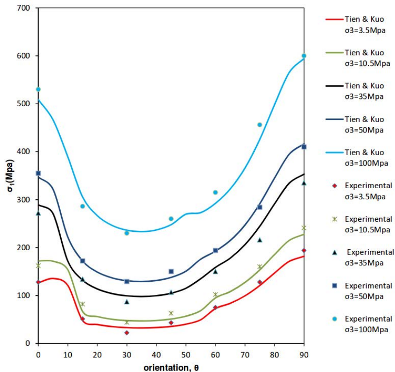
FIGURE 2.34 – Comparaison de l'évolution du seuil de résistance prédit par le critère de Tien et Kuo avec des résultats de laboratoire suivant l'orientation du plan de stratification - [Kassa and Nordal, 2016].
