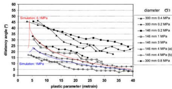
FIGURE 4.10 – Mesures et modélisation de la dilatance en fonction d'un paramètre de plasticité pour différents confinements sur des grès - [Alejano and Alonso, 2005].
