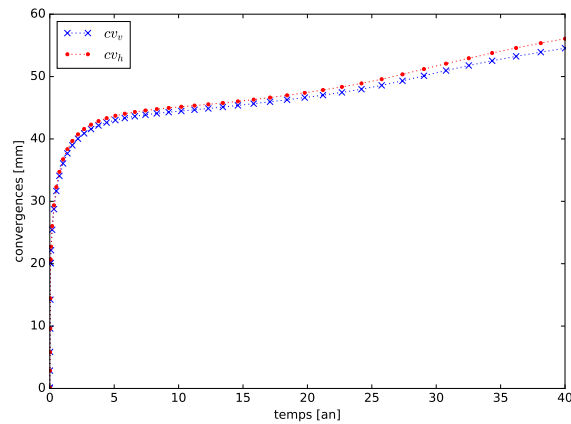
FIGURE 5.9 – Convergences verticale et horizontale des parois, pour une galerie orientée dans la direction de la contrainte majeure \sigma_H - LKR anisotrope.
