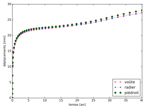
FIGURE 5.8 – Déplacements de points en parois, pour une galerie orientée dans la direction de la contrainte majeure \sigma_H - LKR anisotrope.
