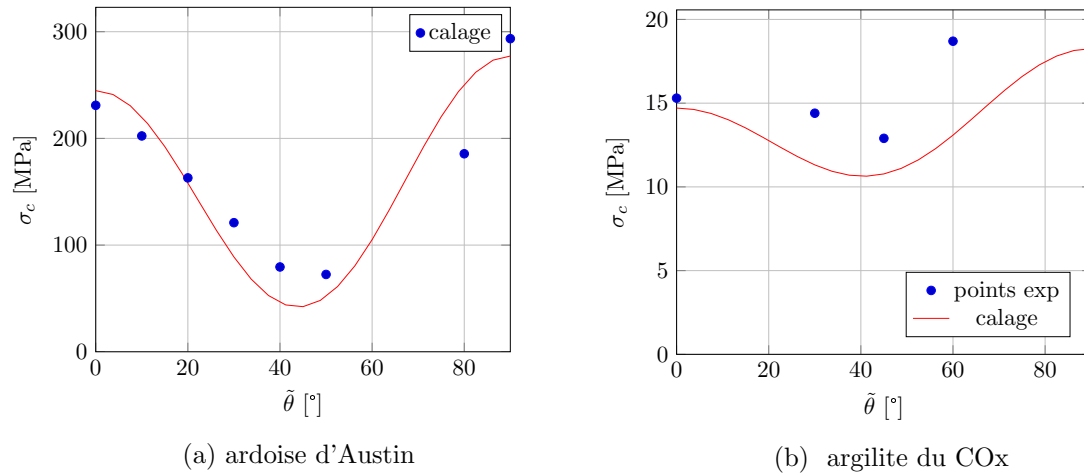
FIGURE 4.29 – Évolutions de \sigma_c selon l'orientation du plan de stratification \tilde{\theta} .
