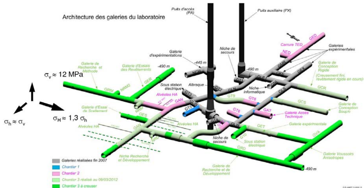
FIGURE 1.4 – Schéma des galeries du Laboratoire de Recherche Souterrain en 2012 - http://www.andra.fr .
