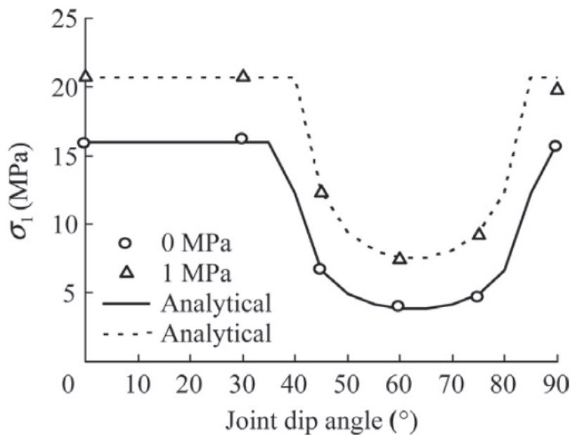
FIGURE 2.32 – Variation de la contrainte en compression uniaxiale en fonction de l’orientation du plan de faiblesse pour des confinements de 0MPa et 1MPa - [Oliveira, 2012].
