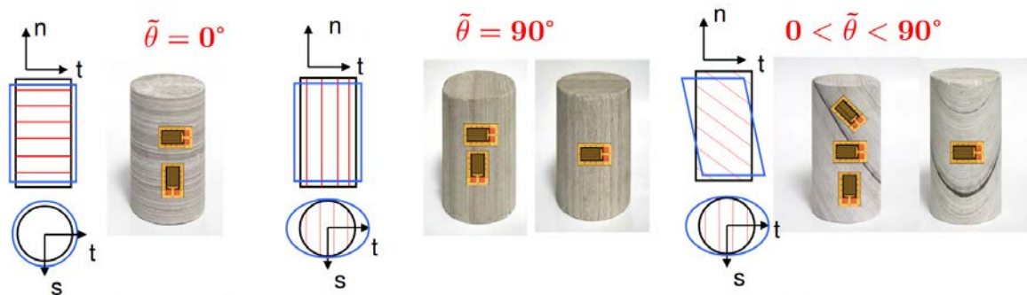
FIGURE 2.36 – Convention pour l'orientation des éprouvettes - [Pellet, 2017].
