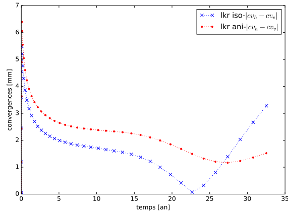
FIGURE 5.20 – Convergences verticale et horizontale des parois, pour une galerie orientée dans la direction de la contrainte majeure \sigma_h .
