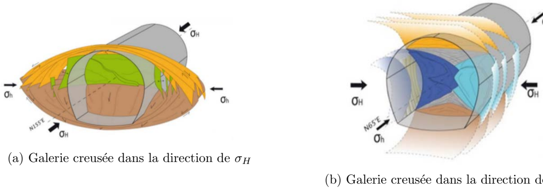
FIGURE 1.5 – Schéma des zones de fracturations induites après excavation - [Guayacan-Carrillo et al., 2017].
