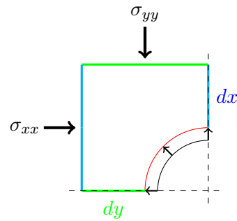
FIGURE 3.14 – Conditions limites imposées au domaine d'étude pour une excavation.
