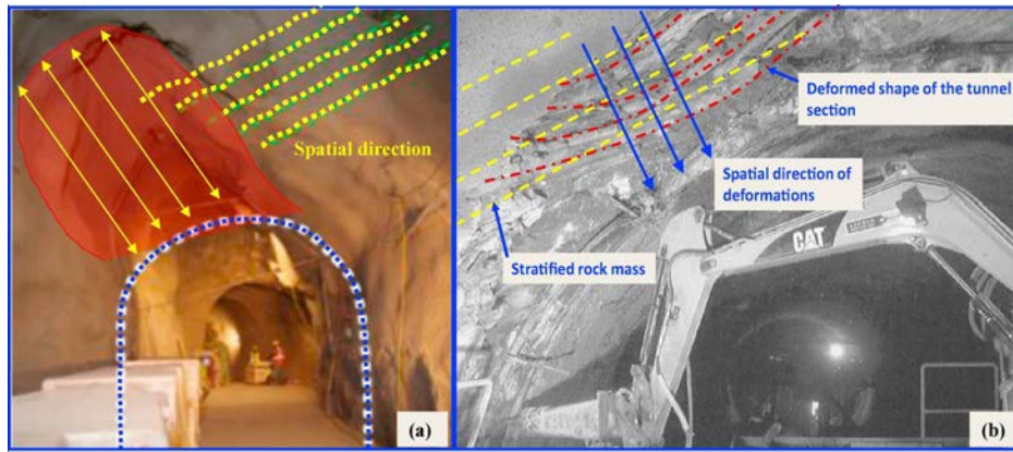
FIGURE 2.18 – Distribution spatiale de la structure géologique et des schémas de fractures correspondants, (a) site de Mont Terri [Li, 2013], (b) [Seingre et al., 2005] - [Wang et al., 2018].
