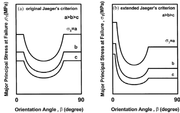
FIGURE 2.27 – Comparaison entre le critère de Jaeger initial, à gauche et le critère amélioré, à droite.
