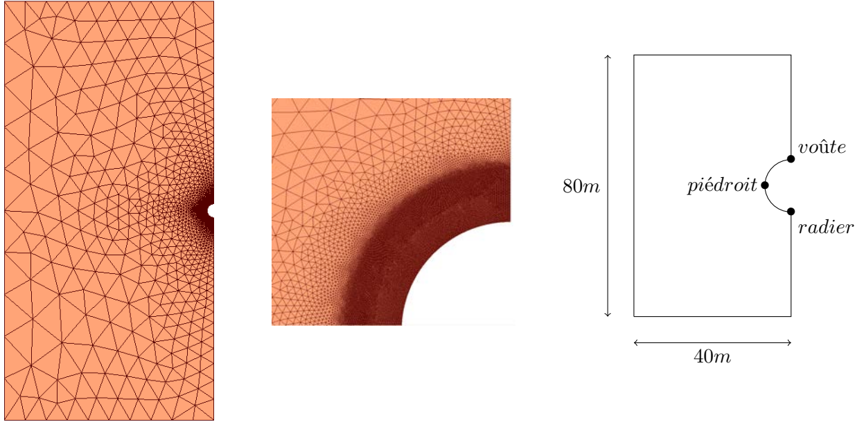
FIGURE 5.2 – Maillage pour la simulation d’excavation et géométrie de la galerie circulaire.
