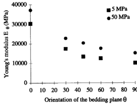
FIGURE 2.16 – Évolution du module de Young suivant l'orientation du plan de stratification pour des confinements de 5MPa et 50MPa, sur de l'argilite de Tournemire - [Niandou et al., 1997].
