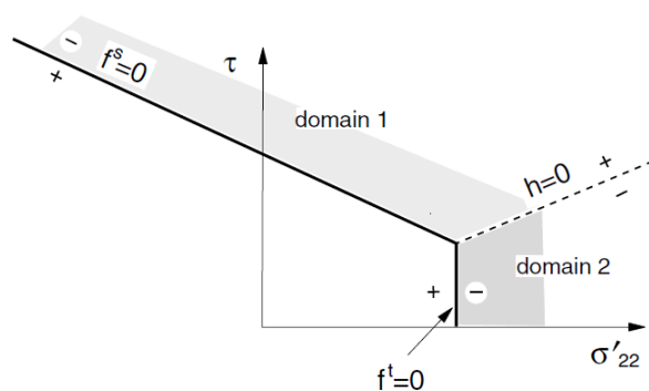
FIGURE 2.30 – Critère de rupture défini dans le plan de faiblesse.
