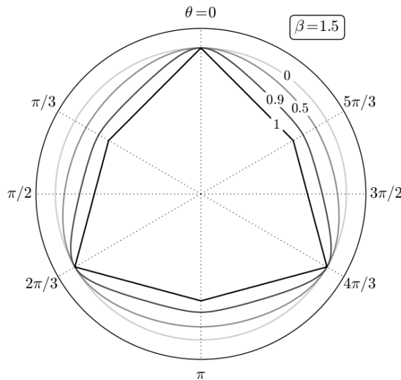
FIGURE 4.14 – Évolution du critère de plasticité dans le plan \pi pour \beta = 1.5 et \gamma \in [0, 1] - [Raude, 2015].
