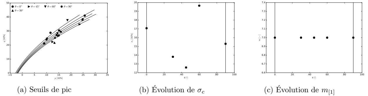
FIGURE 4.28 – Calage du paramètre \sigma_c avec m_{[1]} fixé pour l'argilite du COx, pour différentes orientations.
