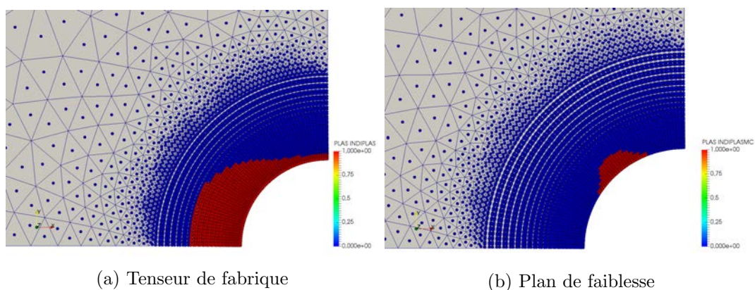
FIGURE 3.17 – Indice de plasticité.
