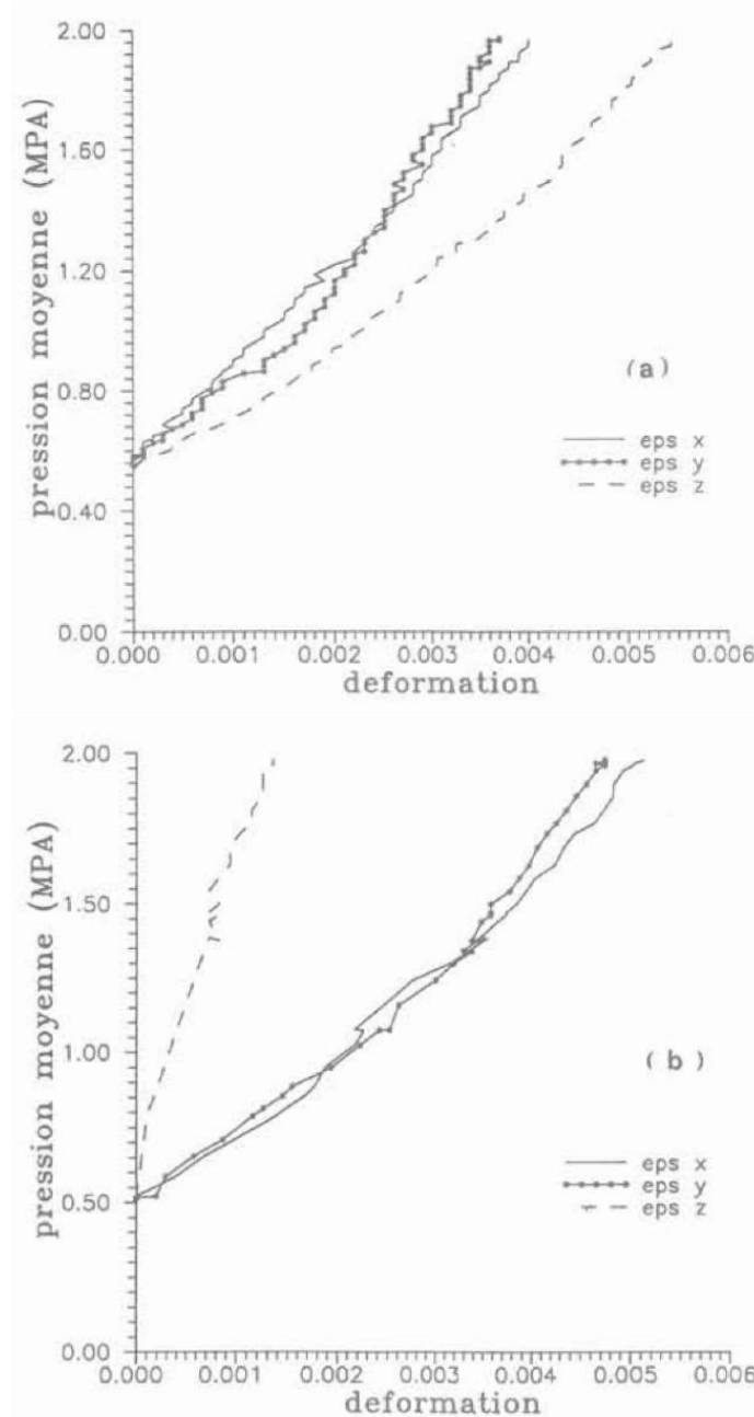
FIGURE 2.11 – Déformations \varepsilon_z , \varepsilon_x et \varepsilon_y pour un essai de compression triaxiale sur du sable dense, (a)échantillon vierge et (b)échantillon ayant subi une compression suivant la direction z - [Lanier et al., 1991].
