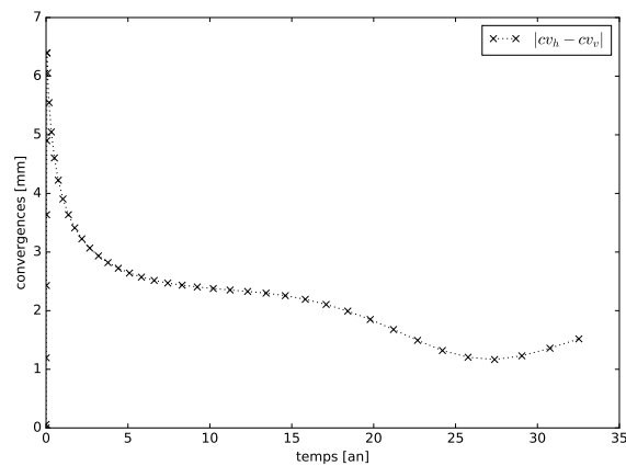
FIGURE 5.14 – Convergences verticale et horizontale des parois, pour une galerie orientée dans la direction de la contrainte mineure \sigma_h - LKR anisotrope.
