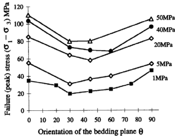
FIGURE 2.20 – Évolution de la résistance maximale à la rupture pour différentes pressions de confinement pour les argilites de Tournemire (l'angle 0^\circ correspond à une éprouvette verticale) - [Niandou et al., 1997].
