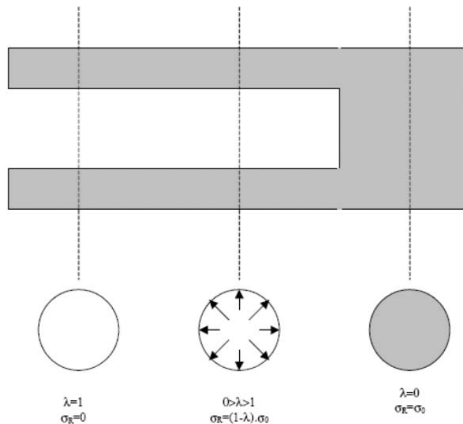
FIGURE 5.1 – Évolution du taux de déconfinement \lambda et de la contrainte radiale \sigma_r .
