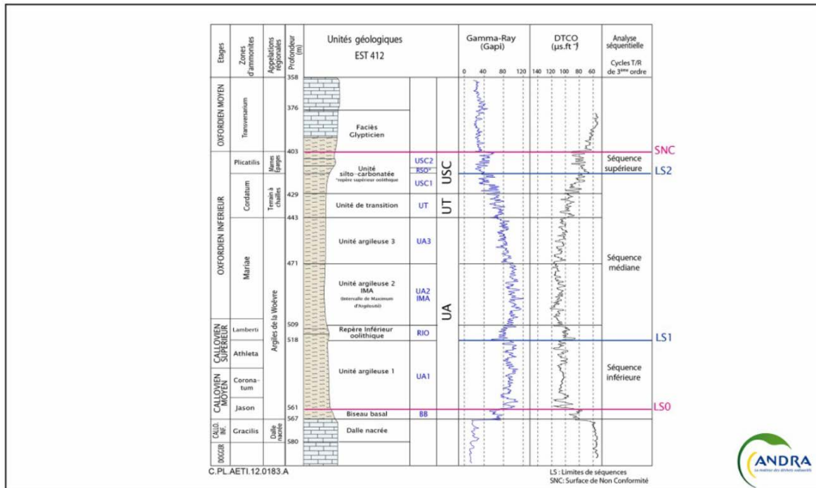
FIGURE A.3 – Principales unités géologiques du Callovo-Oxfordien : unité argileuse (UA), unité de transition (UT) et unité silto-carbonatée (USC). Les limites géologiques du Callovo-Oxfordien sont données par les surfaces LSO et SNC - [ANDRA, 2016].
