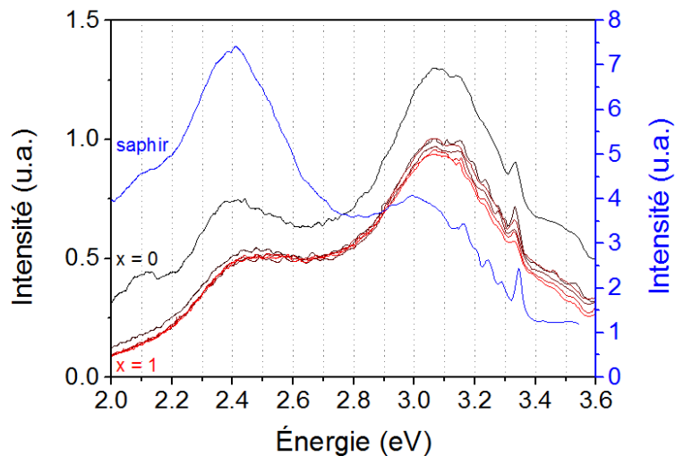
FIGURE 123 – Spectres de photoluminescence du \text{Zn}(\text{Sn},\text{Ge})\text{N}_2 et du substrat de saphir seul à 5 K.
