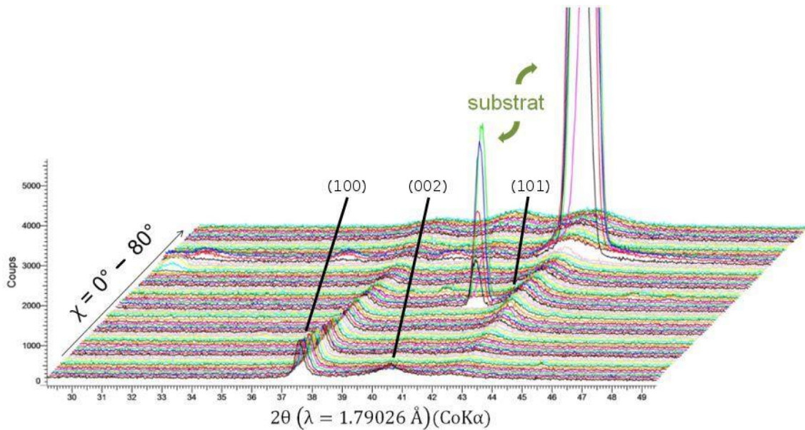
FIGURE 60 – Détexturation d'un échantillon de \text{ZnGeN}_2 sur GaN (diffractogrammes en asymétrique). Les deux pics très intenses et fins sont liés au substrat. Les pics (100), (002) et (101) appartiennent à l'échantillon de \text{ZnGeN}_2 .
