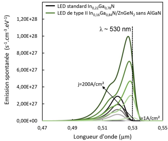
FIGURE 24 – Émissions spontanées pour une LED verte standard (en gris) et une LED de type II (en vert). Issu de [13].
