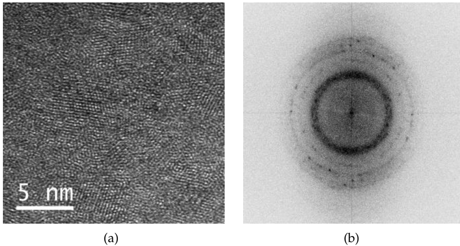
FIGURE 70 – (a) : Observation de cristallites de tailles nanométriques présentes dans la zone intermédiaire entre le substrat de GaN et les colonnes de croissance. (b) : Transformée de Fourier rapide de cette zone.
