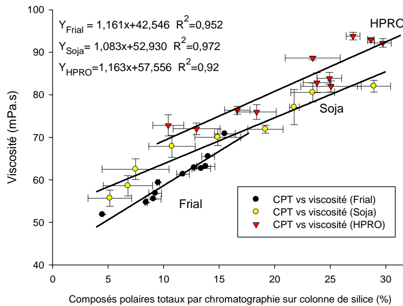
Figure 5-20 : Corrélations entre les CPT mesurés par méthode chromatographique en fonction de la viscosité des différentes huiles (Frial, soja et d'huile de palme raffinée oléine HPRO).
