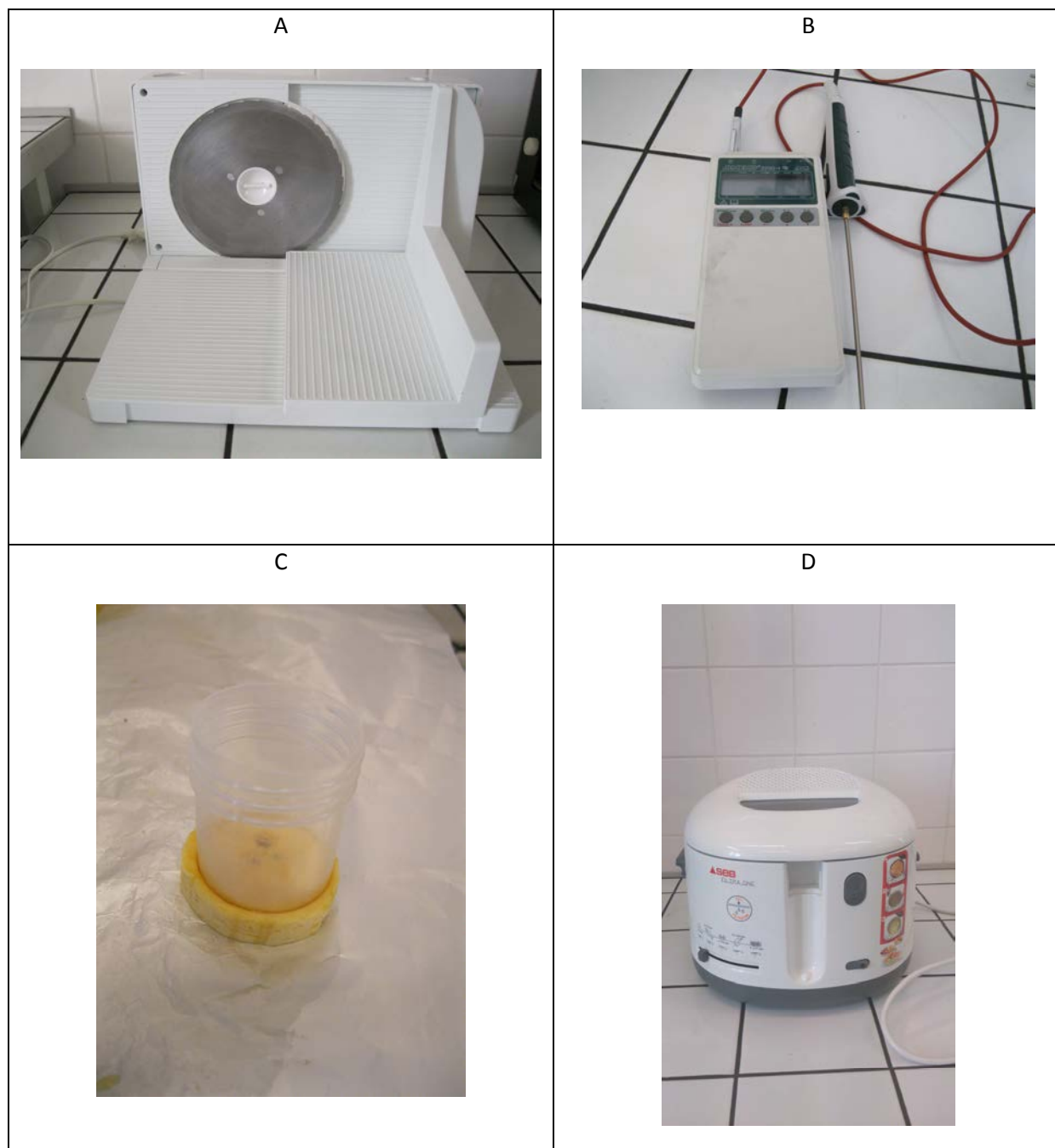
Figure 8-2 : Ensemble du matériel utilisé pour la préparation du plantain : trancheuse électrique SEB (A), enregistreur des données Almemo (B) ; emporte-pièce manuel (C) ; et friteuse ménagère électrique (D).
