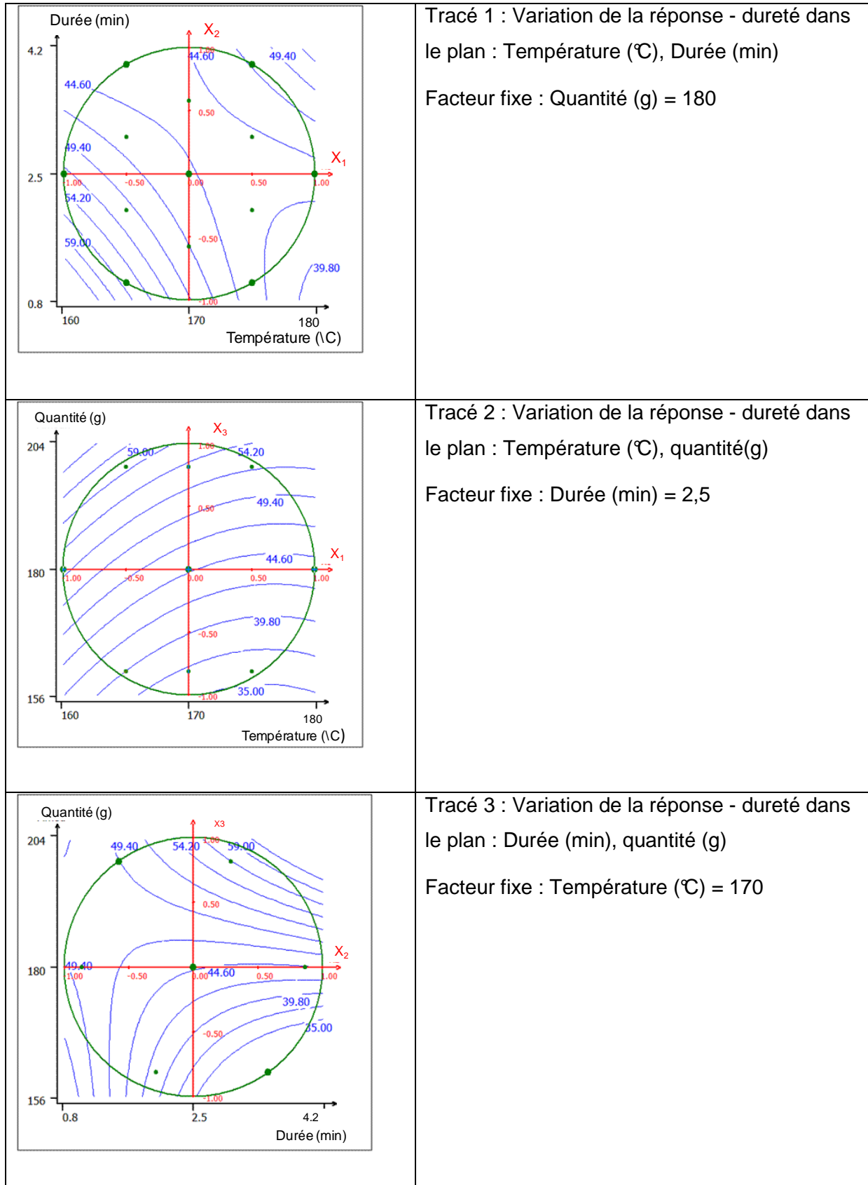
Figure 5-5 : Courbes d'isorréponses de la dureté de la banane plantain frite ( Y_3 ) dans le cas de l'huile Frial
