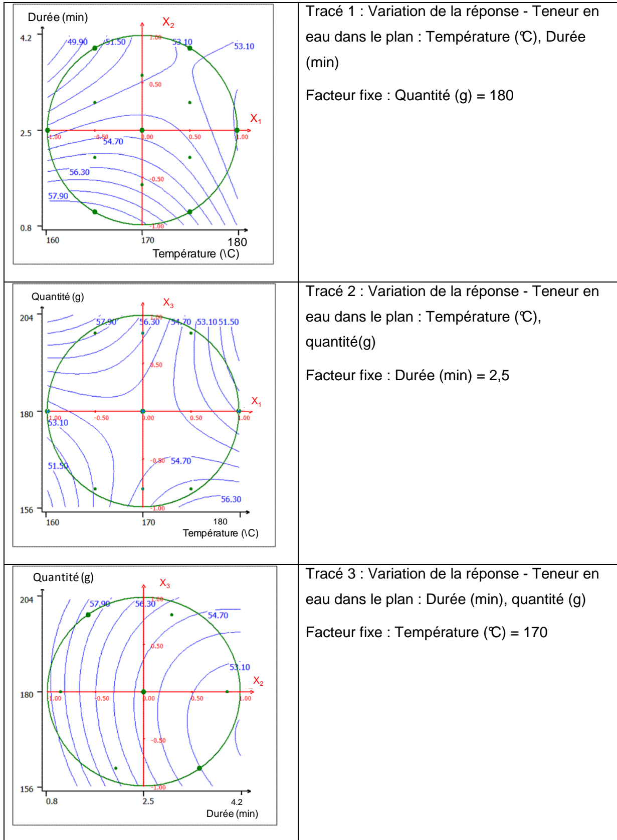
Figure 5-9 : Courbes d'isoréponses de la teneur en eau de la banane plantain frite ( Y_1 ) dans le cas de l'huile de soja.
