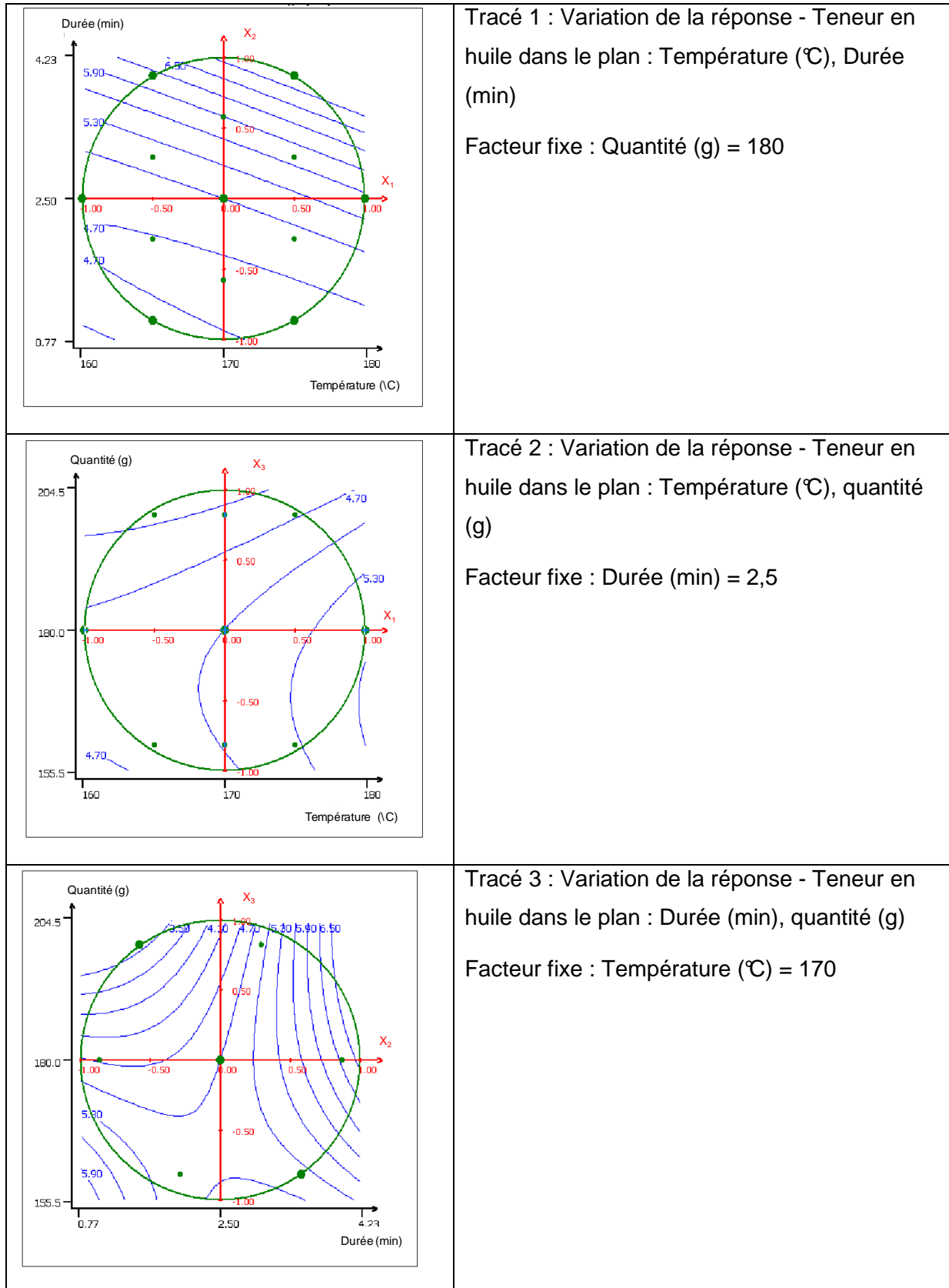
Figure 5-12 : Courbes d'isoresponses de la teneur en huile de la banane plantain frite ( Y_2 ) dans le cas de l'huile de soja
