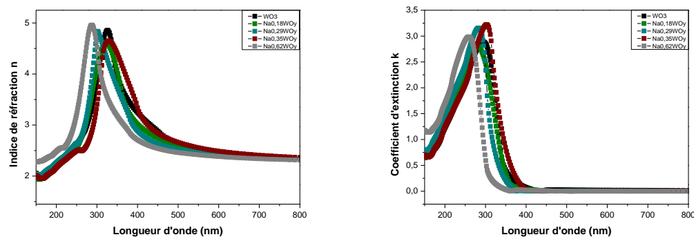
Figures A-10 : Évolution de l'indice de réfraction n (gauche) et du coefficient d'extinction k (droite) des films \text{WO}_3 et \text{Na}_x\text{WO}_y synthétisés dans l'UV-Visible et le proche infra-rouge
