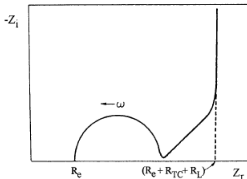
Figure A-3 : Représentation graphique d'un spectre d'impédance électrochimique dans le cas d'une électrode bloquante avec diffusion finie 133
