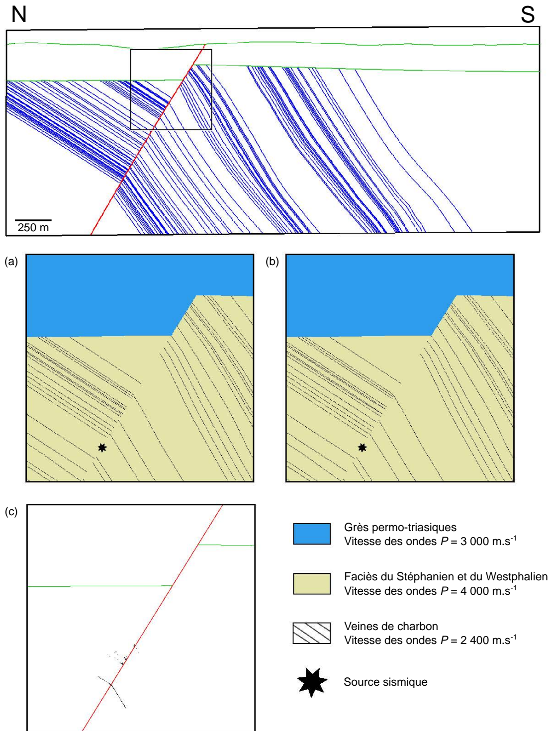
FIGURE 5.5 – MODÈLES DE VITESSES UTILISÉS POUR LA RÉALISATION DES SIMULATIONS DE PROPAGATION D’ONDES. Haut : Emplacement du sous-domaine discrétisé par la grille cartésienne et sur lequel est réalisé les simulations de propagation d’ondes. Bas : (a) Modèle de vitesse correspondant à la coupe réparée, (b) Modèle de vitesse correspondant à la coupe simplifiée, (c) Différence entre les deux modèles de vitesse (cellules noires). Modifié d’après Anquez et al. [2019].
