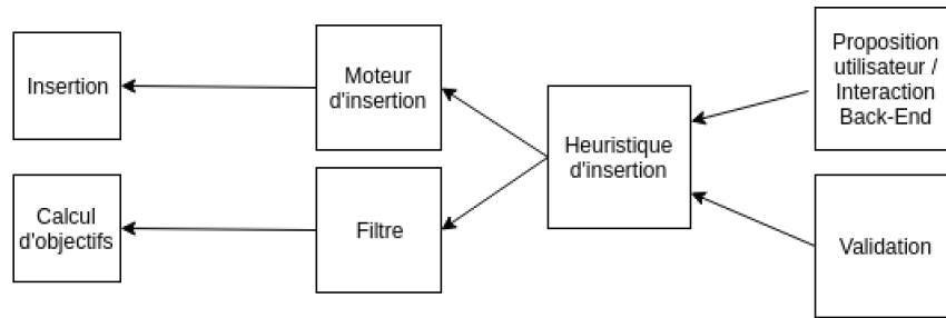
Figure 7.7 – Résumé de l’architecture globale du module online
