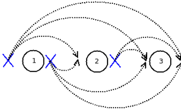
Figure 4.5 – Positions d'insertions testées sur un job avec trois noeuds
