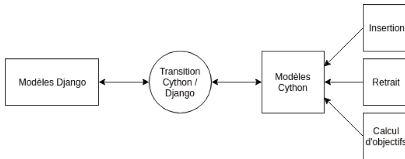
Figure 7.4 – Logique commune à tous les algorithmes
