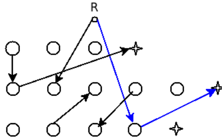
Figure 5.1 – Exemple d’un graphe avec 3 véhicules. R représente la nouvelle requête. Chaque ligne représente les sommets d’une tournée, les ronds représentant les requêtes et la croix étoilée le véhicule.
