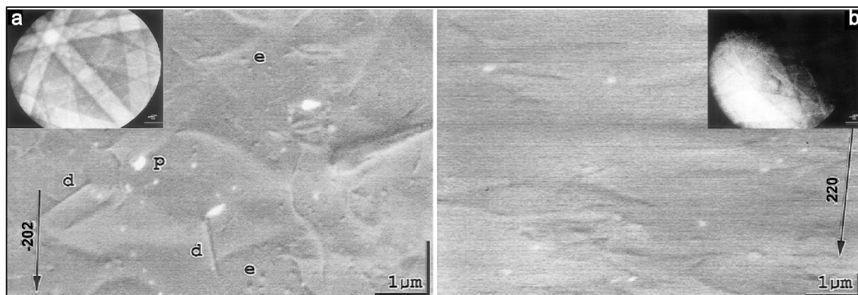
Fig.I.13. Comparaison entre les micrographies ECC et ECP acquis avec (a) la configuration à faible inclinaison et (b) la configuration à forte inclinaison [Figure d'après Simkin, 1999].
