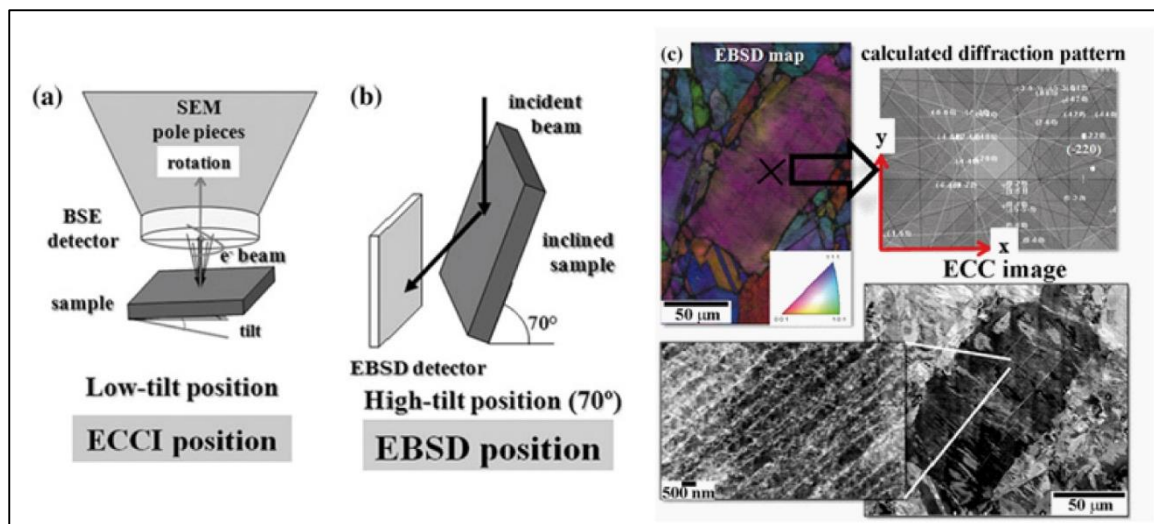
Figure III.6. Configuration géométrique de (a) l'ECCI et de (b) l'EBS. (c) Les différentes étapes pour la réalisation de la cECCI [Gutierrez-Urrutia, 2013].
