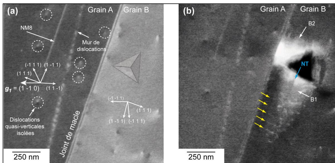
Figure.IV.19. Deuxième zone d'intérêt (Z12) formée par le grain A et le grain B dont les normales à la surface, respectives, sont [457] et [013] . (a) Micrographie ECC acquise pour la diffraction \mathbf{g}_1=(1-10) comportant la position de l'empreinte Berkovich. Les flèches blanches situent les normales des plans \{111\} . (b) Micrographie BSE montrant les deux bourrelets autour de l'empreinte. La flèche bleue pointe vers une NM et les jaunes vers les dislocations.
