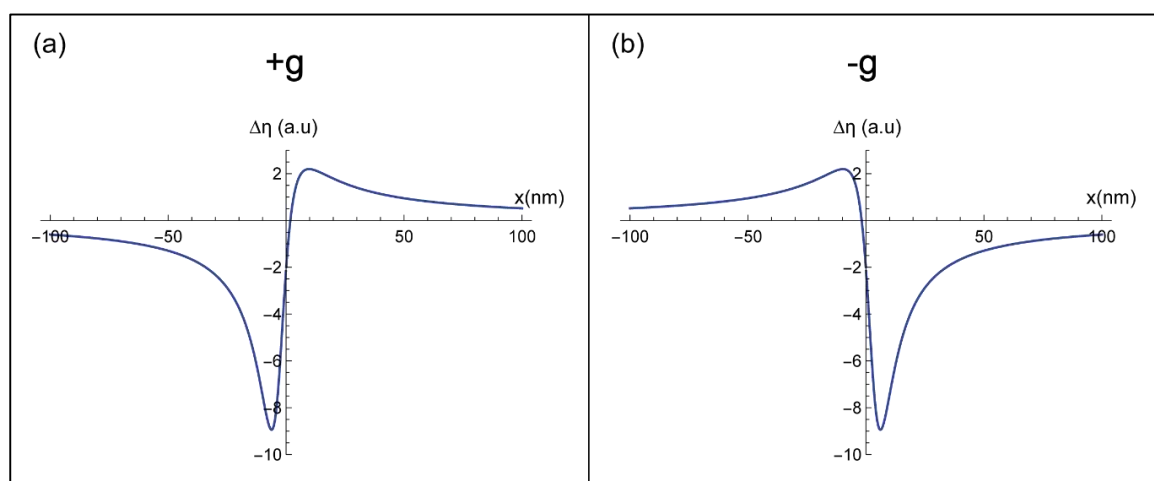
Figure.III.22. Profils d'intensité BSE modélisés au voisinage de la dislocation vis avec s < 0 pour la diffraction (a) +g et (b) -g .
