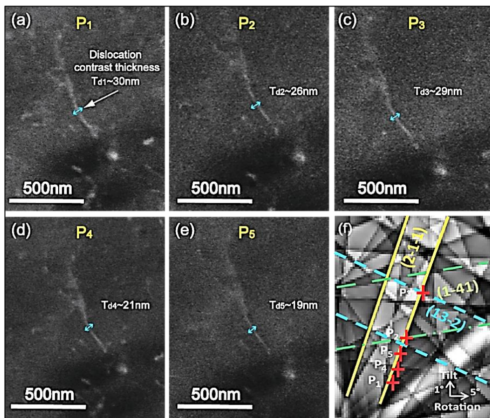
Figure.III.15. (a-e) Micrographies ECC de la même dislocation observée sous la même condition de diffraction \mathbf{g} = (2-1-1) et s > 0 . (f) Pseudo-diagramme de Kikuchi simulé à 0^\circ sur lequel sont indiquées les différentes positions du faisceau incident P_i . Les lignes vertes et bleues repèrent, respectivement, les bandes (1-41) et (13-2).
