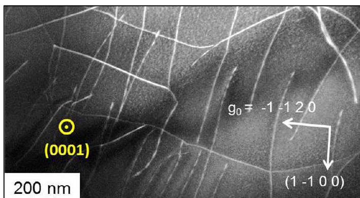
Figure.I.6. Micrographie MET des dislocations observées, en mode faisceau faible, dans un échantillon \text{Ti}_2\text{AlN} déformé [Guitton, 2014].
