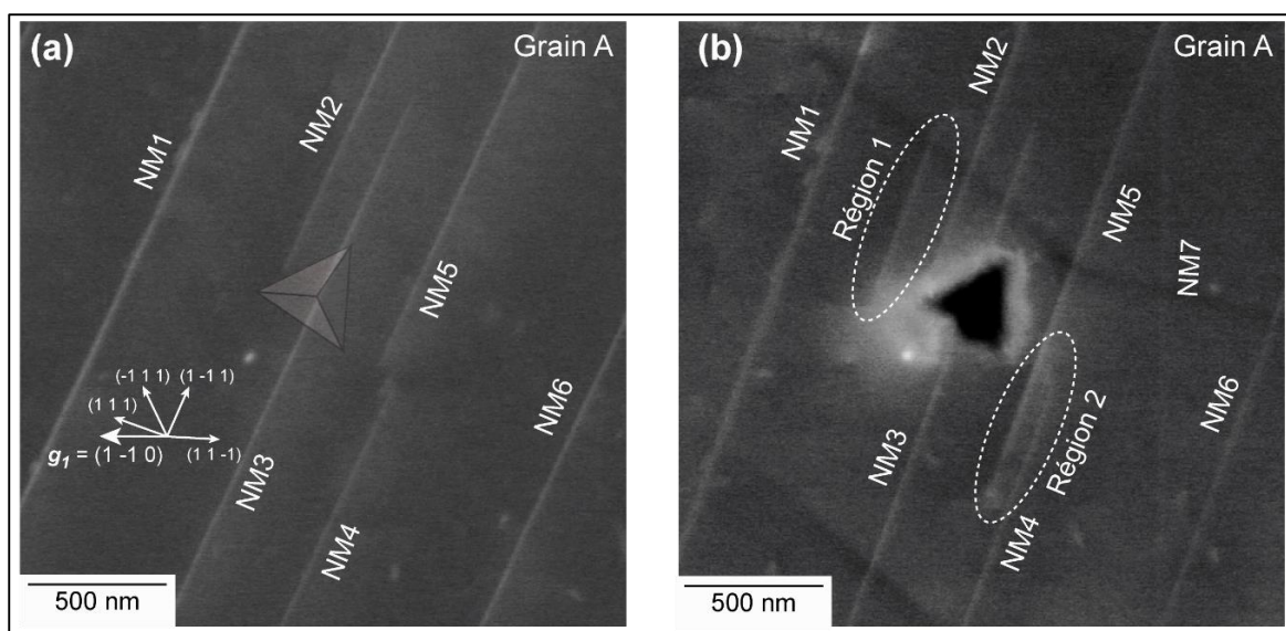
Figure.IV.18. Première zone d'intérêt (ZI1) dont la normale à la surface est proche de [457] . (a) Micrographie ECC acquise, avant déformation, pour la diffraction \mathbf{g}_1=(1-10) montrant 6 nano-macles (NM) [11-2] (111) et la position de l'empreinte (une empreinte Berkovich transparente). Les flèches blanches situent les normales des plans \{111\} . (b) Micrographie BSE montrant l'indentation de charge 500 \mu\text{N} et les deux régions nommées région 1 et région 2.
