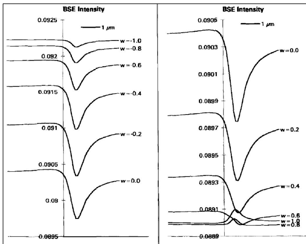
Figure.I.18. Effet de la déviation par rapport à la position de Bragg sur les profils d'intensité BSE calculés pour des dislocations vis [Wilkinson, 1993].
