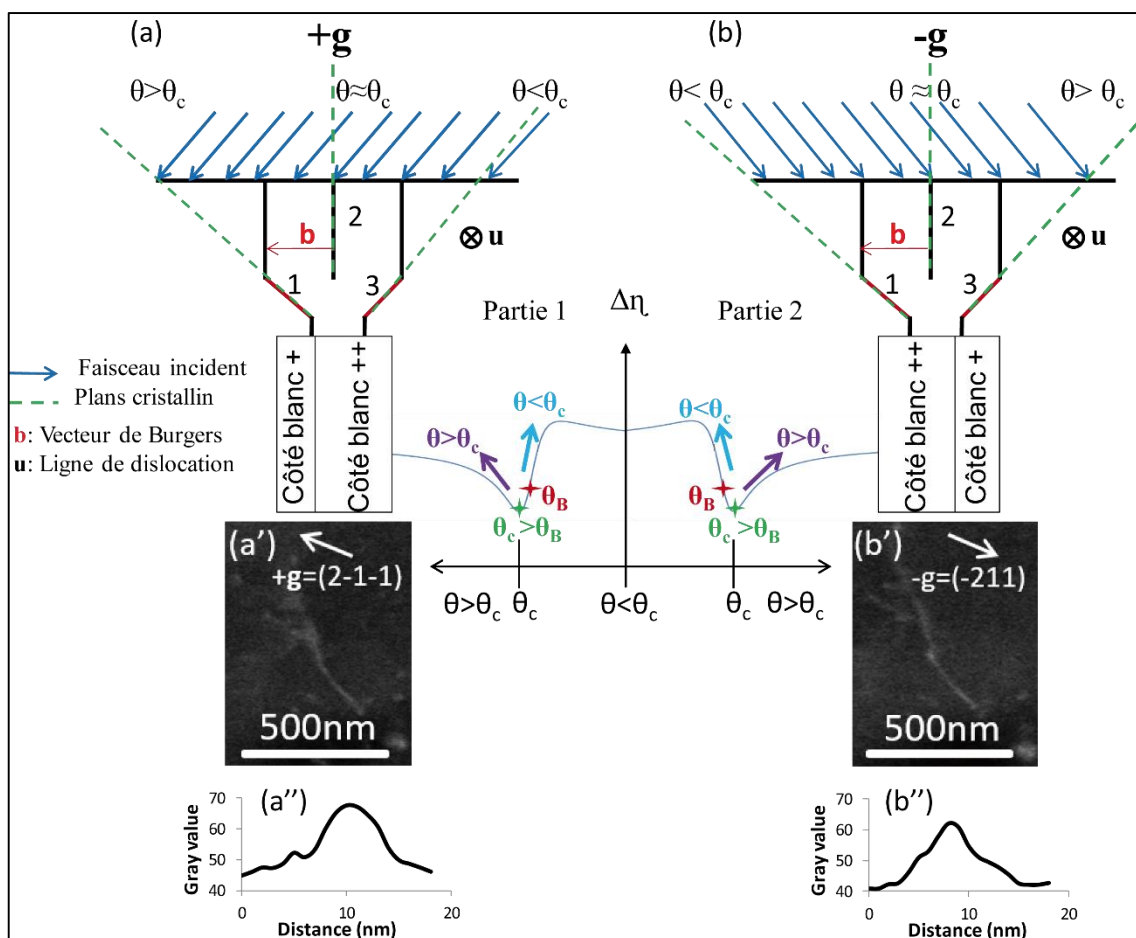
Figure.III.19. Présentations schématiques d'une dislocation en condition de diffraction s>0 avec (a) +\mathbf{g}=(2-1-1) et (b) -\mathbf{g}=(-211) . Les micrographies ECC, de la même dislocation, et leurs profils d'intensité correspondants sont présentés, respectivement, par (a') (b') et (a'') (b''). La courbe théorique ( \Delta\eta=f(\theta) ) décrit la modulation de l'intensité BSE en fonction de l'angle d'incidence.
