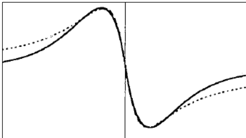
Figure.I.19. Profils d'intensité calculés pour une dislocation coin située à une profondeur 0,2\xi_g sous la surface. La courbe en pointillés ne met en évidence que les effets de la déformation locale des plans cristallins sur le contraste d'intensité BSE. La courbe en trait plein tient compte à la fois des effets de la déformation locale et de ceux de la relaxation des contraintes surfaciques sur le contraste [Wilkinson, 1995].
