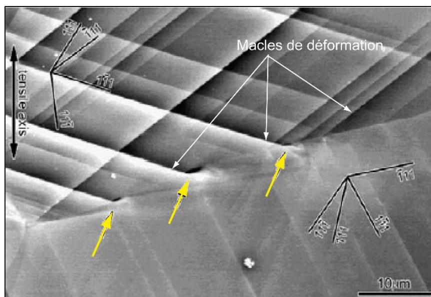
Figure.IV.11. Micrographie BSE d'un joint entre deux grains \gamma . Les flèches jaunes pointent vers les microfissures [Simkin, 2003].
