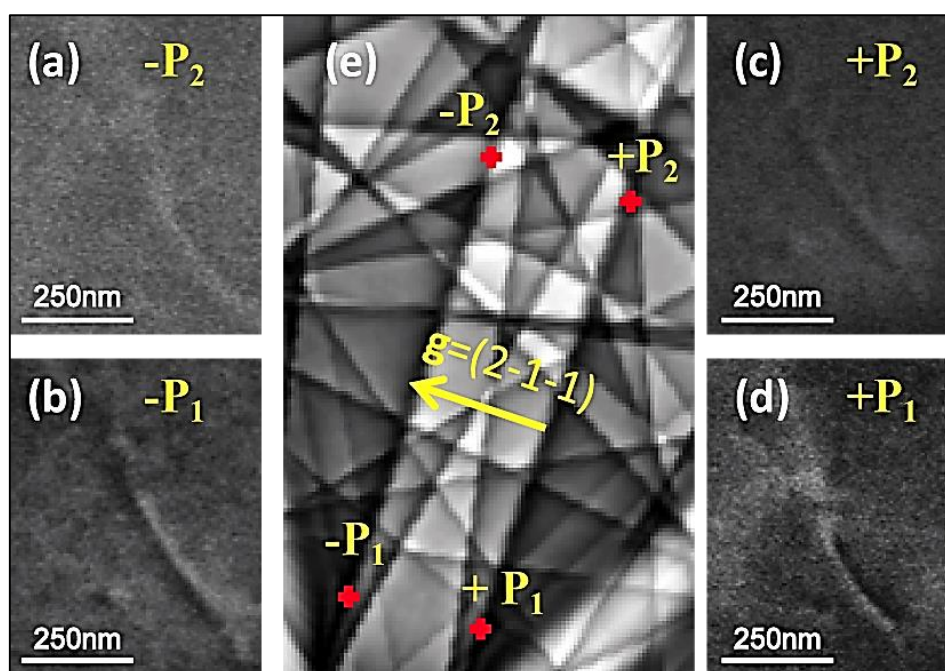
Figure.III.16. (a-d) Micrographies ECC de la même dislocation observée avec g=(2-1-1) et s=0 .(e) Les différentes positions \pm P_1 et \pm P_2 du faisceau incident sont indiquées par des croix rouges sur le pseudo-diagramme de Kikuchi.
