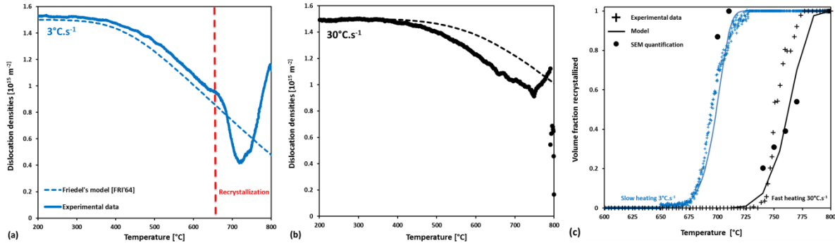
Figure 5 : Evolution mesurée (trait plein) et calculée (trait pointillé) de la densité de dislocations en fonction de la température lors de la chauffe (a) à 3^\circ\text{C.s}^{-1} en bleu et (b) à 30^\circ\text{C.s}^{-1} en noir respectivement. (c) Evolution de la fraction recristallisée en fonction de la température pour les deux vitesses de chauffage avec le même code couleur que précédemment. Les croix correspondent aux mesures in situ par HEXRD, les points à des mesures en MEB et les traits continus au modèle développé dans ces travaux.
