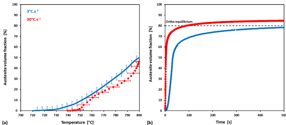
Figure 6 : Mesures in situ réalisés par DRXHE du volume d'austénite transformé (a) en fonction de la température et (b) du temps pour deux vitesses de chauffage (chauffage à 800^\circ\text{C} à vitesse constante puis maintien à 800^\circ\text{C} pendant 600s).
