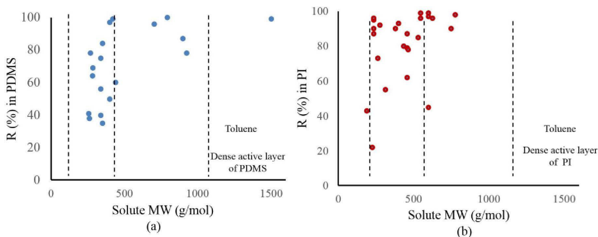
Figure 4: Performance de rejet de la membrane OSN en fonction du masse moléculaire (MW) du toluène: (a) PDMS (b) PI.
