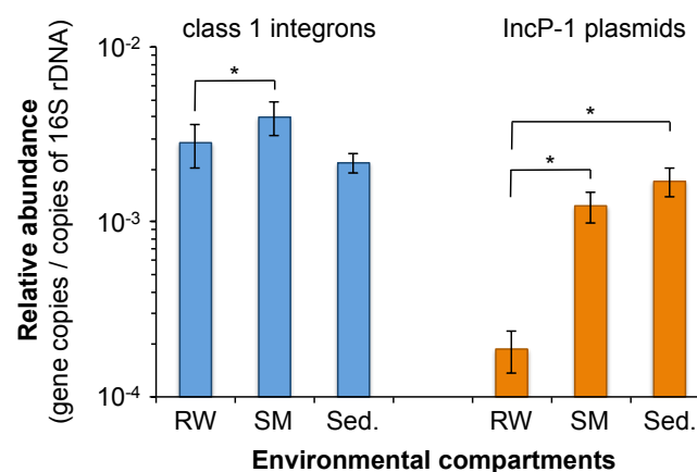
Figure 12 : Abondances relatives des intégrons de classe 1 et des plasmides IncP-1 dans les compartiments physiques de la rivière Orne (De la Cruz Barrón et al., 2018).
