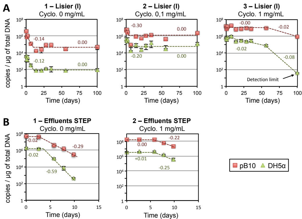
Figure 4 : Suivi du transfert de pB10 en matrices environnementales (adapté de Bellanger et al, 2014a).
