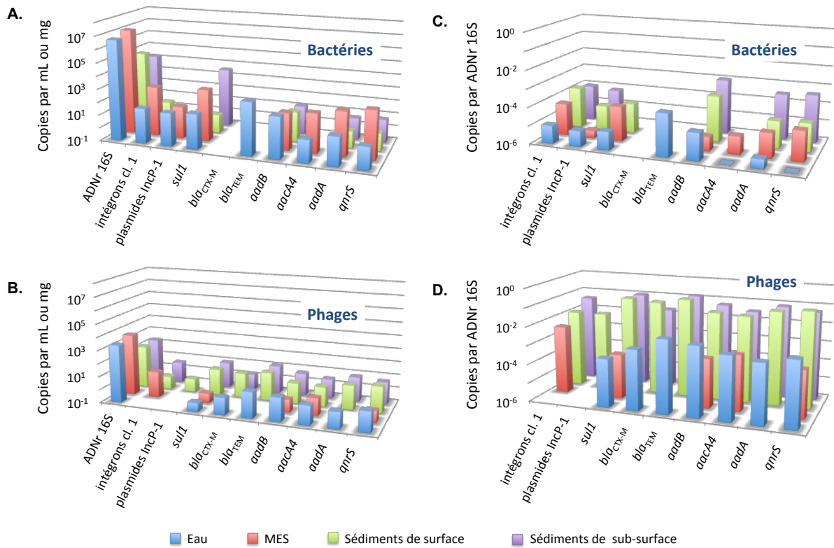
Figure 17 : Abondances absolues et relatives en différents marqueurs moléculaires bactériens indicateurs d'antibiorésistance dans les compartiments physiques de la rivière Orne.
