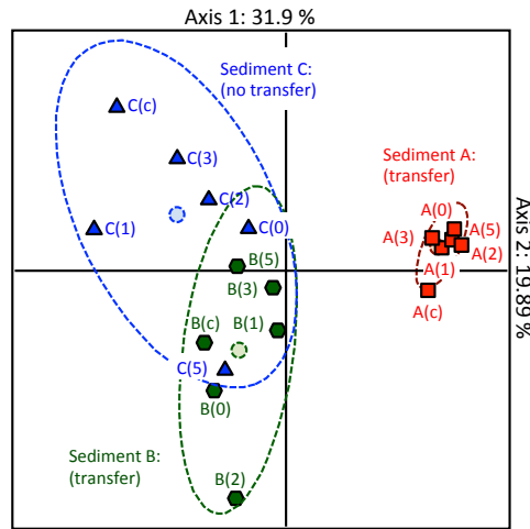
Figure 5 : Tentative de mise en lumière du caractère permissif de diverses communautés microbiennes environnementales vis-à-vis du transfert de pB10 par TTGE (adapté de Bellanger et al, 2014b).
