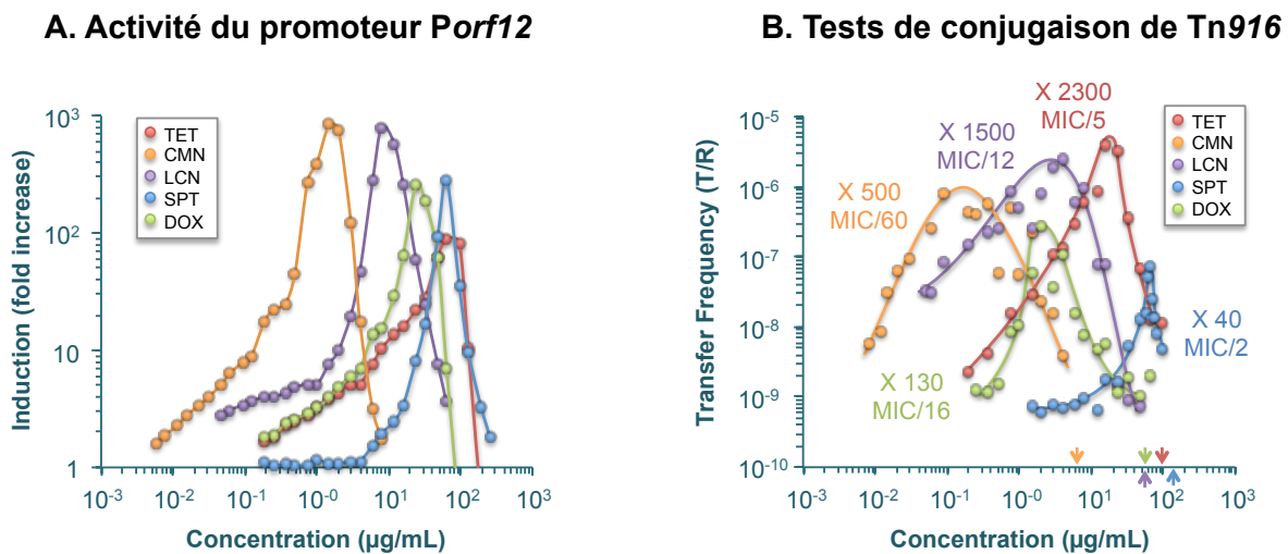
Figure 10 : Effet d'antibiotiques en doses sub-inhibitrices sur l'activité du régulateur central de Tn916, orf12 , et son transfert conjugatif (d'après Scornec et al., 2017).
