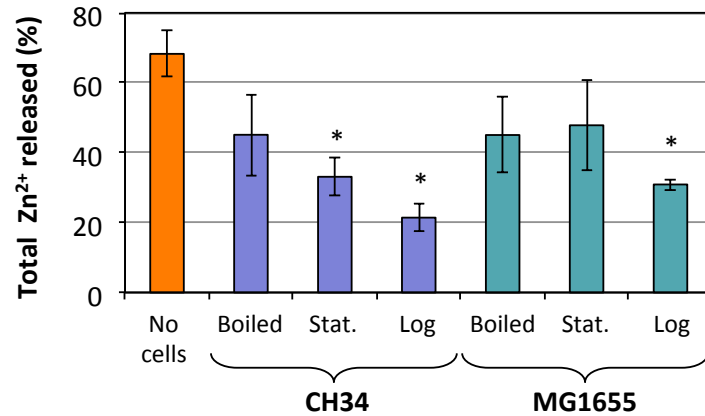
Figure 7 : Quantification du Zn 2+ libéré par des quantum dots d'oxyde de zinc co-incubés 24h dans un dispositif de dialyse avec des cellules bactériennes (adapté de Bellanger et al, 2015).
