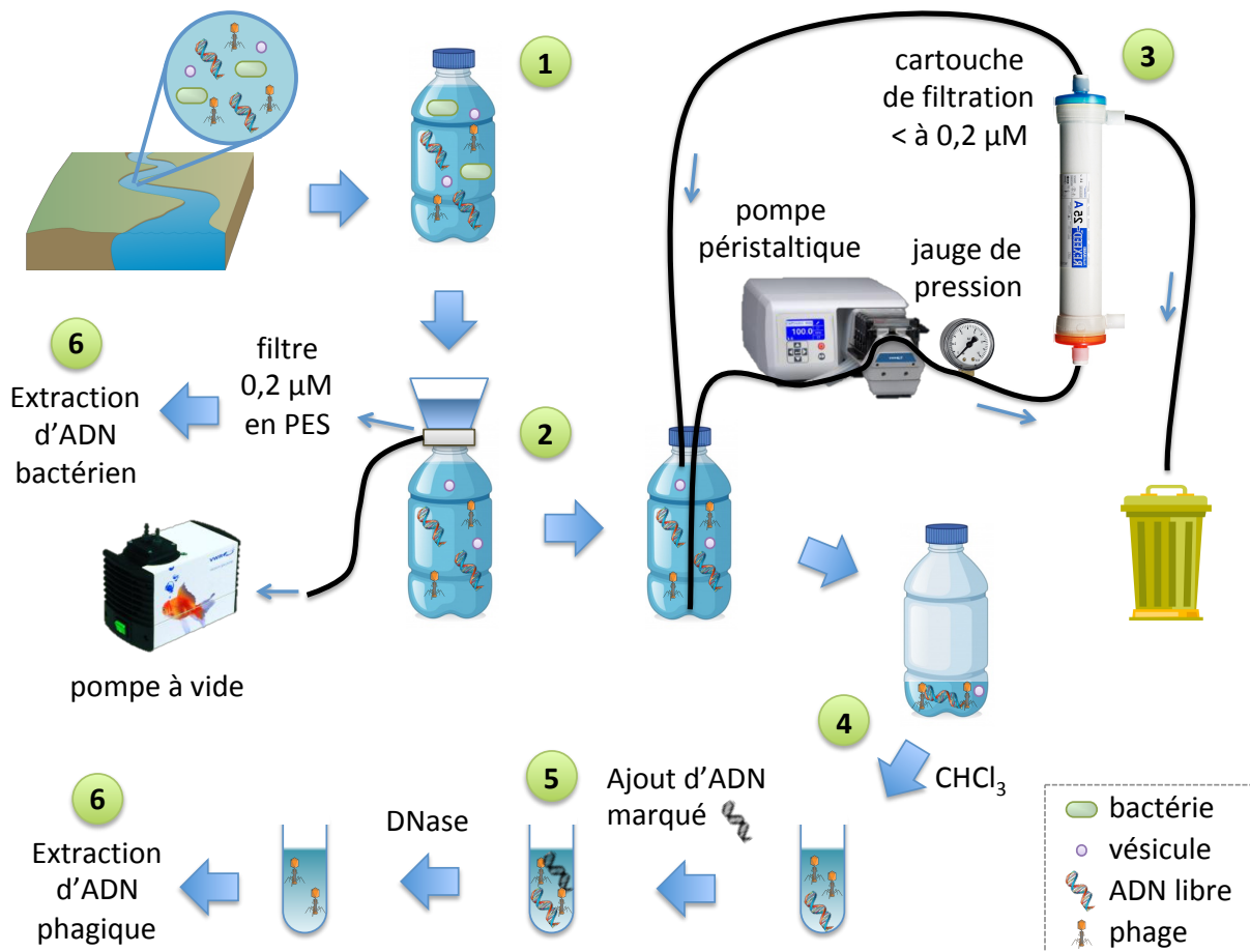
Figure 16 : Schématisation du protocole d'extraction d'ADN phagique environnemental développé.
