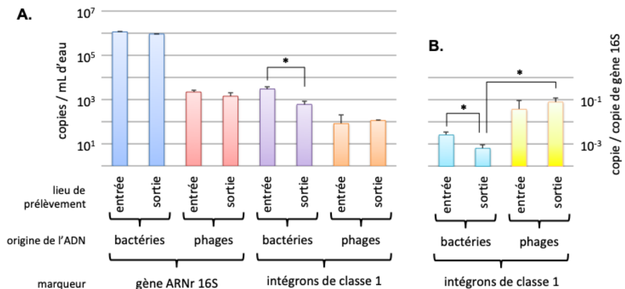
Figure 18 : Abondances absolues (A.) et relatives (B.) en gènes codant l'ARNr 16S et l'intégrase des intégrons de classe 1 ( int1 ) dans l'eau d'une zone humide en aval de la station d'épuration du Grand Reims.
