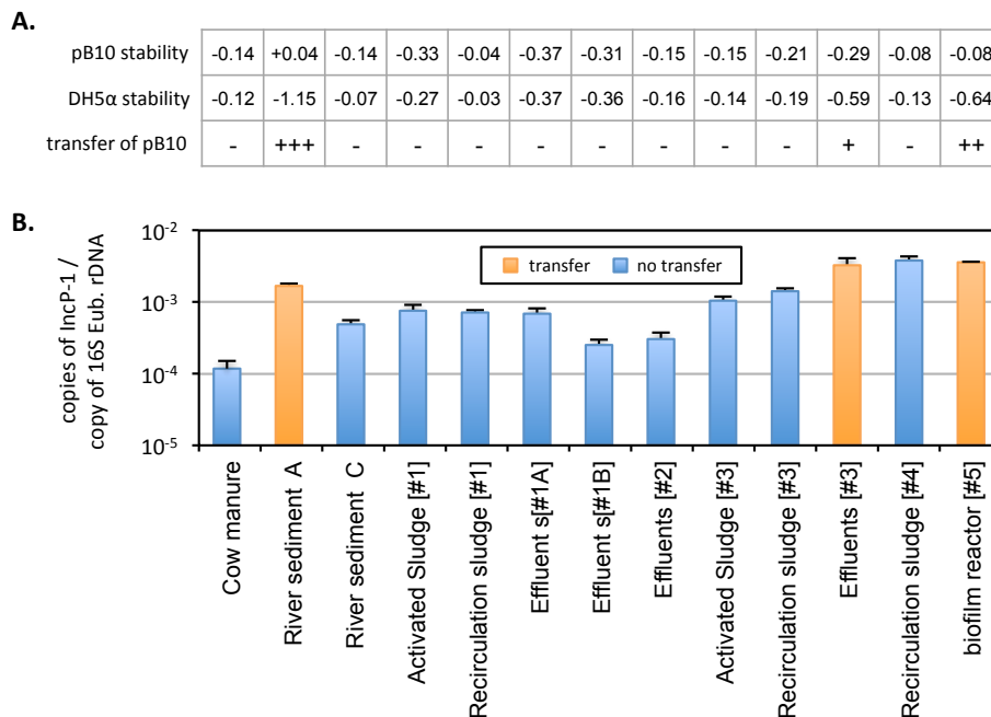
Figure 6 : Mise en lumière du caractère permissif de diverses communautés microbiennes environnementales vis-à-vis du transfert de pB10 par analyse de l'abondance relative en plasmides IncP-1 (adapté de Bellanger et al, 2014b).
