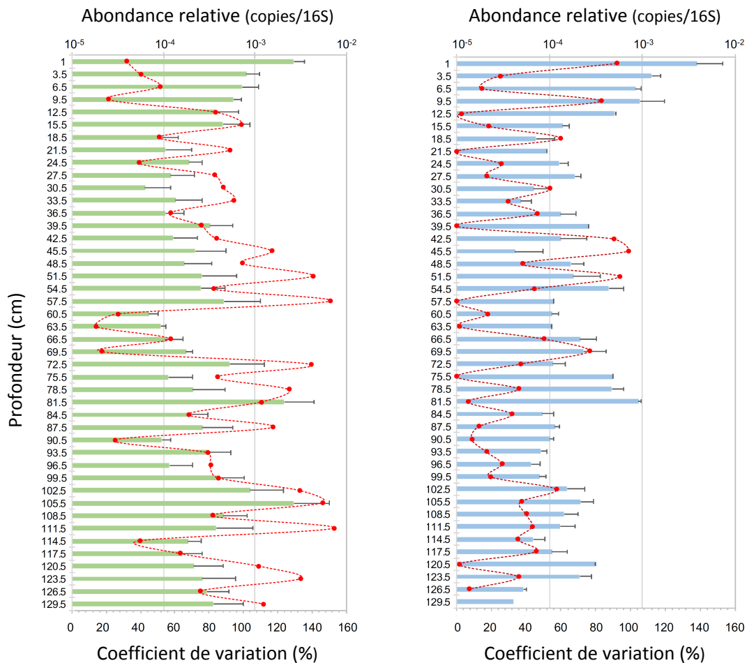
Figure 13 : Abondances relatives des intégrons de classe 1 dans la carotte de sédiments prélevée à BETH (De la Cruz Barrón, 2018).
