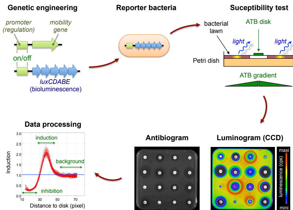
Figure 9 : Stratégie expérimentale d'étude de l'effet des antibiotiques en doses sub-inhibitrices sur des promoteurs d'éléments génétiques mobiles.
