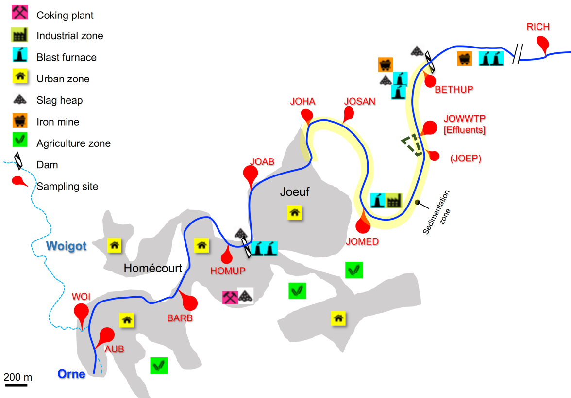
Figure 11 : Présentation de la section de la rivière Orne étudiée dans le cadre du projet « MobiSed » et de la thèse de Magali de la Cruz Barrón (2015-2018) (De la Cruz Barrón, 2018; Kanbar et al., 2017).
