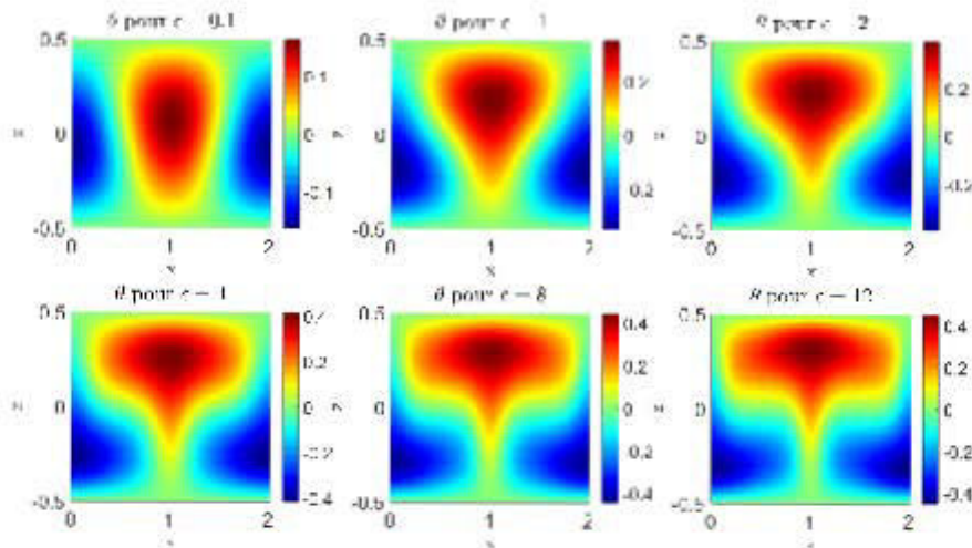
FIGURE 3.12 – Champs de température \theta pour un fluide Newtonien
