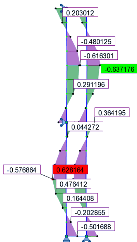
Fig. IX.57. Moment fléchissant au 2 nd ordre de l'échafaudage de façade 8 m x 0,7 m avec les I.I. déterminées selon la méthode (e)
