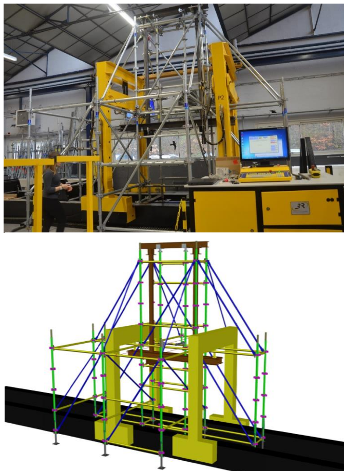
Fig. IV.14. Dispositif d'essai en vraie grandeur pour les essais sur les échelles d'échafaudage
