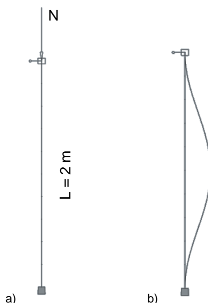
Fig. V.3. a) Barre bi-encastée sous un effort de compression ; b) Déformée critique de la barre
