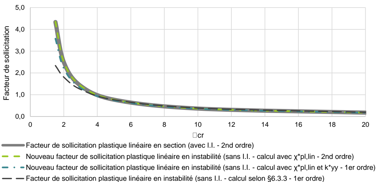
Fig. VI.41. Résultats de l'étude comparative des nouveaux critères de vérification plastique linéaire en instabilité pour la barre bi-encastée comprimée fléchie avec chargement transversal concentré
