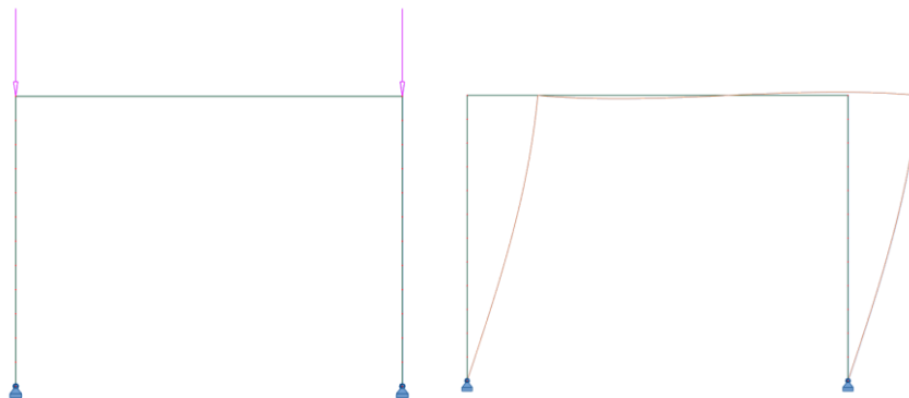
Fig. III.5. a. Portique bi-articulé sollicité par deux charges de compression ; b. Déformée critique du premier mode de flambement du portique
