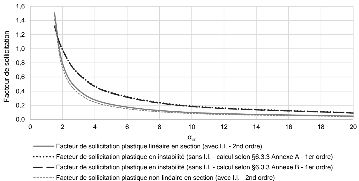
Fig. V.33. Résultats de l'étude comparative des critères de vérification en plasticité pour le portique bi-articulé comprimé fléchi
