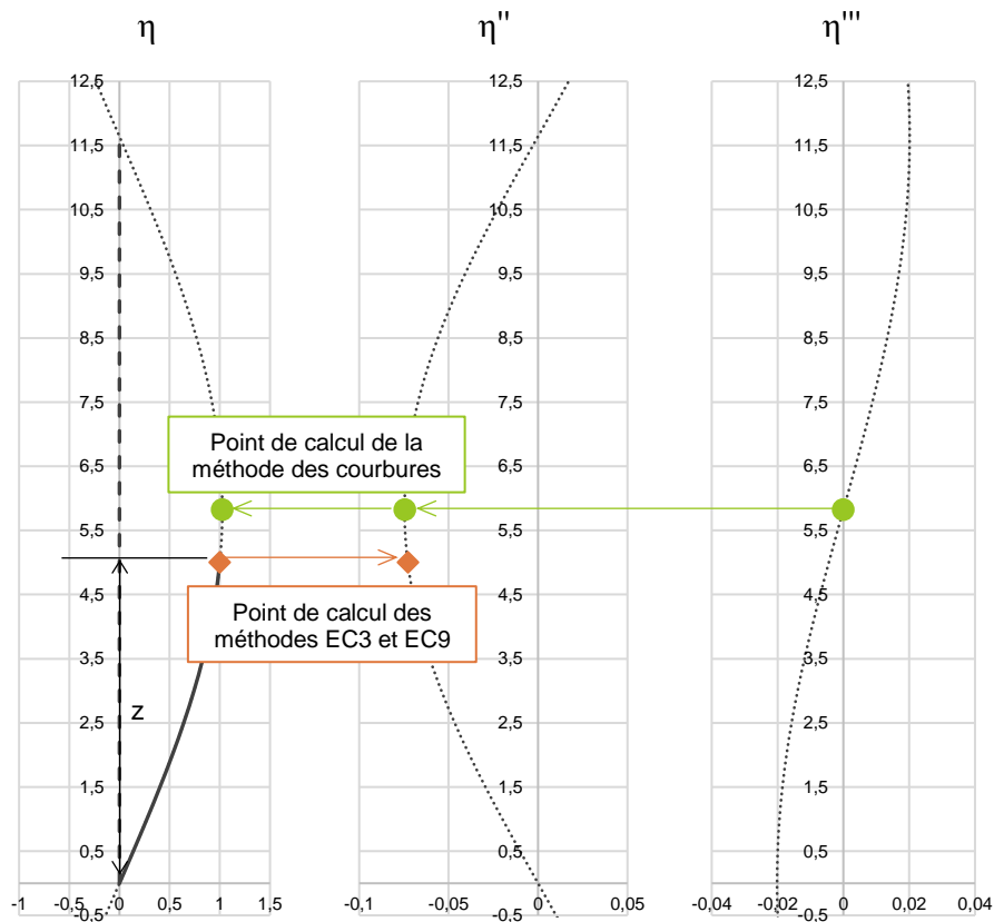
Fig. IX.26. Barre virtuelle du poteau gauche du portique bi-articulé 5 m x 5 m déterminée à partir de la méthode des courbures
