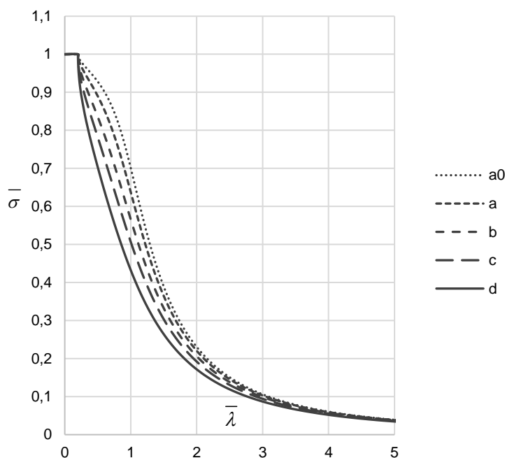
Fig. II.10. Courbes européennes de flambement
