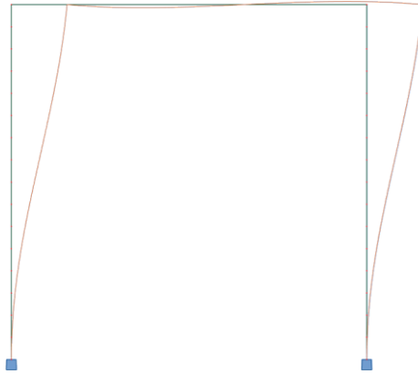
Fig. IX.9. Déformée critique du 1 er mode de flambement du portique bi-encastéré 4 m x 4 m
