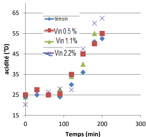
Figure 62. Variation de l'acidité pour les échantillons de vin au cours de la fermentation
