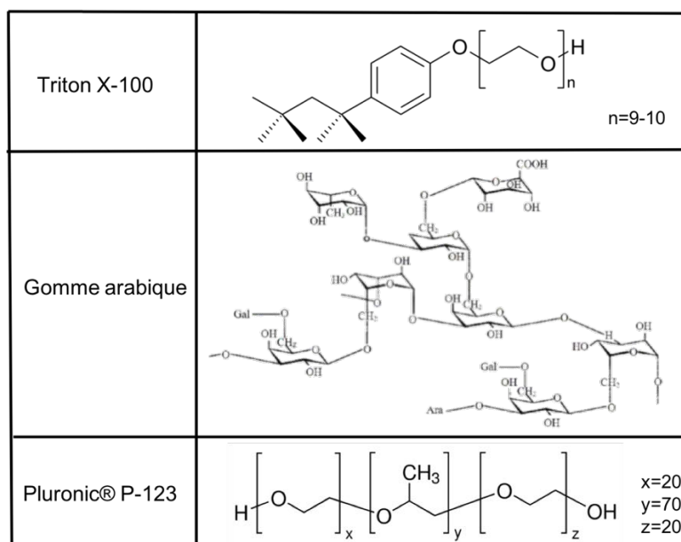
Figure II. 5 : Récapitulatif des trois tensioactifs utilisés et leur formule développée respective
