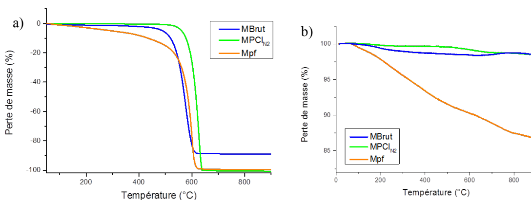
Figure V. 2 : Thermogrammes des échantillons bruts (MBrut) (courbe bleue) ; purifiés MPCl_{N2} (courbe verte) et fonctionnalisés (MPf) (courbe orange) ; a) sous air et b) sous hélium
