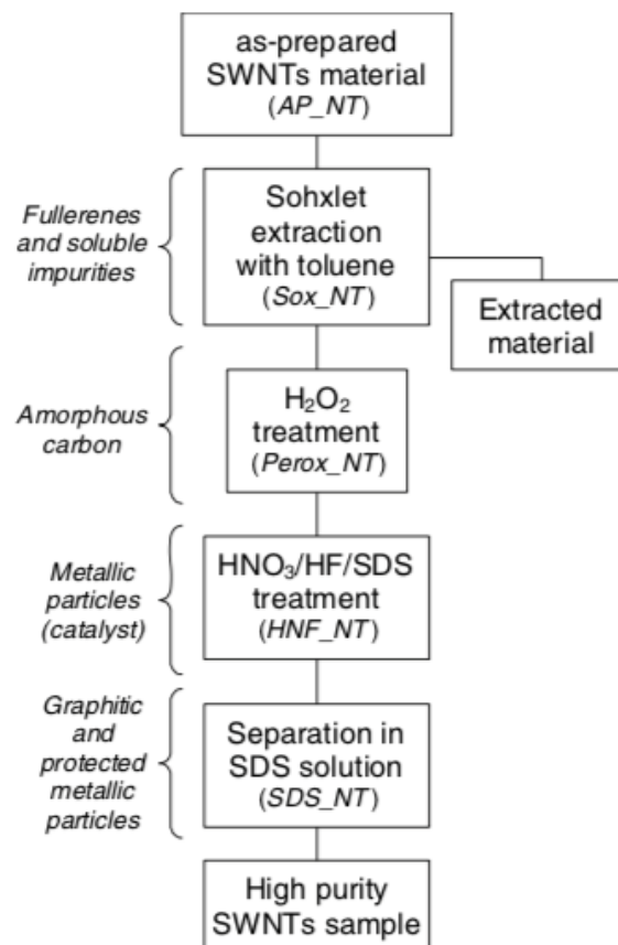
Figure I. 19 : Exemple de purification multi-étape avec le type de traitement dans les encadrés et les impuretés éliminés à leur gauche 117
