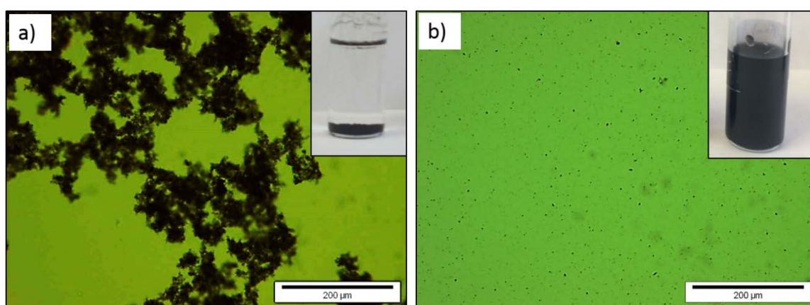
Figure V. 14 : Images de microscopie optique des MWCNTs fonctionnalisés ( MPf_{enz} ) dans a) la solution tampon Tris et b) l'eau à pH 10. L'aspect visuel de la dispersion associée est visible dans le coin en haut à droite des images respectives.
