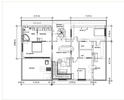
2 1er étage Copie 1 1:100
