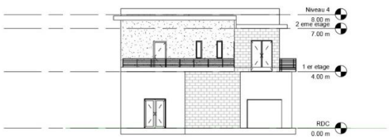
4 Est Copie 1 1:100
