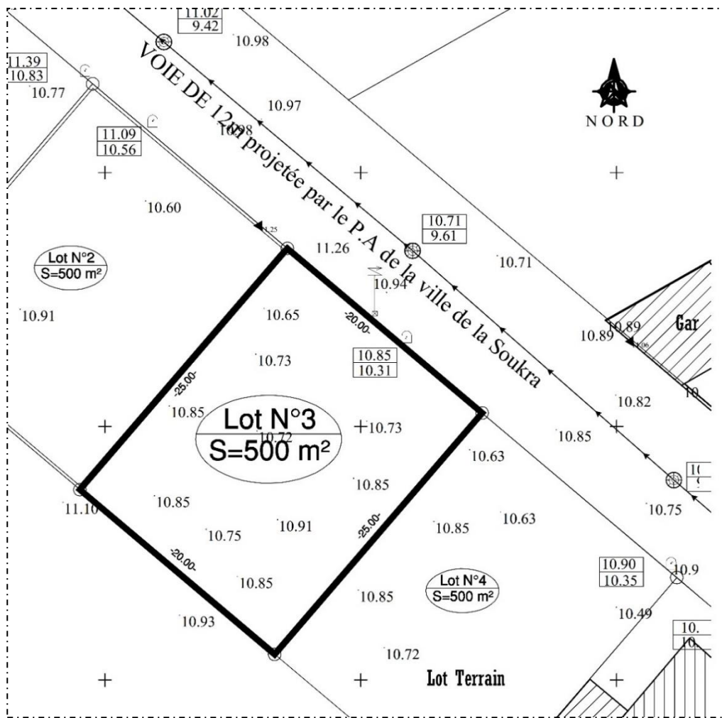
Extrait du levé topographique du terrain
