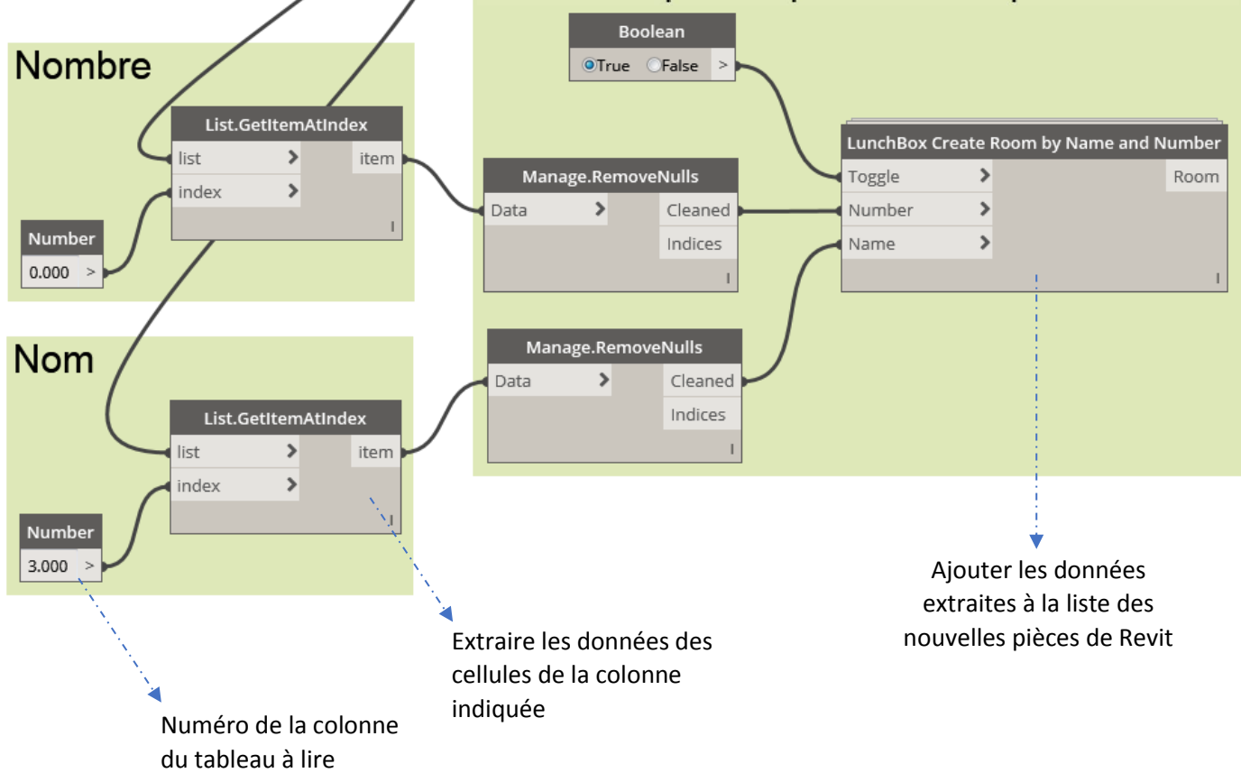
Figure 61 Capture d'écran Dynamo, script d'ajout des pièces du programme à Revit
