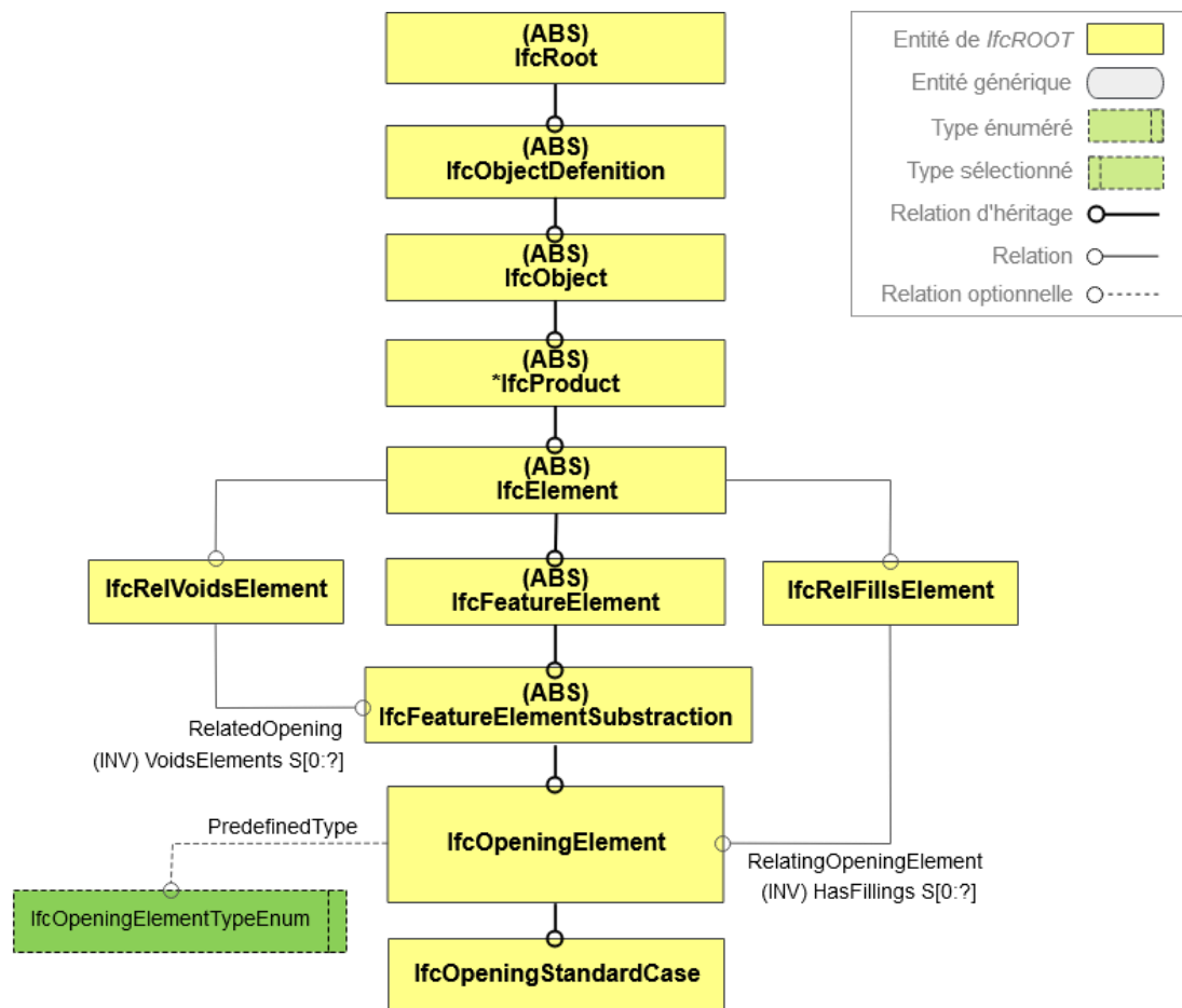
Figure 43 Schéma simplifié de la spécification des éléments d'ouverture (version IFC4 Add2).
