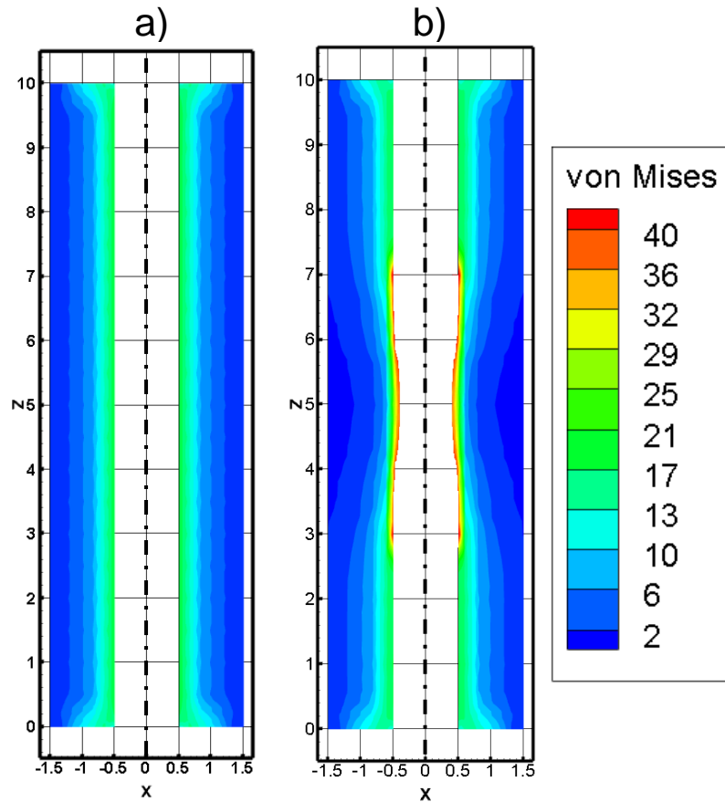
Figure 4. 13 : Impact d'une plaque d'athérome localisée dans un tube soumis à une pression interne sur la contrainte de von Mises dans le plan (Oxz) a) sans plaque d'athérome ; b) Avec plaque d'athérome
