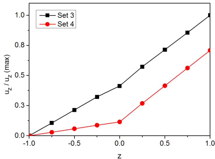
Figure 4. 3 : Validation du contact – Propriétés macroscopiques différentes : Déplacement axial
