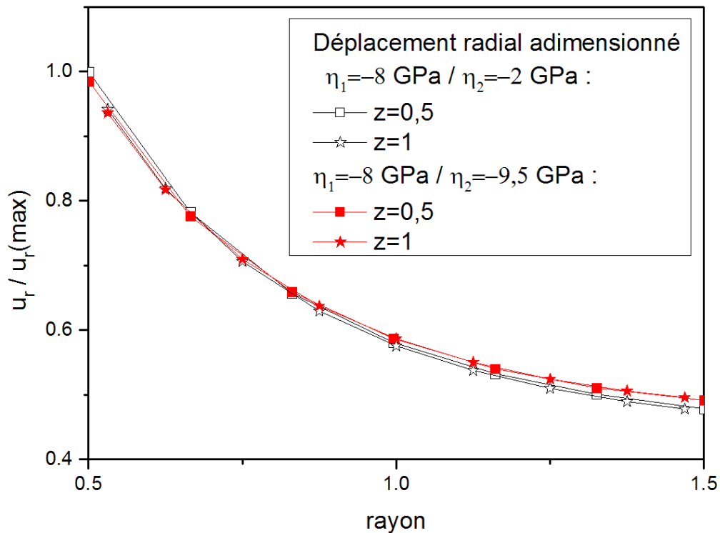
Figure 3. 18 : Déplacement radial adimensionné d'un tube de hauteur 1 soumis à une pression interne et dont la non-homogénéité est radiale
