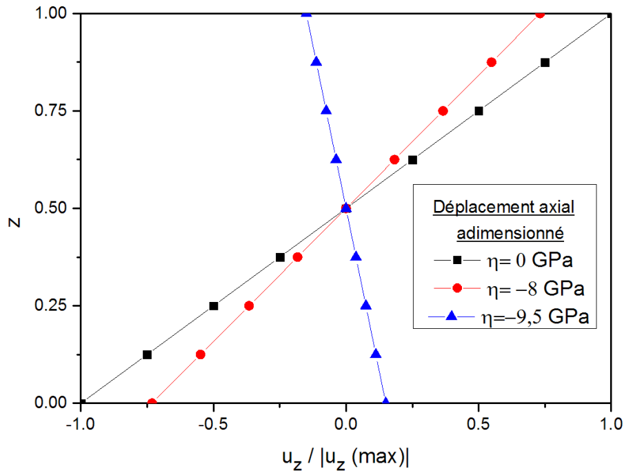
Figure 2. 12 : Déplacement axial adimensionné d'un tube soumis à une pression externe pour des échantillons possédant différents paramètres de couplage
