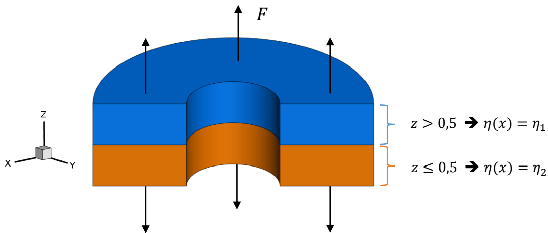
Figure 3. 7 : Tube soumis à une traction, possédant une non-homogénéité axiale
