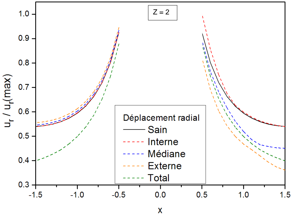
Figure 3. 32 : Influence d'une zone rigidifiée de taille différente sur le déplacement radial le long d'une droite passant par le centre de cette zone ( y=0 ; z=2 )
