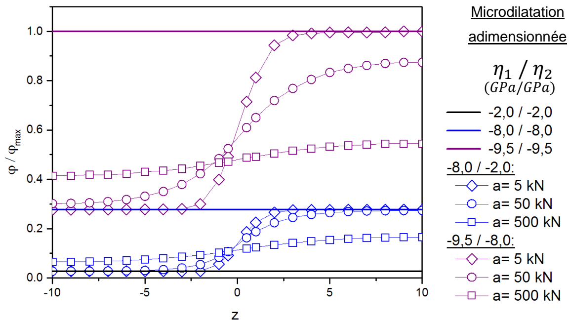
Figure 3. 5 : Évolution de la microdilatation le long d'une barre dont le paramètre de couplage \eta(x) dépend de la position et soumise à une sollicitation de traction pour différentes valeurs du paramètre a
