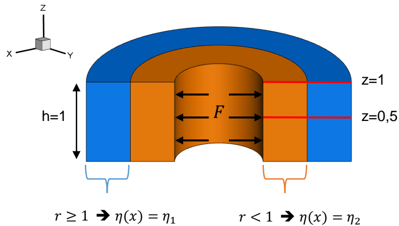
Figure 3. 17 : Tube soumis à une pression interne possédant une non-homogénéité radiale
