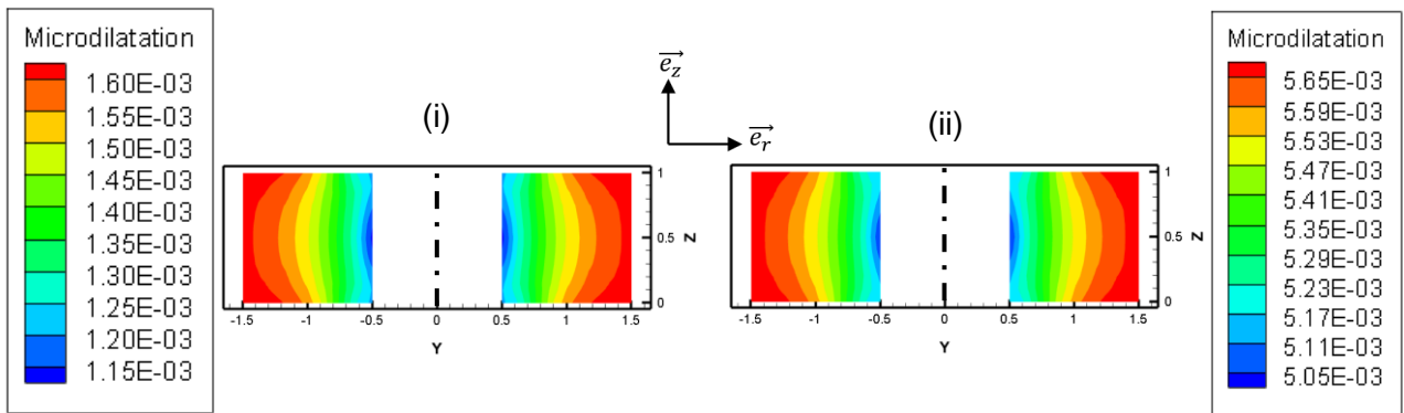
Figure 2. 15 : Microdilatation d'un tube soumis à une pression interne (i) set 1 ( \eta = -8 \text{ GPa} ) ; (ii) set 2 ( \eta = -9,5 \text{ GPa} )
