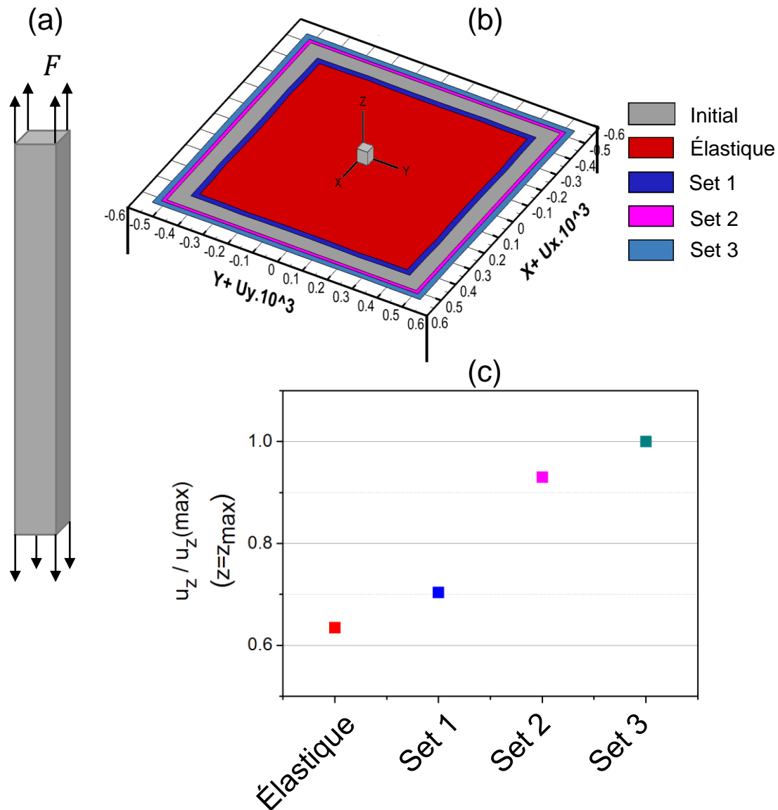
Figure 2. 7 : Essai de traction sur un parallélépipède : (a) Géométrie et chargement (b) Déplacement transverse (c) Déplacement axial maximum
