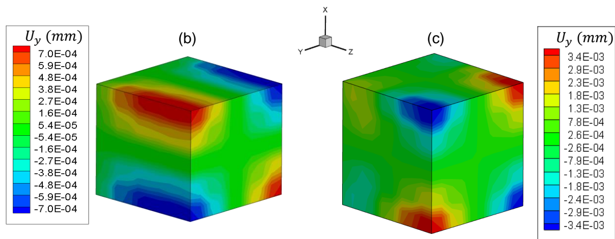
Figure 2. 8 : Flexion d'un cube (a) Géométrie et chargement Déplacement transverse de l'échantillon pour (b) un milieu élastique auxétique et (c) un milieu à microdilatation : set2 ( E=2.38 GPa)
