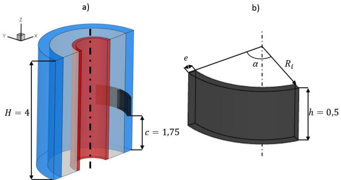
Figure 3. 24 : Artère et inclusion a) Position de l'inclusion au sein de l'artère ; b) Définition géométrique de l'inclusion
