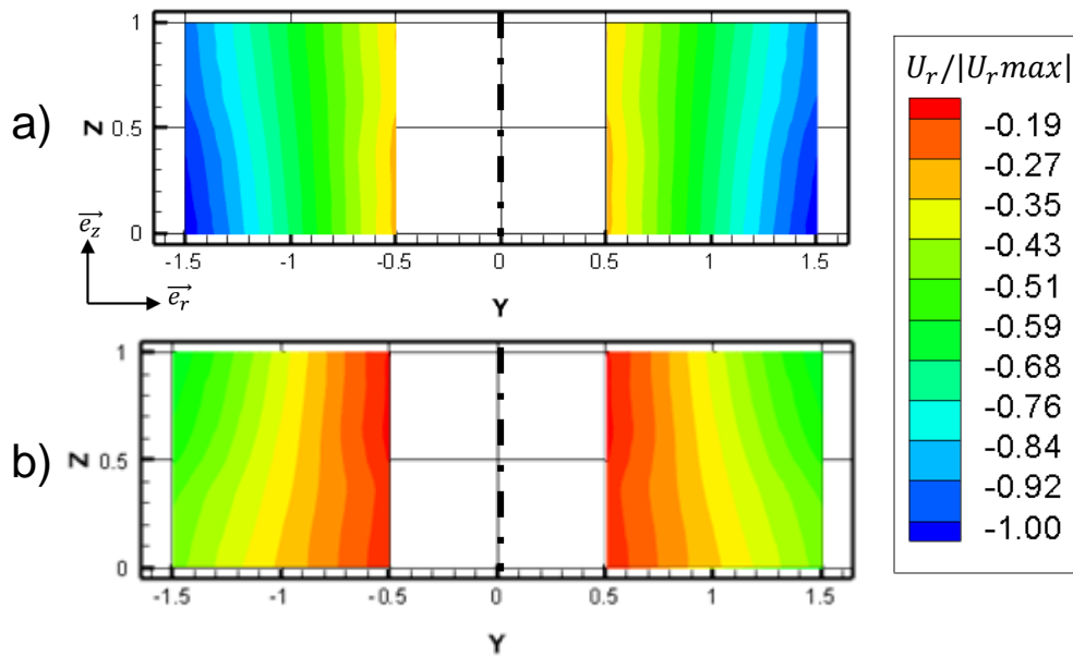
Figure 3. 8 : Déplacement radial adimensionné d'un tube soumis à une traction et dont la non-homogénéité est axiale : a) Set 1 : \eta_1 = -8GPa, \eta_2 = -2GPa b) Set 2 : \eta_1 = -8GPa, \eta_2 = -9.5GPa
