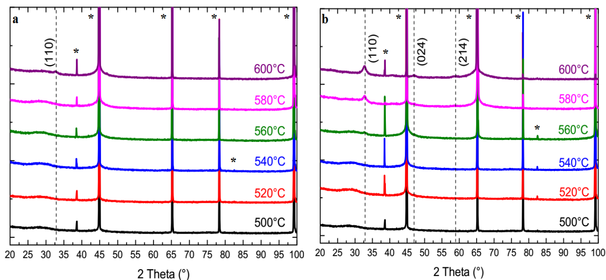
Figure 33. Clichés de diffraction des rayons X de couches minces de \text{LaCoO}_3 de 200 nm recuit pendant a – 5 minutes, b – 10 minutes. L'astérisque « * » désigne les pics correspondant au substrat d'aluminium
