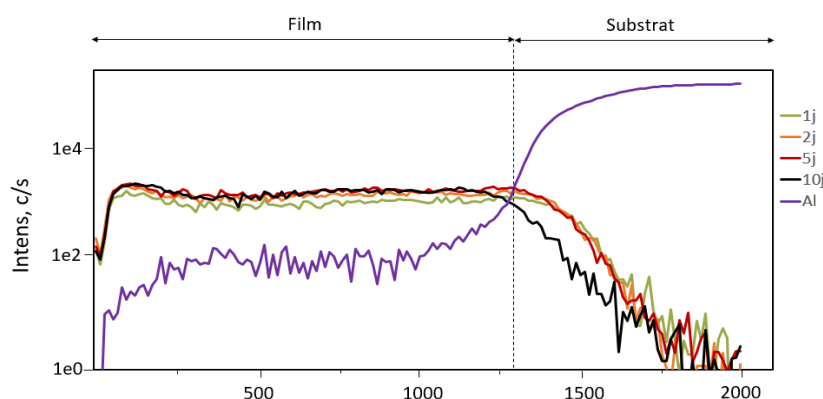
Figure 52. Profils d'oxygène et d'aluminium pour les films de 600 nm issus de la machine semi-industrielle « vieillis » à l'air pendant 1, 2, 5 et 10 jours puis recuits pendant 10 minutes à 600°C
