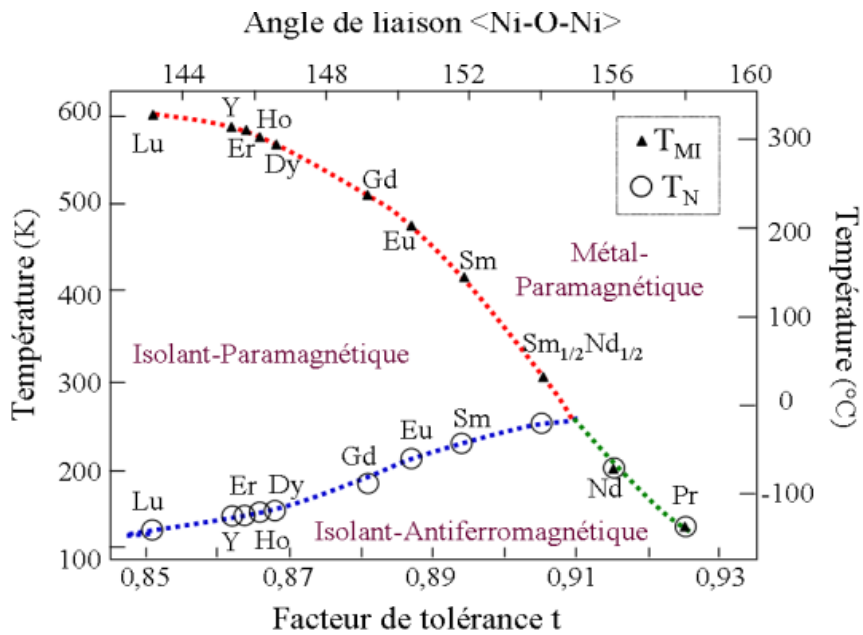
Figure 13. Diagramme de phases des composés ReNiO 3 (Re = terre rare) en fonction de la température et du facteur de tolérance t qui est lié à l'angle de liaison <Ni-O-Ni>, d'après [99]
