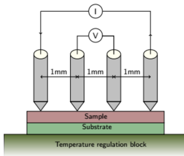
Figure 26. Représentation schématique du montage Mesure 4-pointes
