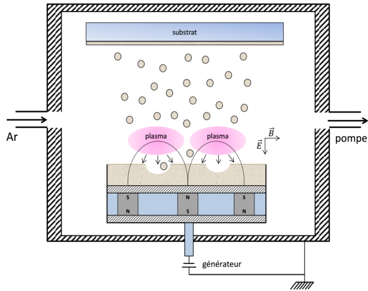
Figure 17. Représentation schématique de la pulvérisation cathodique magnétron
