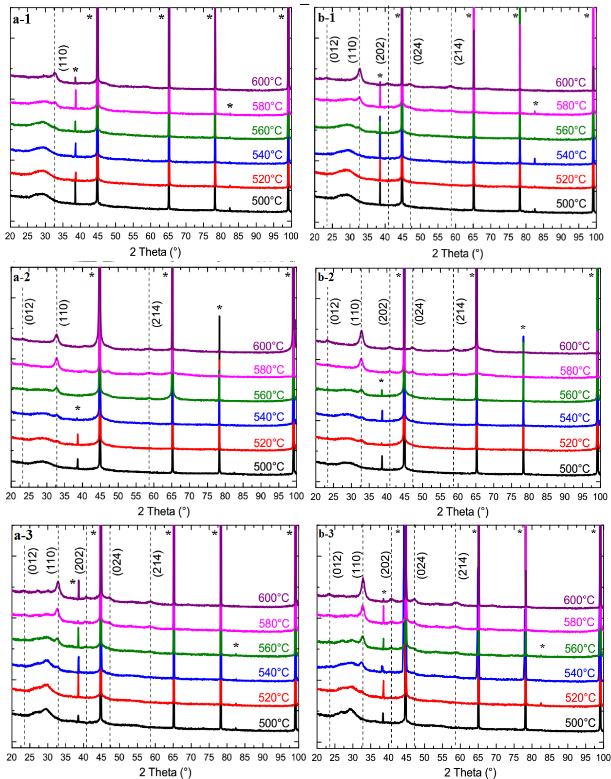
Figure 34. Clichés de diffraction des rayons X pour les de recuits de 5 minutes (diffractogrammes indexés avec la lettre a) et 10 minutes (diffractogrammes indexés avec la lettre b) pour les échantillons de 1 – 400 nm, 2 – 600 nm, 3 – 800 nm. L’astérisque « * » désigne les pics correspondant au substrat d’aluminium
