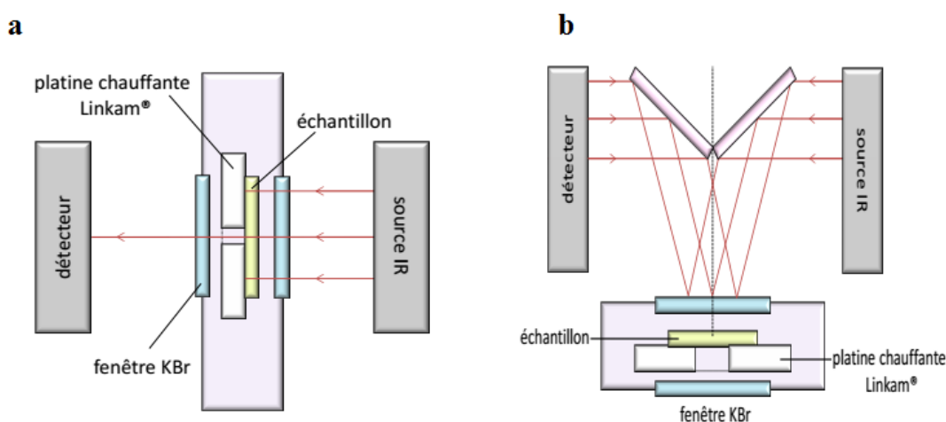
Figure 24. Représentation schématique du banc de mesure FTIR avec le dispositif Linkam a – en transmittance, b – en réflectance
