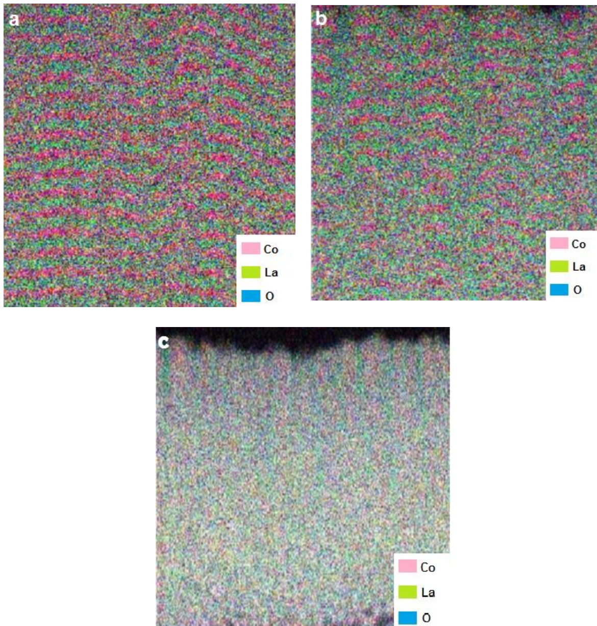
Figure 41. Cartographies EDS agrandies pour les films de \text{LaCoO}_3 de 600 nm recuits à a – 520°C pendant 10 minutes, b – 600°C pendant 2 minutes, c - 600°C pendant 10 minutes
