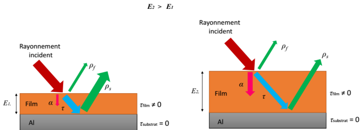
Figure 36. Schématisation de l'évolution de la réflectance globale du système film/substrat avec l'épaisseur du film
