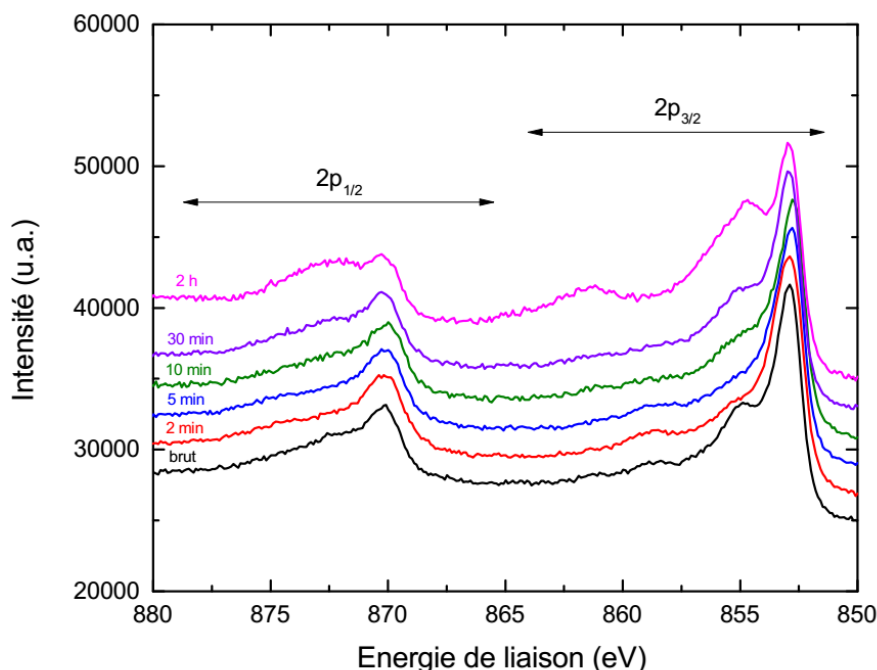
Figure 78. Spectres XPS réalisés sur le niveau Ni2p pour les échantillons avant le recuit et après le recuit à 750°C pendant 2, 5, 10, 30 minutes et 2 heures
