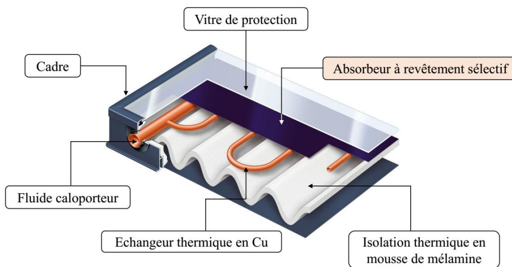
Figure 1. Représentation schématique d'un panneau solaire thermique Viessmann
