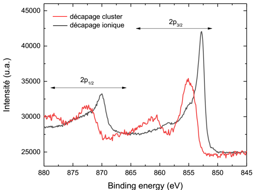
Figure 77. Spectres XPS réalisés sur le niveau Ni2p ; comparaison du décapage ionique et décapage cluster
