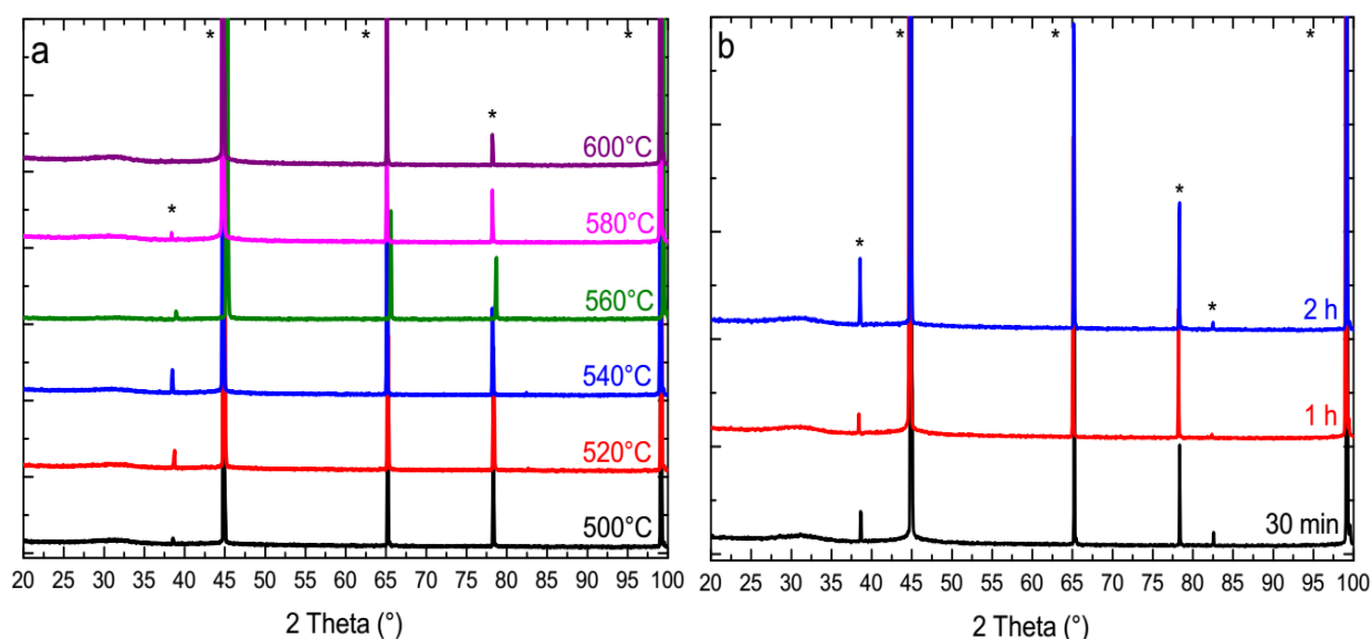
Figure 72. Clichés de diffraction des rayons X pour les échantillons de \text{SmNiO}_{3-\delta} recuits a – pendant 10 minutes ; b – à 600^\circ\text{C} pour les temps différents. Le symbole « * » désigne les pics correspondant au substrat d'aluminium
