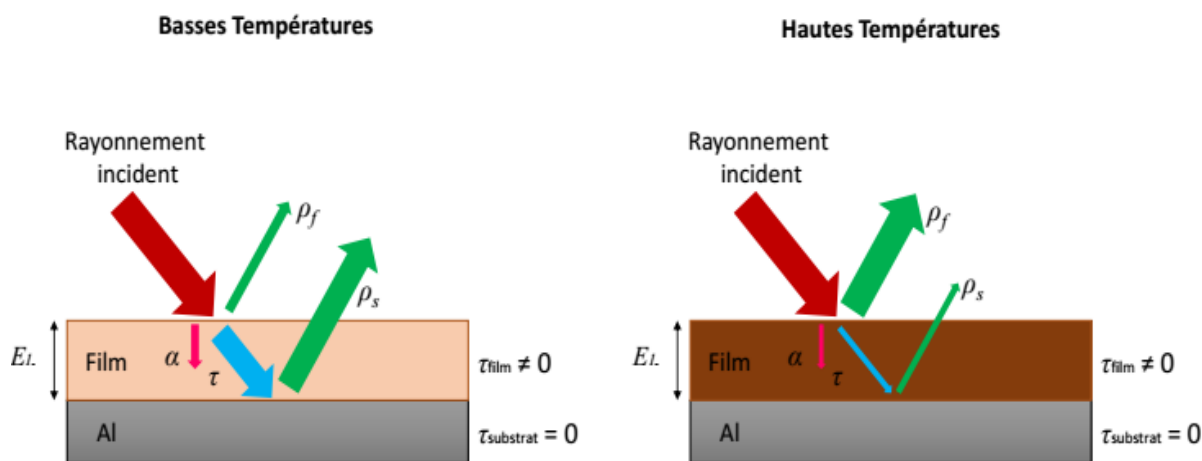
Figure 37. Schématisation de l'effet thermo-chrome
