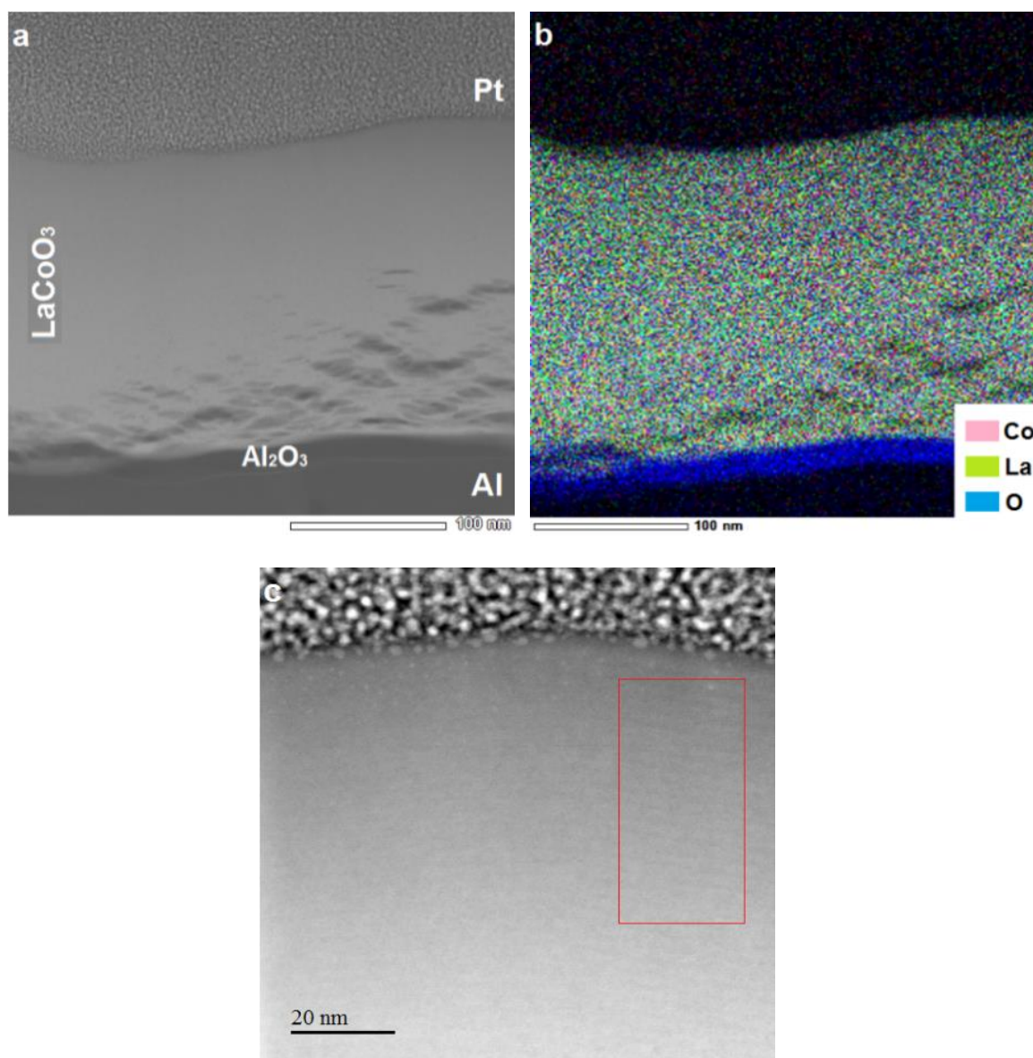
Figure 50. Micrographie STEM (a), cartographie EDS associée (b) et micrographie STEM agrandie (c) pour un film de LaCoO 3 de 200 nm
