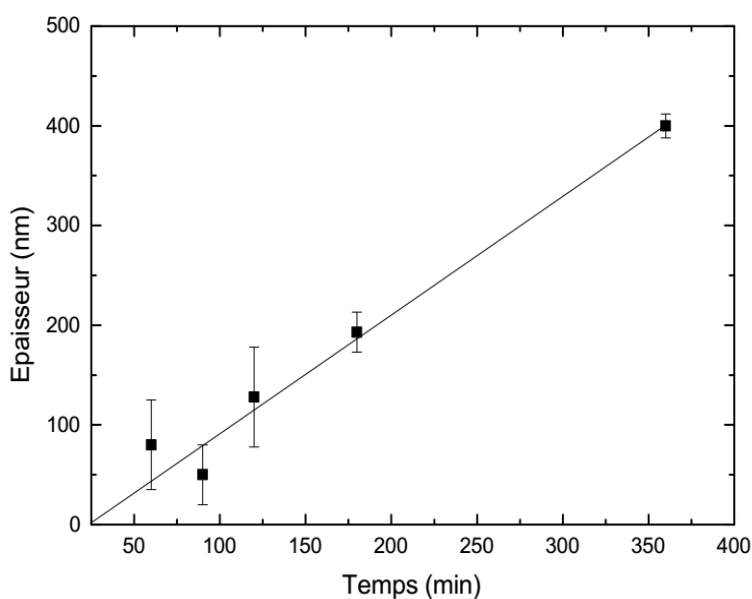
Figure 71. Évolution de l'épaisseur en fonction du temps de dépôt pour le film de SmNiO 3-δ
