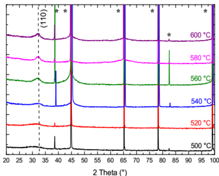
Figure 63. Clichés de diffraction des rayons X pour les échantillons de 200\text{ nm} recuits pendant 10 minutes
