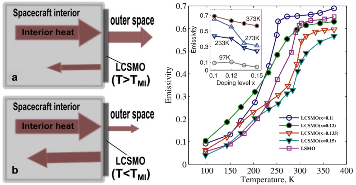
Figure 4. Principe de la régulation thermique d'un satellite par un film mince \text{La}_{0,7}\text{Ca}_{0,3-x}\text{Sr}_x\text{MnO}_3 (a) état métallique ( T > T_{MI} ), (b) état isolant ( T < T_{MI} ) et les courbes d'émissivité en fonction de la température [26]
