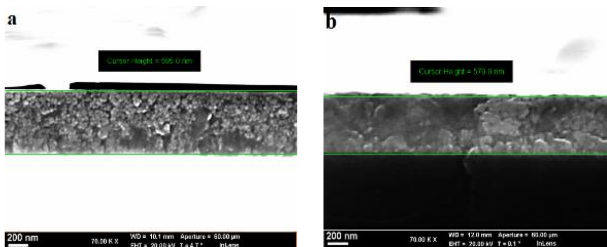
Figure 30. Micrographie MEB en section transverse pour les films d'épaisseur initiale de 420 nm a – recuit à 500^\circ\text{C} pendant 2 minutes, b – recuit à 600^\circ\text{C} pendant 10 minutes
