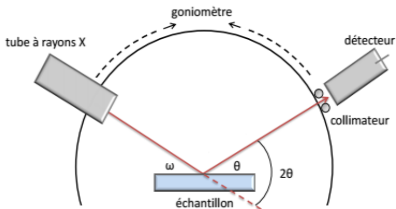
Figure 23. Schéma du diffractomètre à configuration Bragg-Bretano
