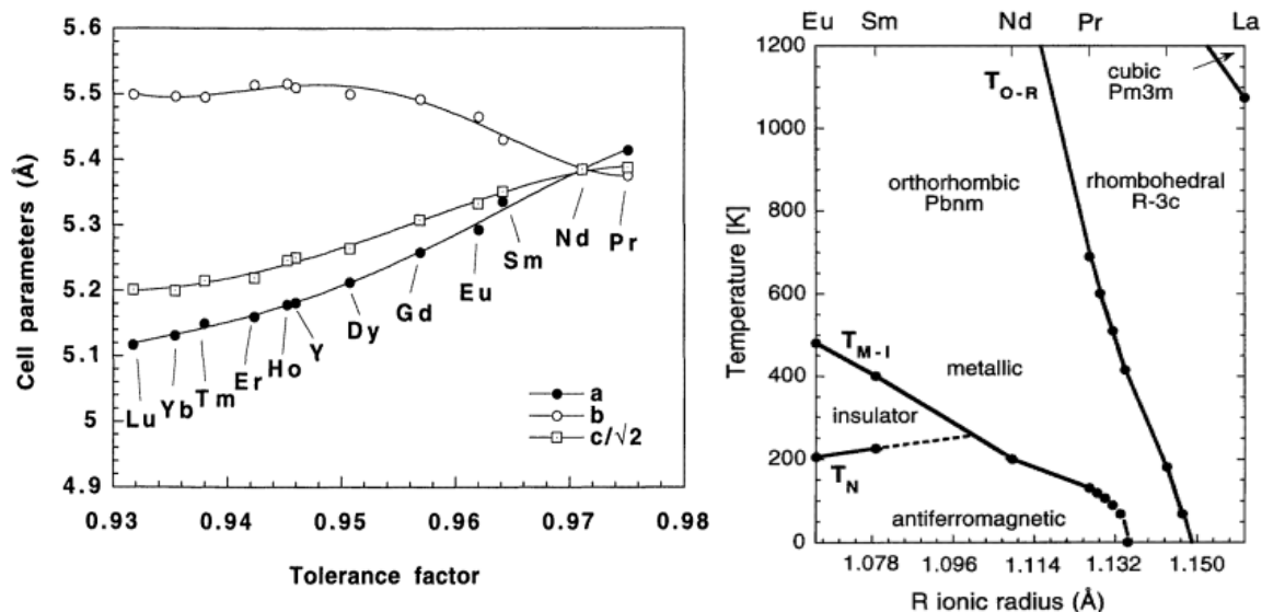
Figure 12. Variation des paramètres de maille en fonction du facteur de tolérance de Goldschmidt (à gauche) et diagramme de phases pour les pérovskites de la famille \text{ReNiO}_3 (à droite) [97]
