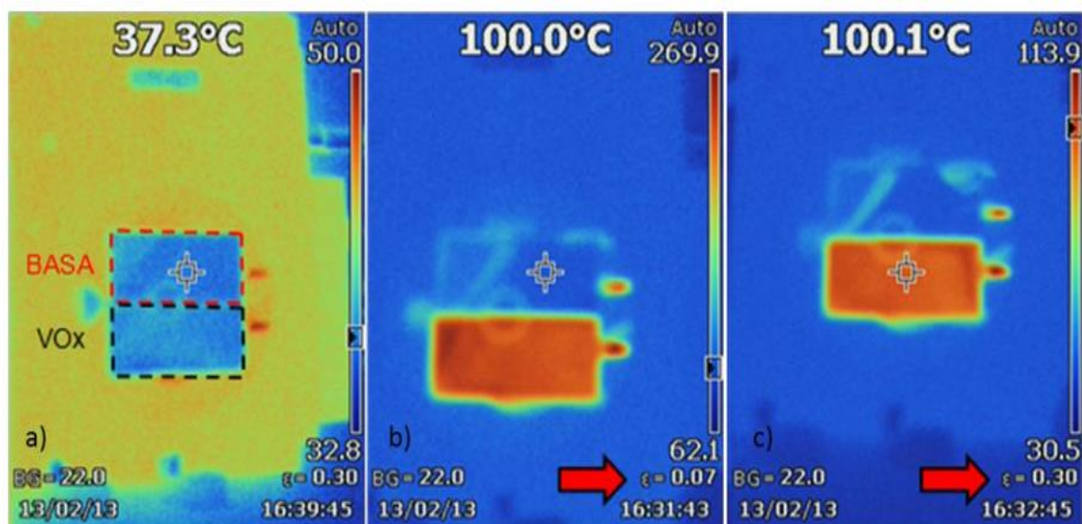
Figure 5. Images thermiques (a – c) d'un capteur solaire hybride recouvert par la couche sélective de l'ancienne génération (partie « BASA ») et le film mince à la base de l'oxyde de vanadium (partie «VOx») [5,6]
