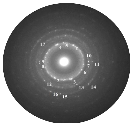
Figure 43. Cliché de diffraction pour un échantillon de LaCoO 3 recuit à 600°C pendant 10 minutes
