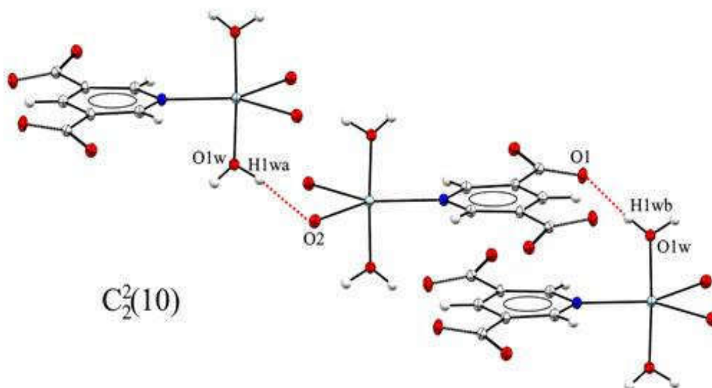
Figure IV-10: Graphe C_2,2(10) décrivant les interactions intermoléculaires ( O1w-H1wa \cdots O2^i , O1w-H1wb \cdots O1^{ii} )
