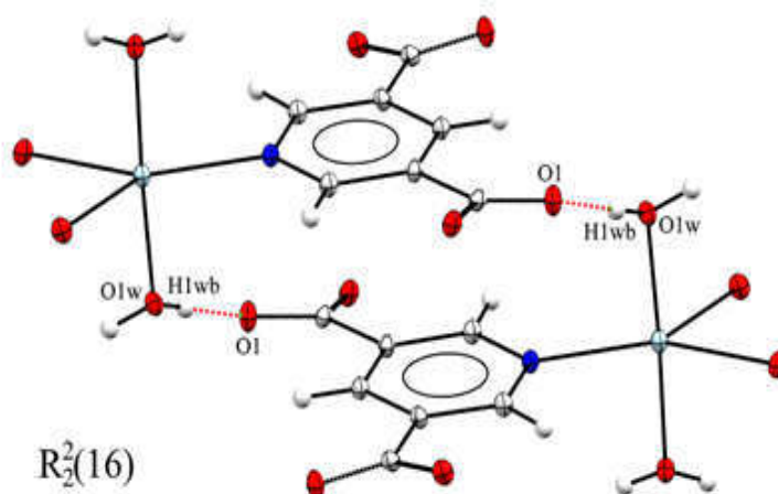
Figure IV-9: Graphe R_2,2(16) décrivant l'interaction intermoléculaire ( O1w-H1wb \cdots O1^{ii} )
