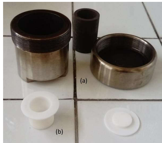
Figure I-25: Schéma d'un réacteur en acier inoxydable (a) et d'une chemise en téflon (b)
