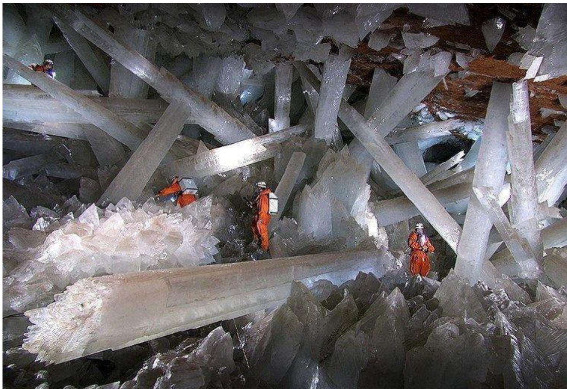
Figure I-18: Cristaux naturels de gypse dans les mines de Naïca dans l'Etat de Chihuahua au Mexique ( https://alchetron.com/Naica-Mine )
