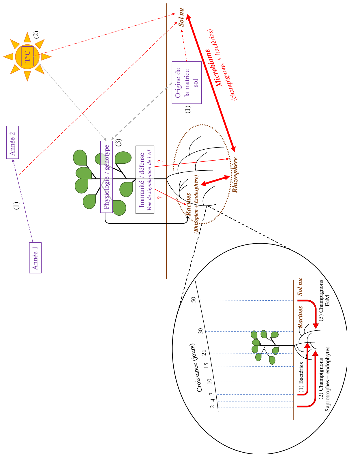
Figure 46 - Modèle de synthèse de la régulation du microbiote du peuplier réalisé à partir des résultats obtenus au cours de cette thèse.
