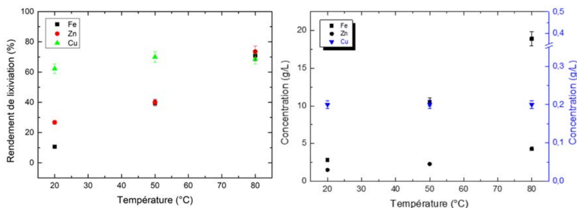
Figure 5-3 : Influence de la température pour un rapport solide/liquide de 1/10 ; gauche : a = rendement de lixiviation, droite : b = concentrations massiques.
