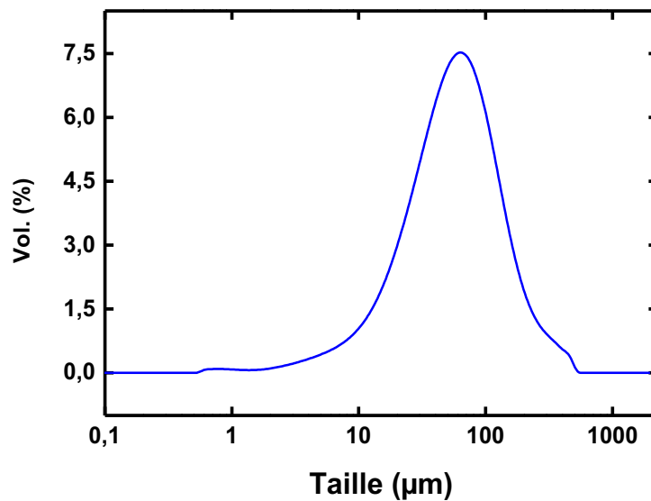
Figure 3-21 : Analyse granulométrique de la blende Glencore
