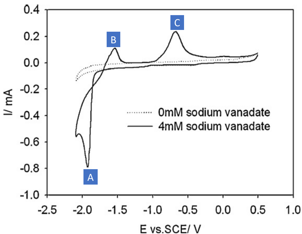
Figure 2-21: Comportement redox du vanadium ( E = -2,1 \text{ V} à 0,6 \text{ V/ECS} , Balayage à 100 \text{ mV/s} ) dans 1 \text{ M NaOH} à 40 \text{ °C} [96].
