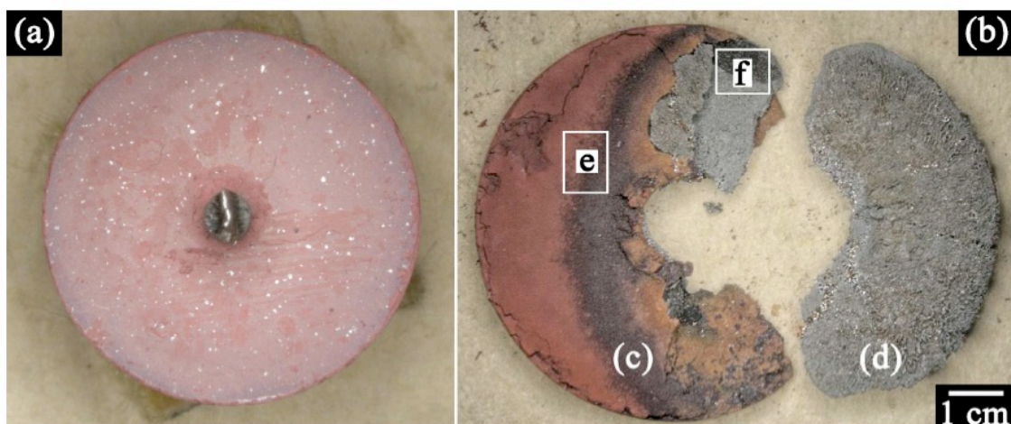
Figure 2-10: Images obtenues par microscopie optique des produits obtenus dans NaOH 60 % à 1,65 V et 110°C pendant 2h. (a) boulette de Fe 2 O 3 avant électrodéposition, (b) produit après l'opération.
