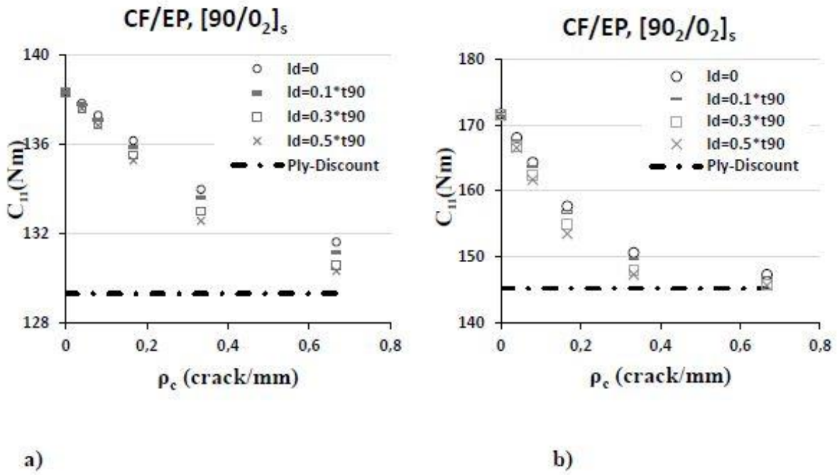
Figure 9: L'effet de la delamination sur la rigidité en flexion pour des composites à plis croisés CF/EP avec des fissures matricielles au plis 90^\circ
