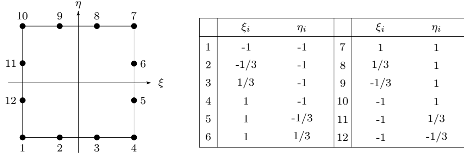
Fig. A.3 Quadrangle à 12 nœuds.
