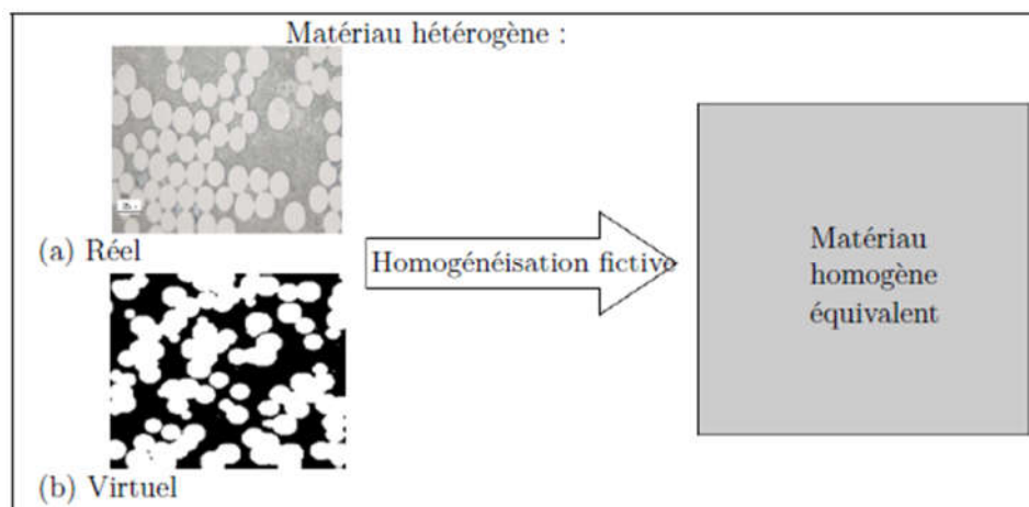
Figure 6 : Principe d'homogénéisation d'un matériau hétérogène [81]
