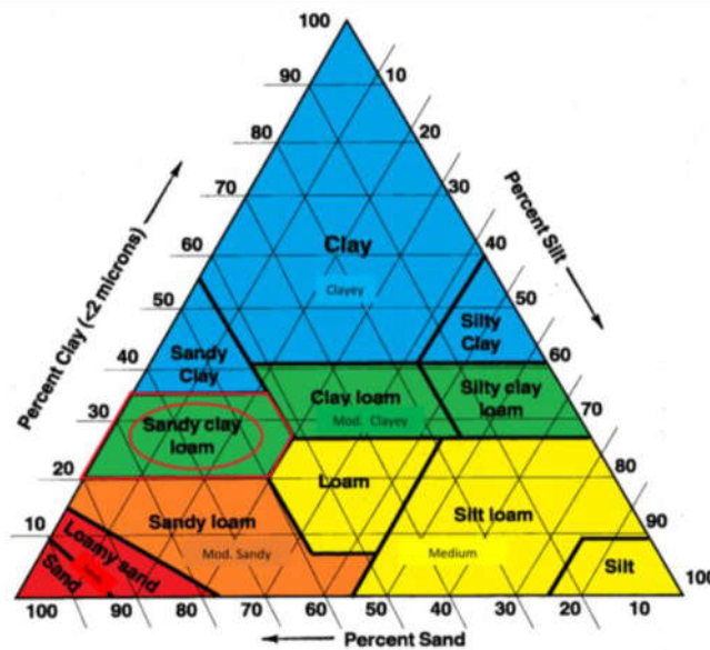
Figure 21 : Texture triangulaire du sol
