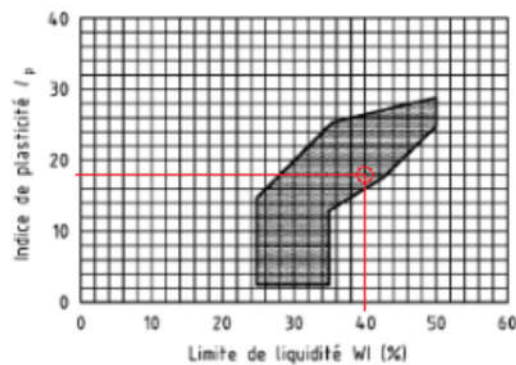
Figure 20 : Diagramme de plasticité (XP P 13-901)
