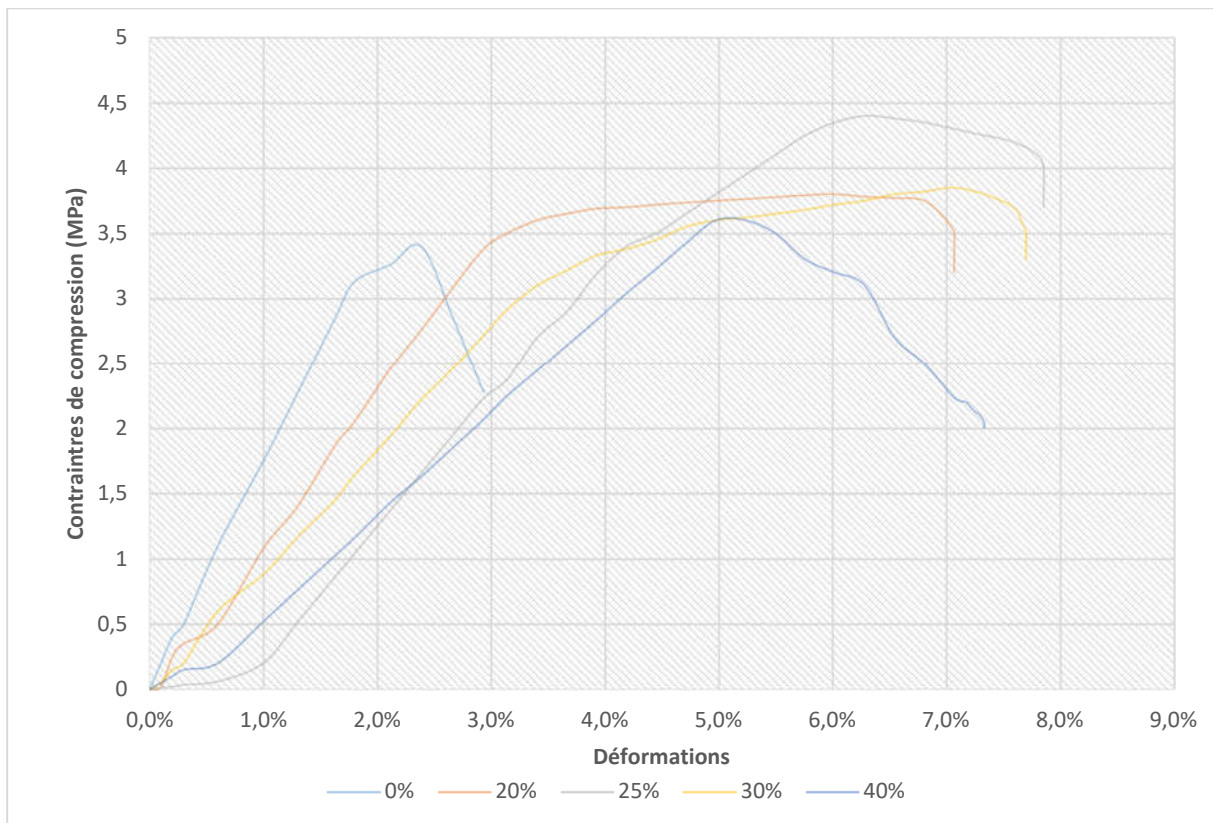
Figure 34 : Courbe contrainte-déformation en compression des éprouvettes prismatiques
