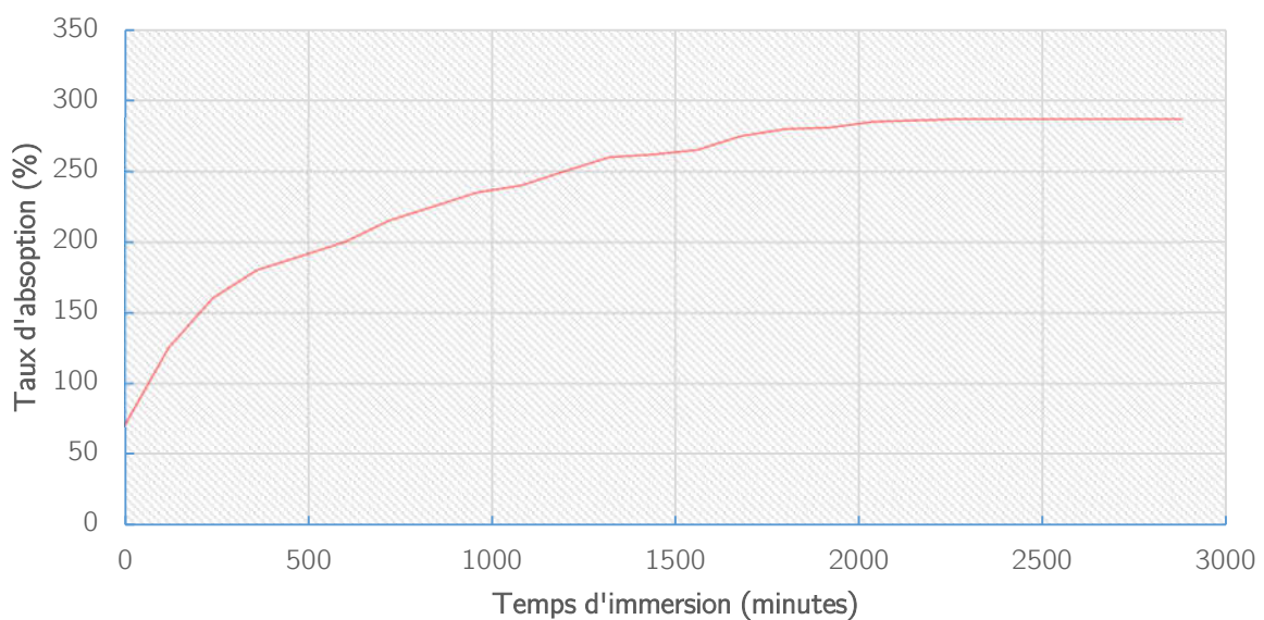
Figure 25 : Cinétique d'absorption d'eau par les pailles
