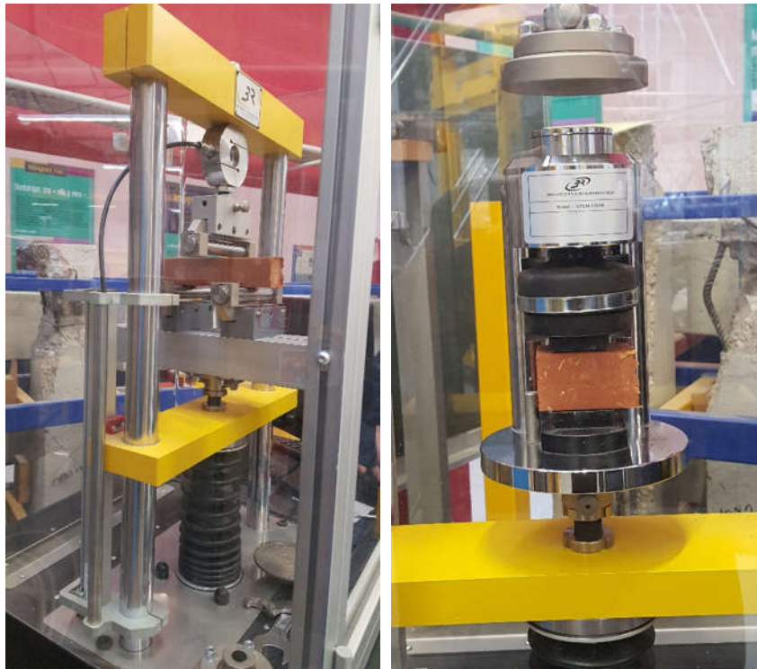
Figure 32 : Dispositifs d'essais de flexion et de compression
