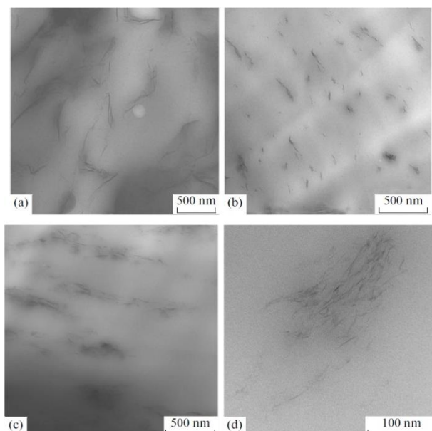
Figure 1.36: Micrographies MET de nanocomposites iPP/GNP produits par polymérisation in situ avec : (a) ajout simple de la charge GNP (1,1 %vol.), (b) charge GNP traitée par ultrasons pendant 20 min (0,9 %vol.) et (c) et (d) pendant 60 min (0,1 %vol.) [306].
