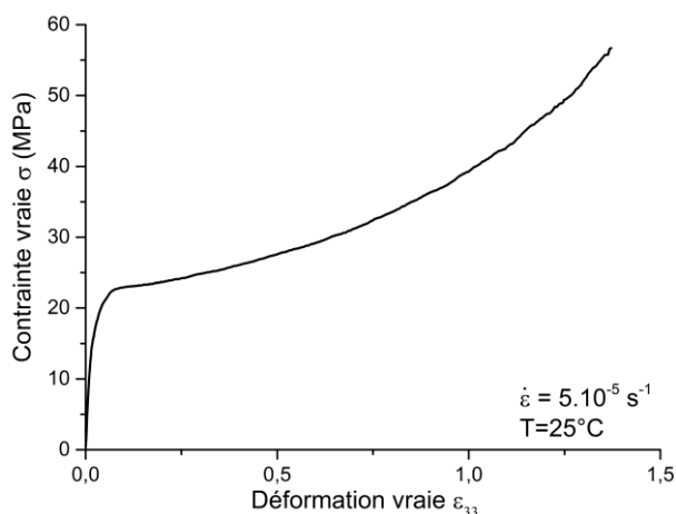
Figure II.39: comportement mécanique vrai CA 100 + T3000 1:1 en traction uniaxiale.
