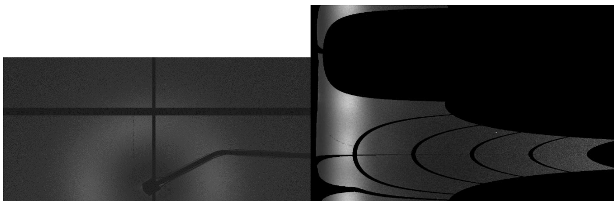
Figure A.16 : Cliché SAXS et « cake » du matériau CA 100 T3000 3:2
