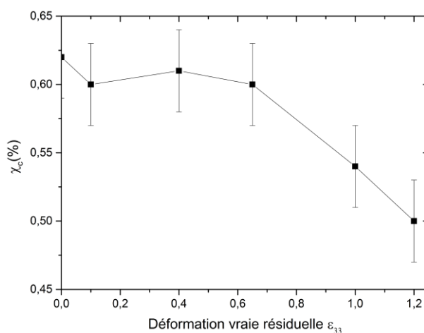
Figure II.36: Évolution du taux de cristallinité calculée par diffraction des rayons X de la matrice CA 100 THF 100 en fonction de la déformation vraie résiduelle.
