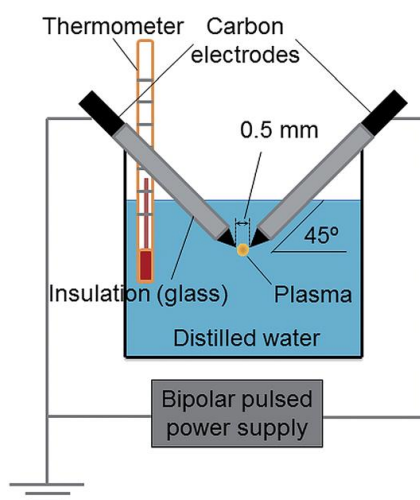
Figure 1.28: Montage expérimental pour l'exfoliation du graphène à partir d'électrodes de graphite par Lee et al. , 2014 [280].
