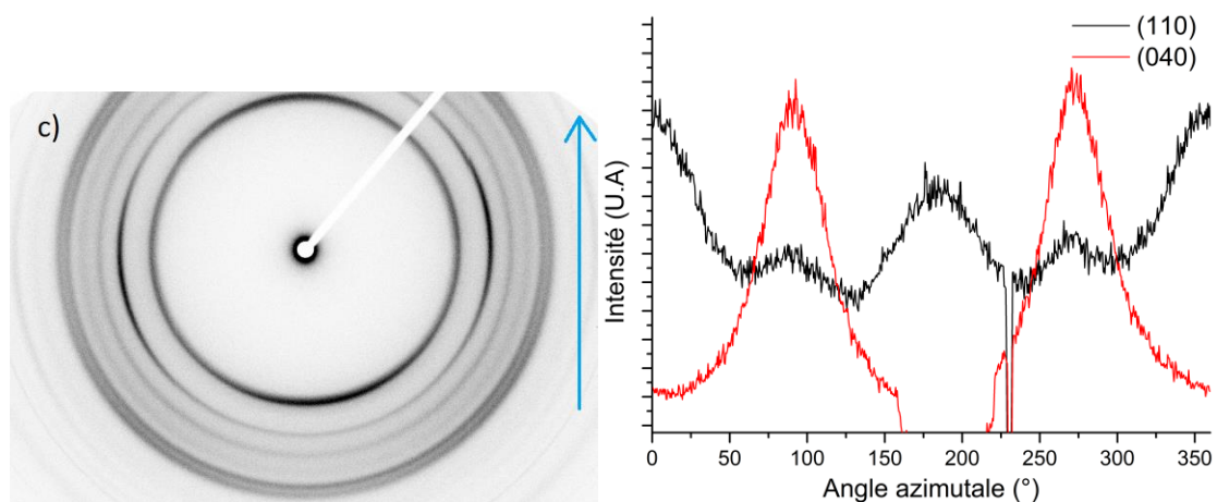
Figure A.58: Cliché WAXS 2D du CA 100 THF 100 1:1 KNG 180 3% m déformé à \epsilon_{33}=0,3 et profile azimuthale des plans de diffraction (110) et (040) du polypropylène.
