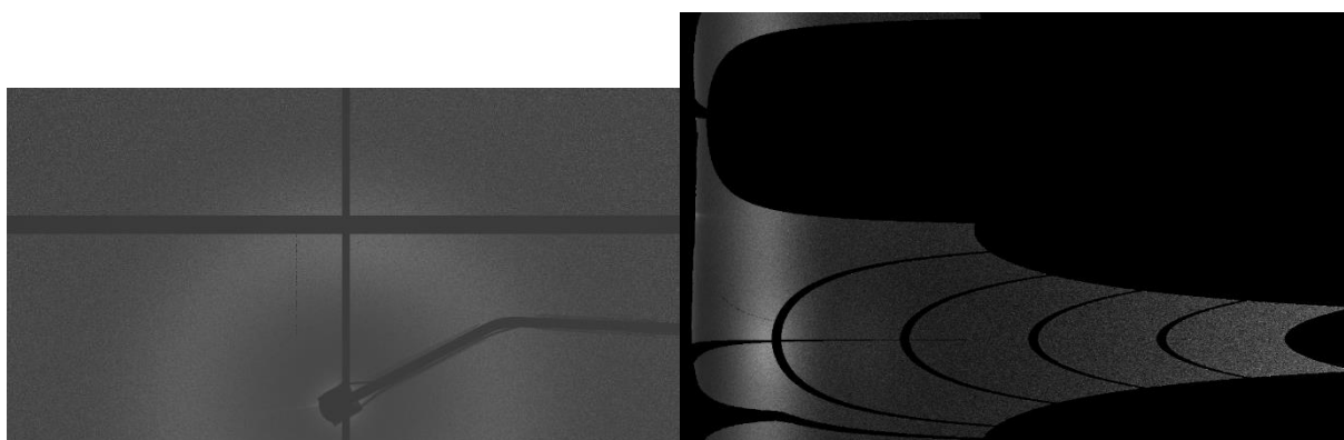
Figure A.15 : Cliché SAXS et « cake » du matériau CA 100 T3000 1:1
