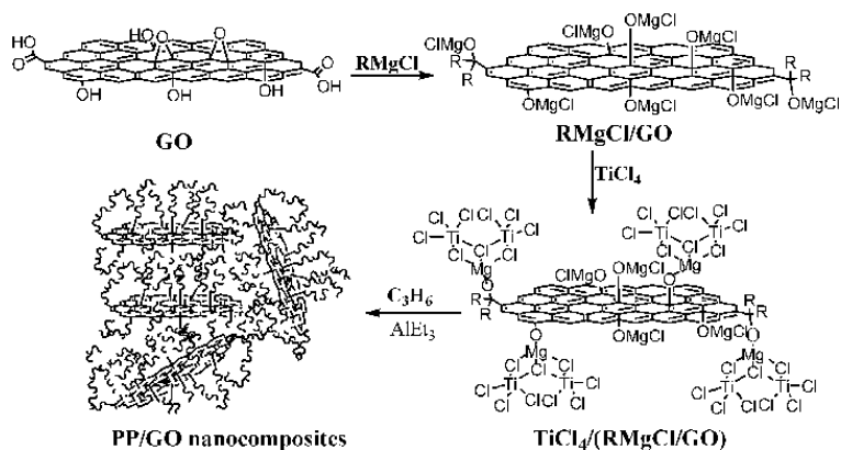
Figure 1.37: Fabrication d'un nanocomposite PP/GO par polymérisation Ziegler-Natta in situ [297].
