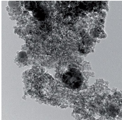
Figure I.26: Nanoparticules d'alumine, produits dans l'eau entre deux électrodes d'aluminium. [272]
