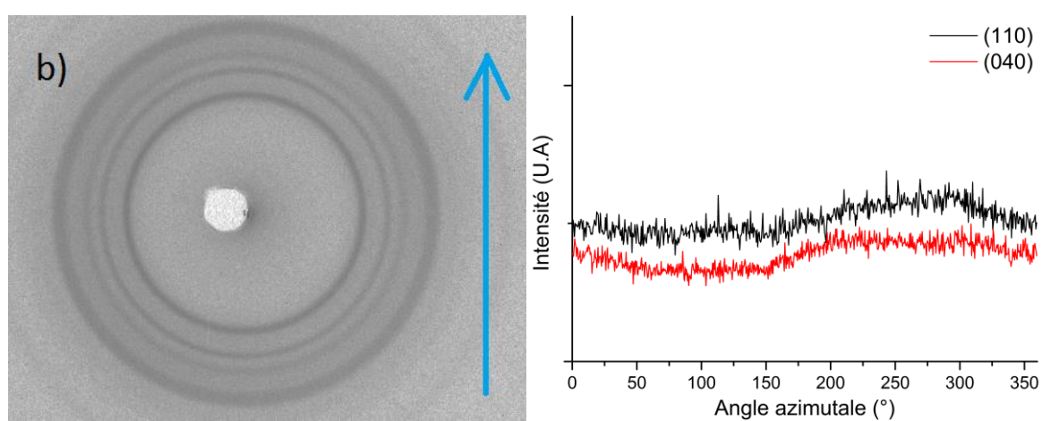
Figure A.42: Cliché WAXS 2D du CA 100 THF 100 1 :1 KNG 180 traité 3% m et profile azimutale des plans de diffraction (110) et (040) du polypropylène.
