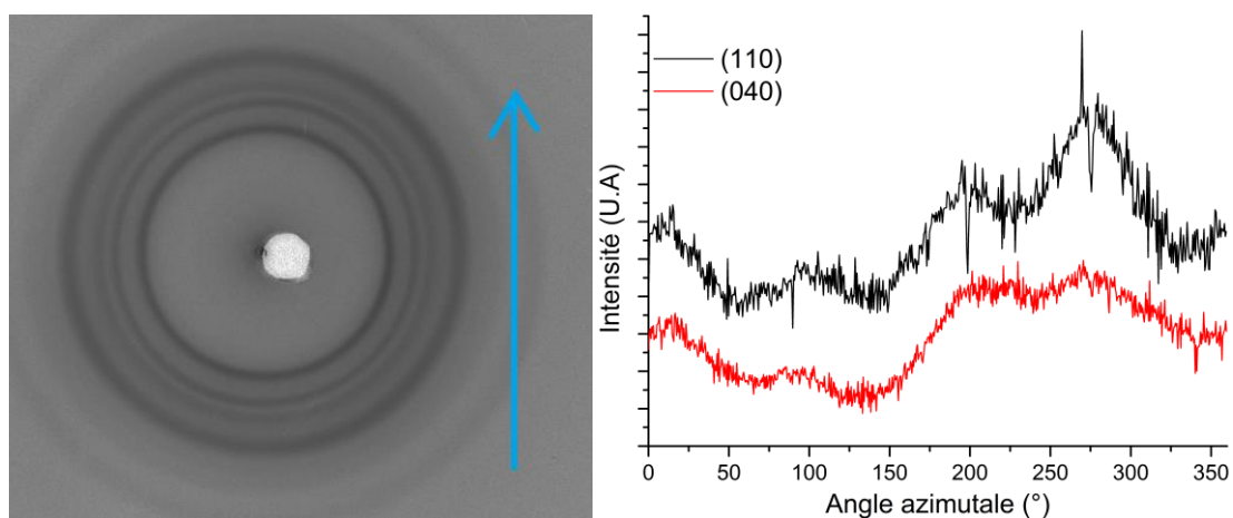
Figure A.25 : Cliché WAXS 2D du CA 100 T3000 1:3 et profile azimutale des plans de diffraction (110) et (040) du polypropylène.
