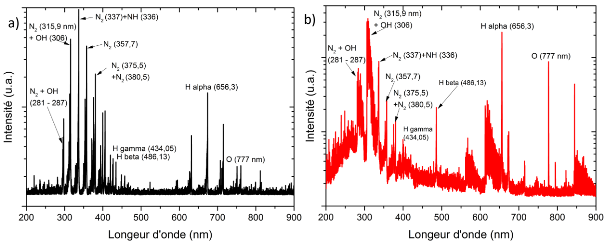
Figure III.7: Spectres d'émission du plasma gazeux après a) 5 minutes et b) 40 minutes de traitement.
