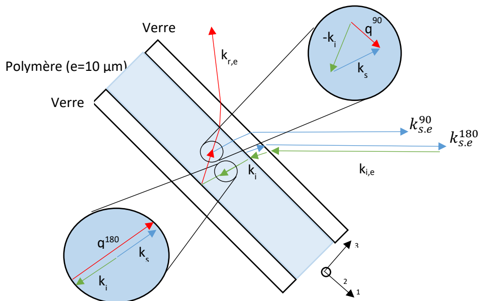
Figure I.66: Test Brillouin en configuration Rita employé pour caractériser les matériaux polymères.
