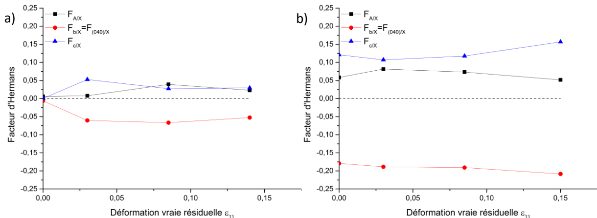
Figure 76: Evolution des facteurs d'Hermans des différentes directions cristallines avec la déformation vraie résiduelle des nanocomposites chargés à a) 1 %m, et b) 3 %m de KNG 180.
