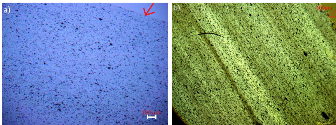
Figure III.35: Observation au microscope optique en transmission des nanocomposites chargés KNG 180 à a) 1 %, b) 3 %, c) 5 %, d) 10 %, e) 20 %. La flèche rouge indique la surface de la plaque injectée.
