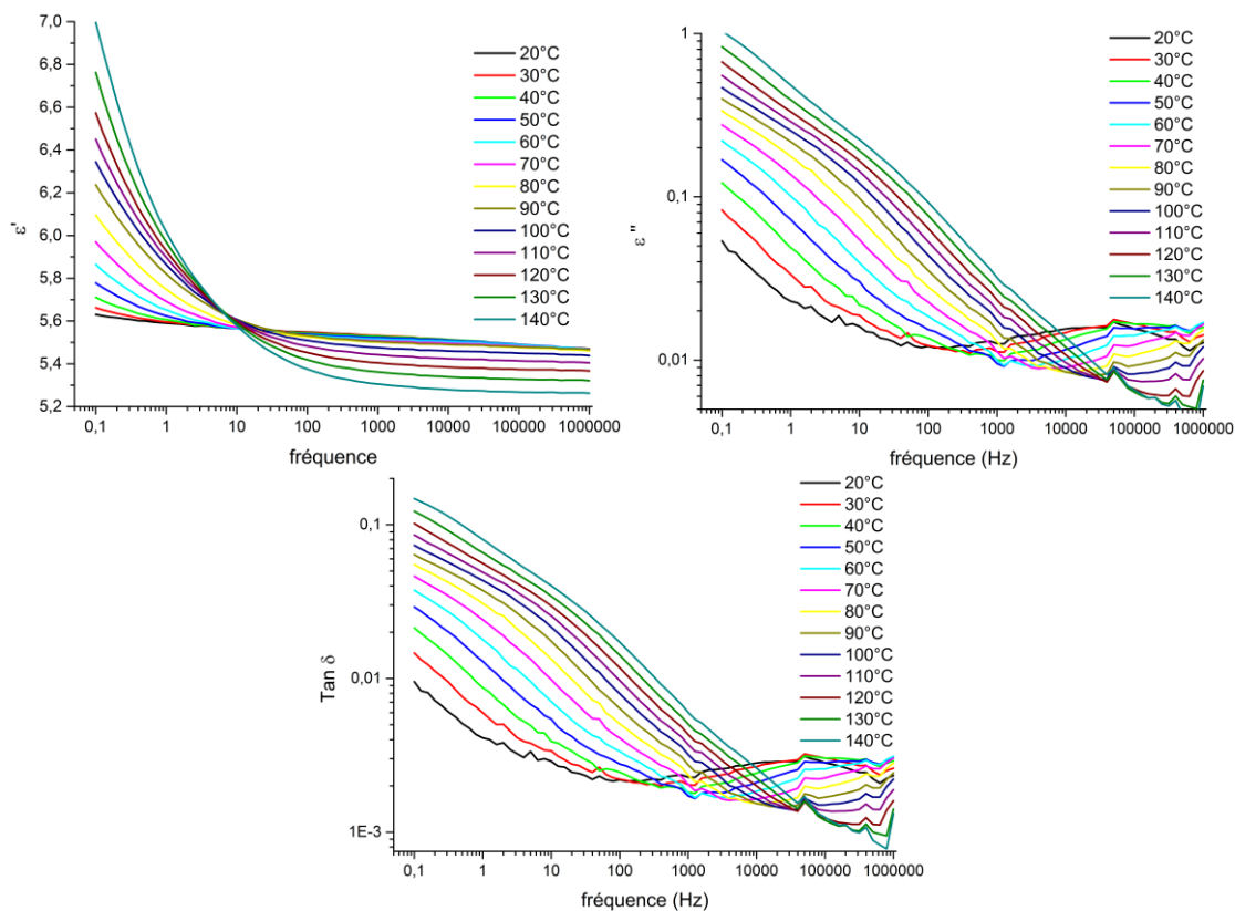
Figure A.61 : Spectre diélectrique \epsilon' , \epsilon'' , et \text{Tan } \delta en fonction de la fréquence du matériau CA 100 THF 100 1:1 KNG 180 1% m
