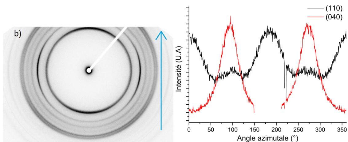
Figure A.57: Cliché WAXS 2D du CA 100 THF 100 1:1 KNG 180 3% m déformé à \epsilon_{33}=0,15 et profile azimuthale des plans de diffraction (110) et (040) du polypropylène.
