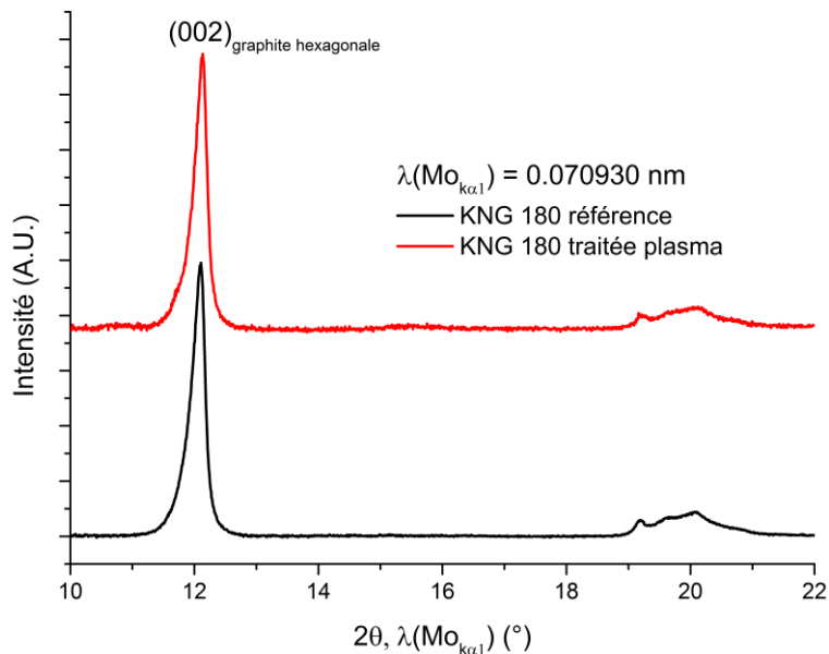
Figure III.16: Diffractogrammes des nano-charges de graphite KNG 180 avant et après le traitement par plasma.
