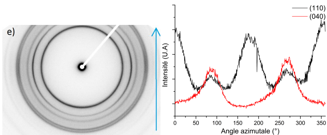
Figure A.53 : Cliché WAXS 2D du CA 100 T3000 1:1 déformé à \epsilon_{33}=1,2 et profile azimuthale des plans de diffraction (110) et (040) du polypropylène.
