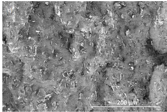
Figure III.55: Micrographies MEB des faciès de rupture des nanocomposites chargés à a) 1 %m, b) 3 %m et c) 10 %m.
