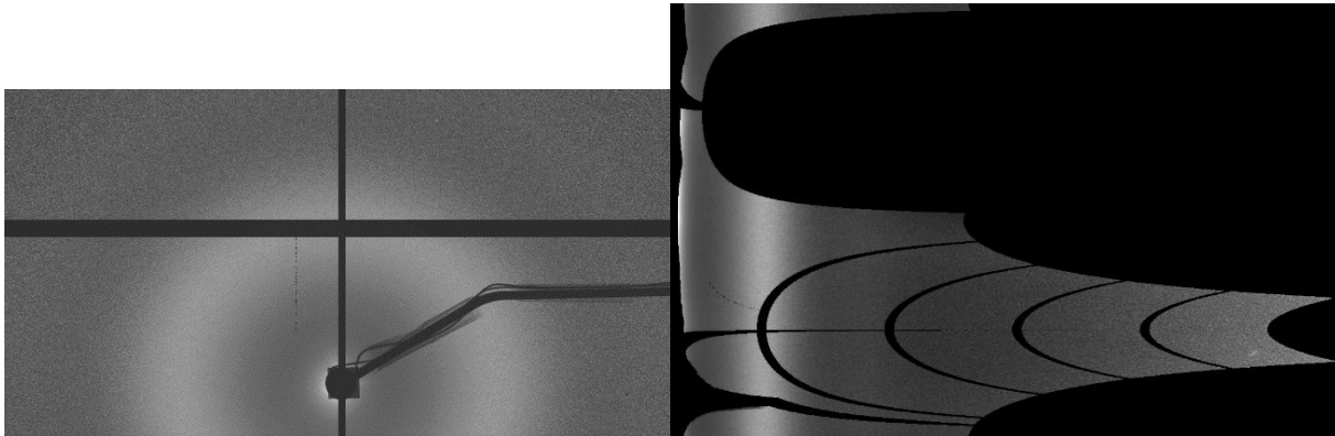
Figure A.2 : Cliché SAXS et « cake » du matériau CA 100 THF 100 1:3
