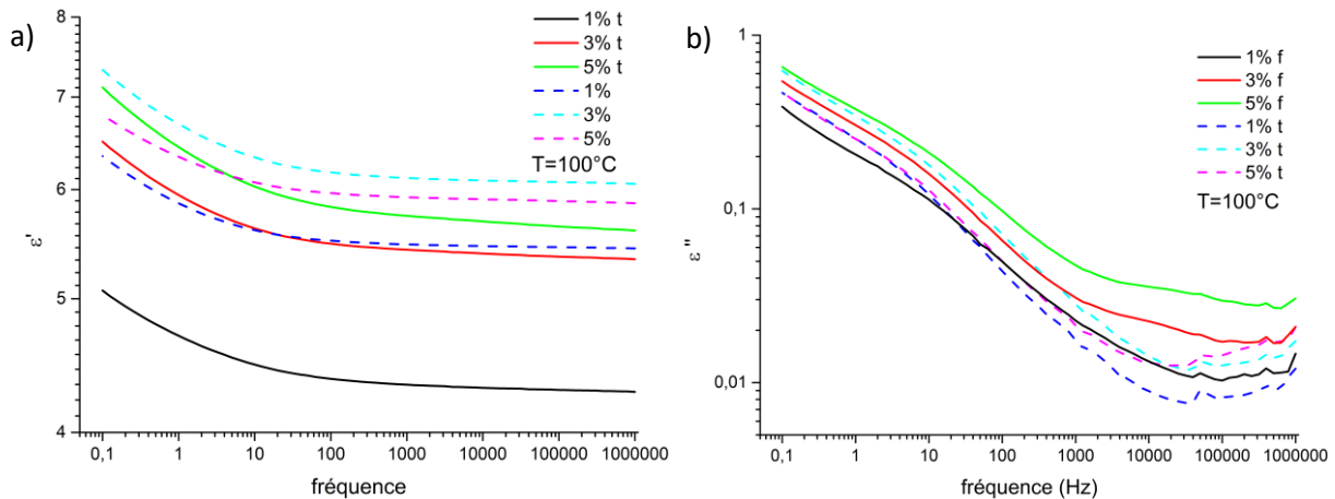
Figure III.67: Comparaison des spectres diélectriques \epsilon' et \epsilon'' en fonction de la fréquence des différentes nanocomposites chargés KNG 180 traités entre 1 et 5 %m à 100°C
