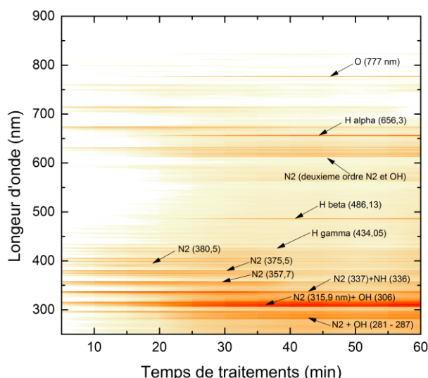
Figure III.8: Evolution du spectre d'émission intégré du plasma au fur et à mesure du traitement.
