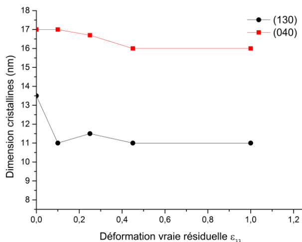
Figure II.49: Évolution des dimensions des lamelles cristallines suivant les plans (130) et (040), calculé par diffraction des rayons X de la matrice CA 100 + T3000 1:1 en fonction de la déformation vraie résiduelle.
