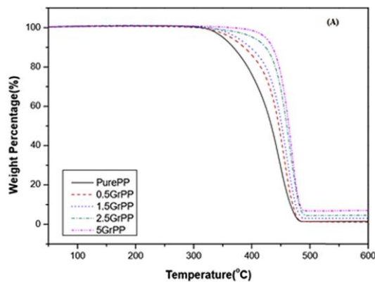
Figure I.50: Evolutions des pertes de masses mesurées par ATG sous air d'un iPP pur et de ses nanocomposites chargés à différents taux de charges graphène [318].
