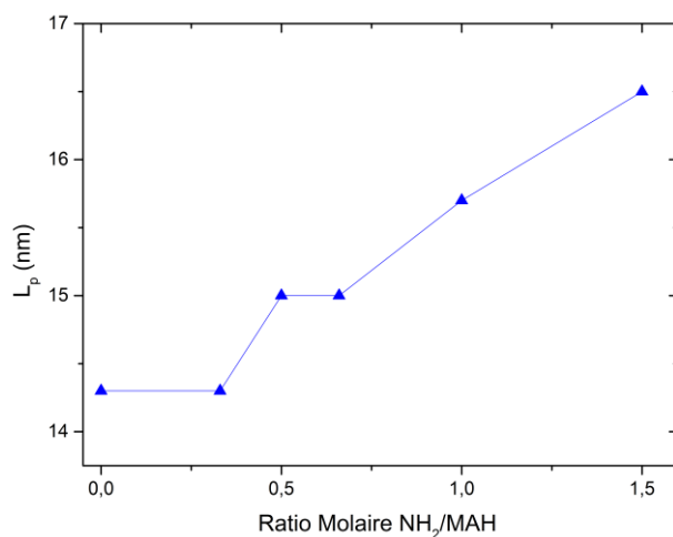
Figure II.17: Evolution de la longue période des matériaux CA 100 + T3000 en fonction du ratio NH 2 :MAH.
