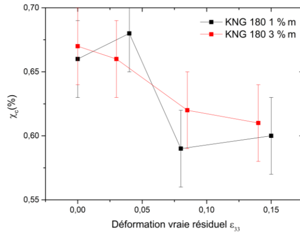
Figure III.77: Evolution du taux de cristallinité estimé par la déconvolution des diffractogrammes DRX
