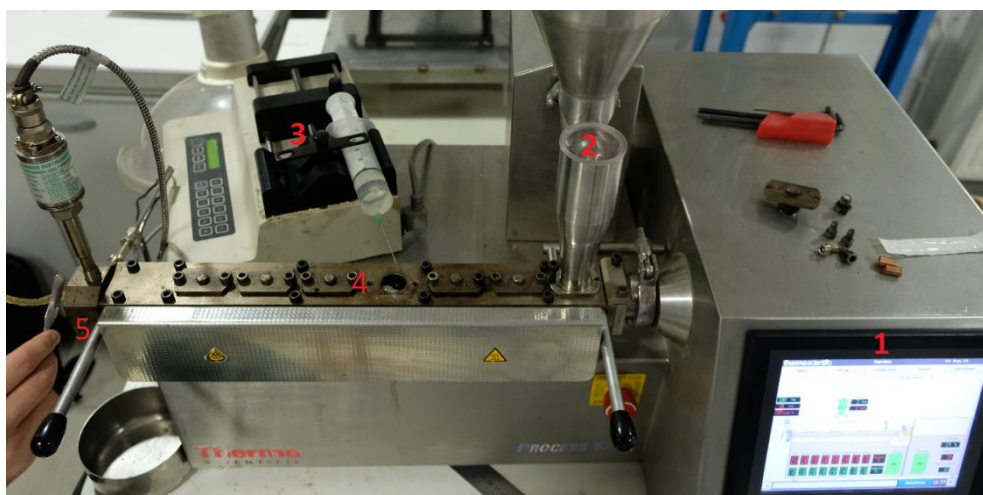
Figure II.2: Processus d'extrusion des matrices réticulées avec en : 1) panneau de contrôle des paramètres d'extrusion, 2) trémie d'alimentation, 3) pousse seringue, 4) zone d'introduction de l'agent réticulant et 5) filière.
