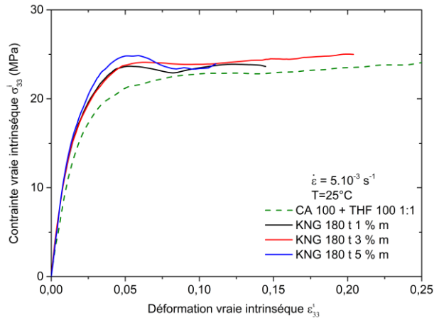
Figure III.69: Comportements mécaniques intrinsèques vrais des nanocomposites chargés de graphite KNG 180 traités.
