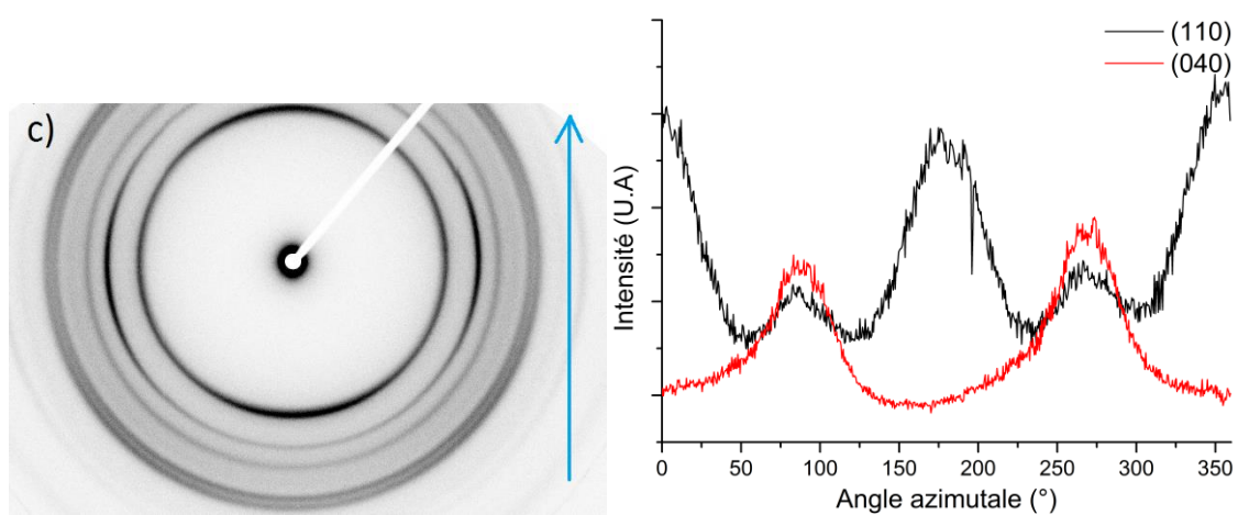
Figure A.51 : Cliché WAXS 2D du CA 100 T3000 1:1 déformé à \epsilon_{33}=0,6 et profile azimutale des plans de diffraction (110) et (040) du polypropylène.
