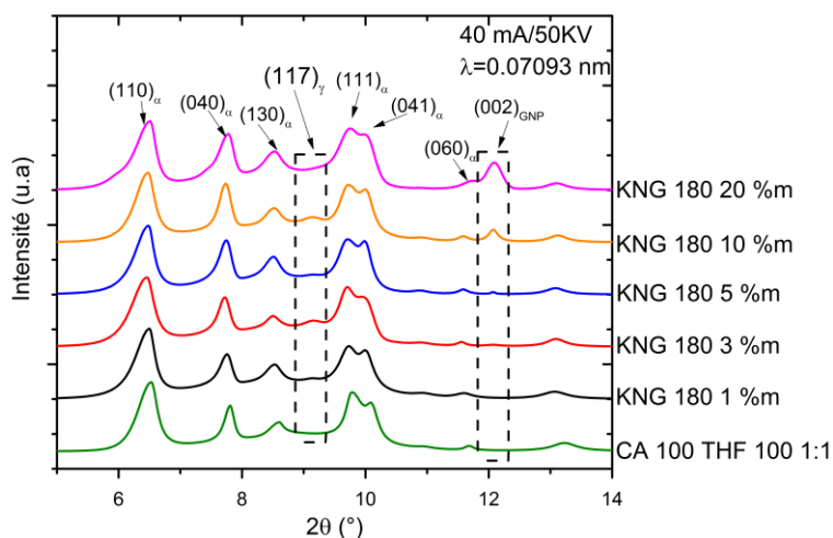
Figure III.42: Diffractogramme DRX des différents nanocomposites chargés KNG 180.
