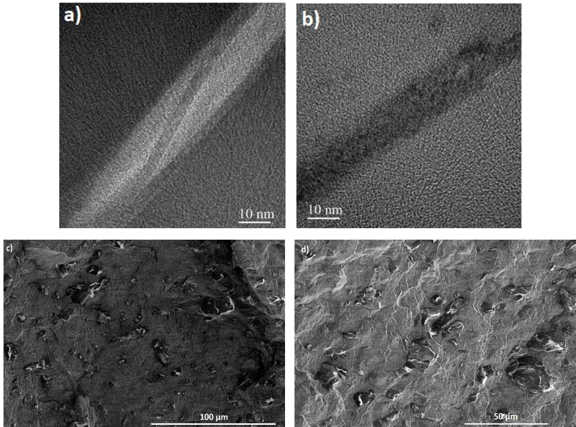
Figure III.64: Micrographies (a) et b)) MET et (c) et d)) MEB du nanocomposite chargé à 3 %m de KNG 180 traités.
