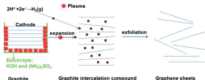
Figure I.30: Mécanisme d'exfoliation du graphène par traitement plasma proposé par Thanh et al. , [281].
