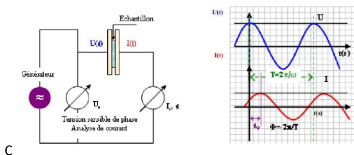
Figure 1: Principe de la mesure en analyse diélectrique [464]
