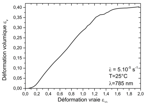
Figure II.35: Évolution de la déformation volumique du CA 100 + THF 100 1:1 lors de la déformation estimée par analyse Raman in situ .
