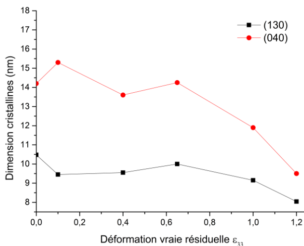
Figure II.37: Évolution des dimensions des lamelles cristallines suivant les normales aux plans (130) et (040), calculées par diffraction des rayons X de la matrice CA 100 THF 100 en fonction de la déformation vraie résiduelle.
