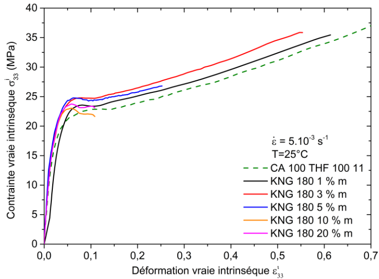
Figure III.54: comportement mécanique intrinsèque vrai des nanocomposites chargés KNG 180
