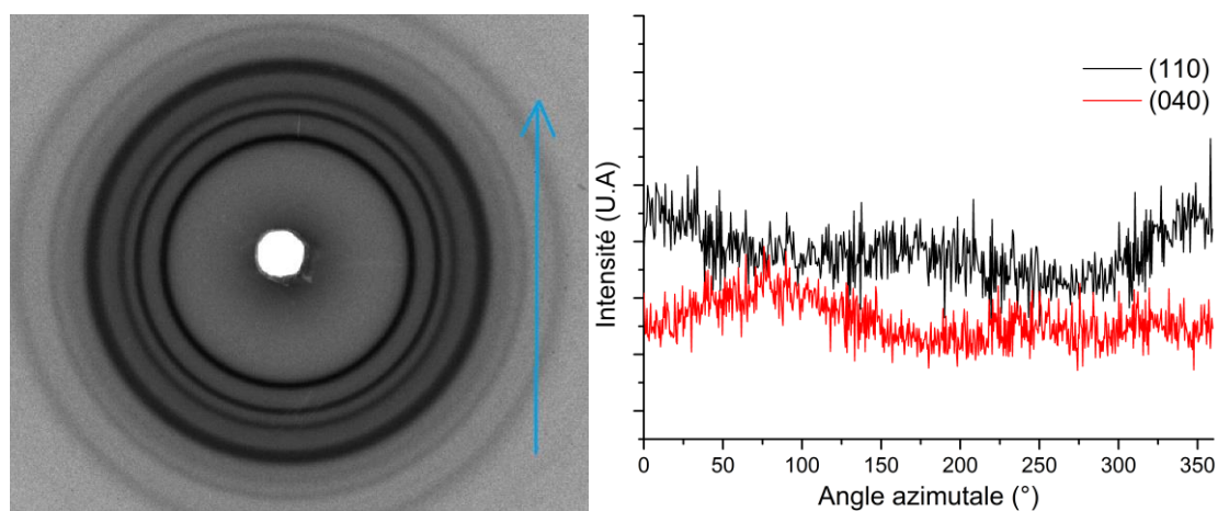
Figure A.19 : Cliché WAXS 2D du CA 100 THF 100 1:2 et profile azimuthale des plans de diffraction (110) et (040) du polypropylène.
