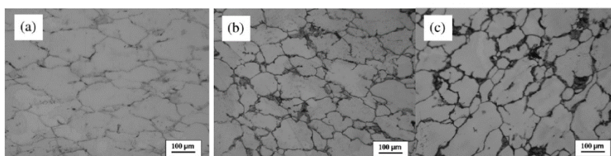
Figure I.38: Micrographie optique du nanocomposite à matrice PEHD pour différents taux en GO : a) 0,05 %vol., b) 0,076 %vol. et c) 0,15 %vol. [313]
