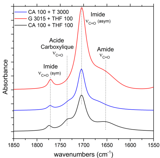
Figure II.20: Comparaison des spectres FTIR des différentes matrices réticulées en ratio 1:1.
