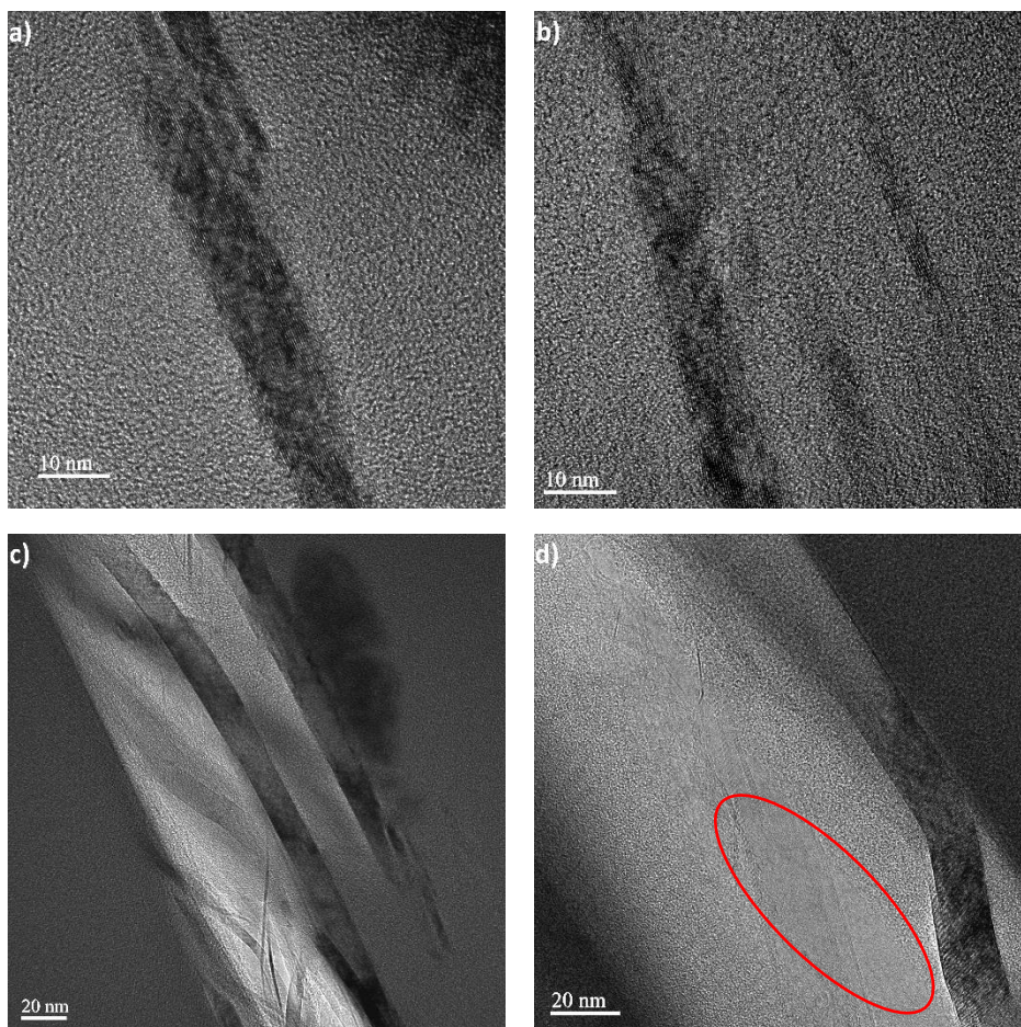
Figure III.45: micrographies MET du nanocomposite chargé à 1 %m de KNG 180.
