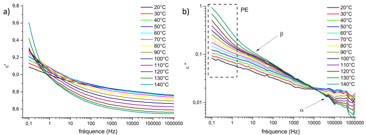
Figure III.49: Spectre diélectrique a) \epsilon' et b) \epsilon'' en fonction de la fréquence du matériau CA 100 THF 100 1:1
