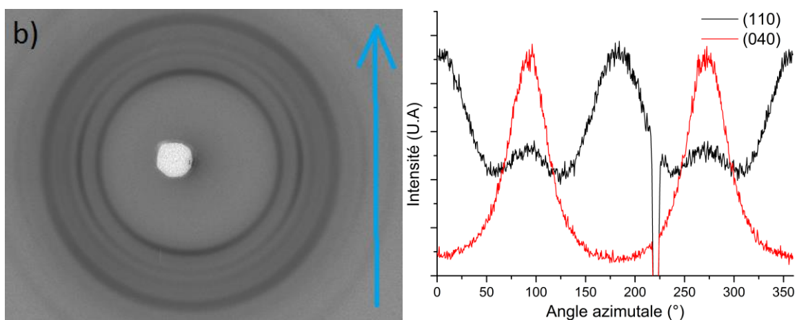
Figure A.37: Cliché WAXS 2D du CA 100 THF 100 1 :1 KNG 180 3% et profile azimutale des plans de diffraction (110) et (040) du polypropylène.
