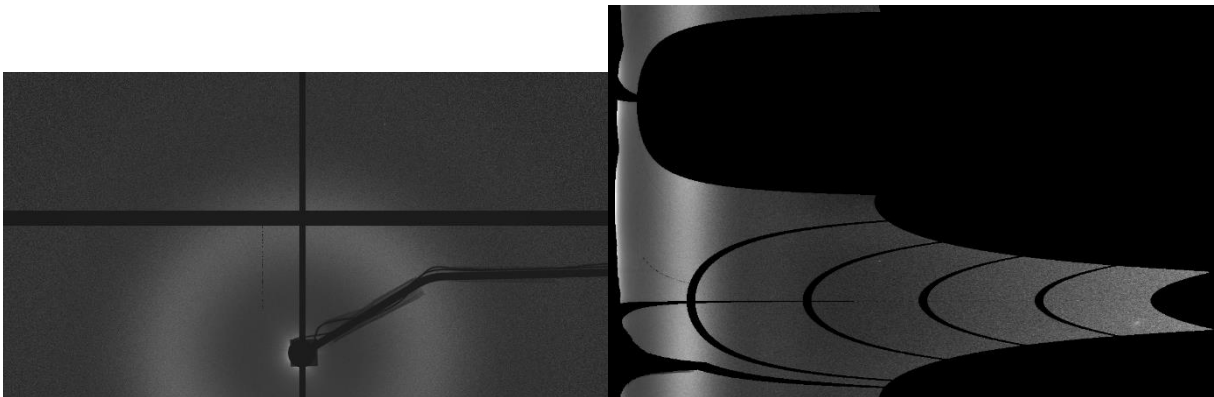
Figure A.6 : Cliché SAXS et « cake » du matériau CA 100 THF 100 3:2
