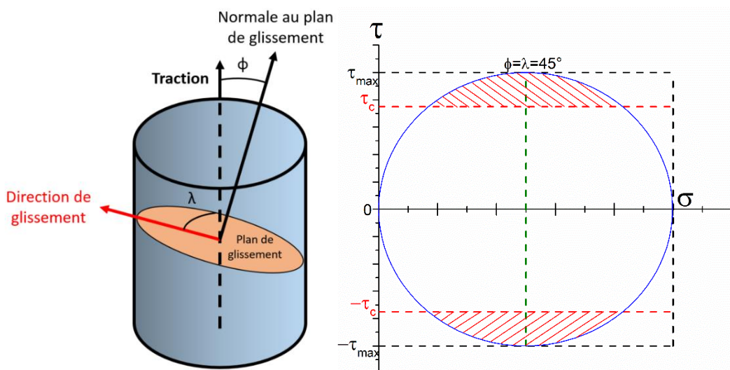
Figure I.12: Construction de la contrainte de cisaillement résolue à un plan de glissement en traction uniaxiale et cercle de Mohr associé, les zones en rouge correspondent aux configurations permettant le glissement lamellaire.
