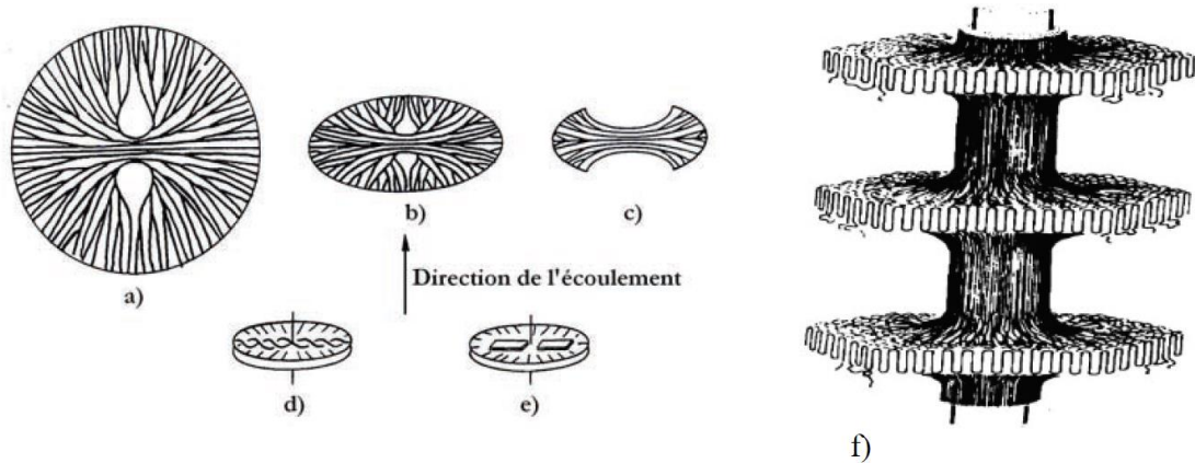
Figure 1.4: Présentation des différentes formes de sphérolites du polypropylène résultant de la mise en forme, a) sphérolite, b) Sphérolite aplati en ellipsoïde, c) disque en forme de gerbe, d) et e) cylindrites et f) « Shish-kebab » [29].
