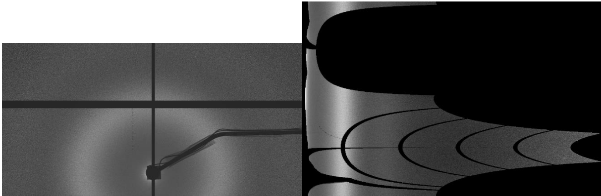
Figure A.1 : Cliché SAXS et « cake » du matériau CA 100 pur
