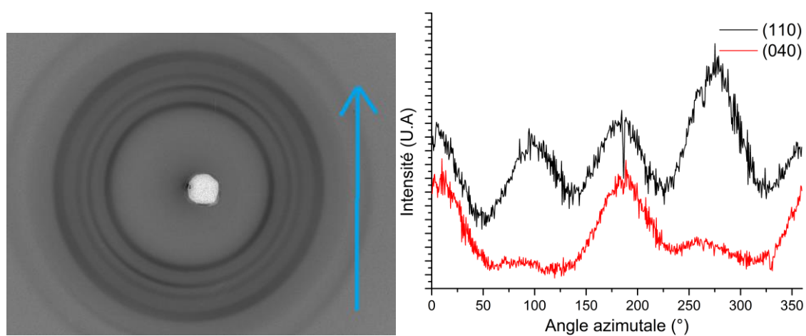
Figure A.33: Cliché WAXS 2D du G3015 THF 100 2:3 et profile azimuthale des plans de diffraction (110) et (040) du polypropylène.
