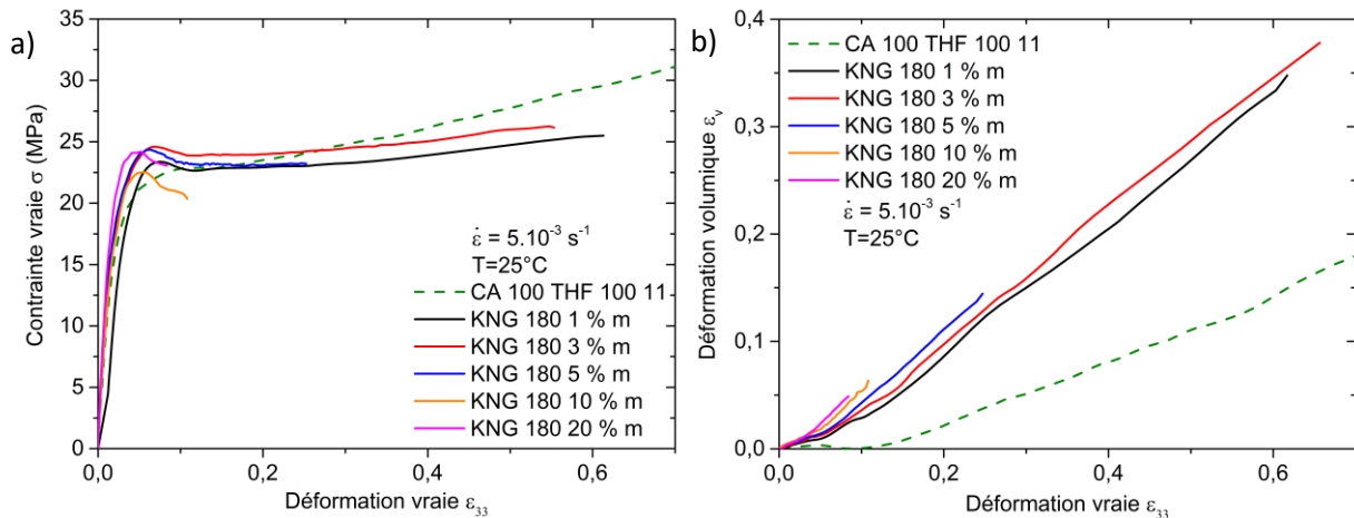
Figure III.53: a) Comportement mécanique vrai des nanocomposites chargés KNG 180, et b) endommagement volumique estimé par VidéoTraction™
