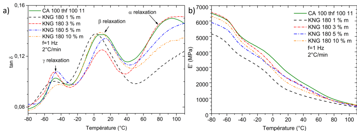
Figure III.56: Analyse DMA des nanocomposites chargés KNG 180, avec a) le facteur de perte et b) le module d'Young
