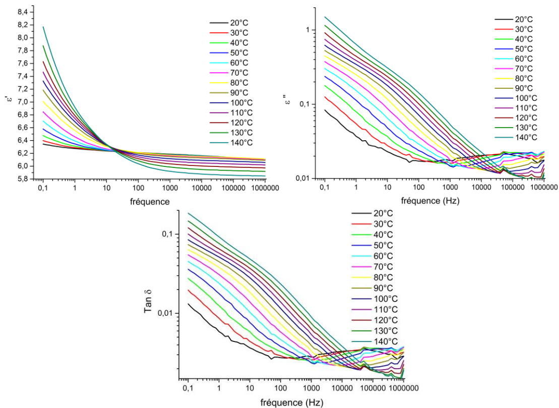
Figure A.61 : Spectre diélectrique \epsilon' , \epsilon'' , et \text{Tan } \delta en fonction de la fréquence du matériau CA 100 THF 100 1:1 KNG 180 3% m
