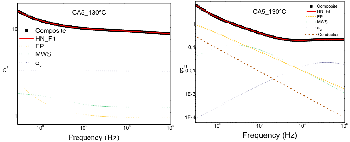
Figure A.68 : Exemple de la déconvolution des spectres diélectriques \epsilon' et \epsilon'' , ici du nanocomposite chargé à 5 % m de KNG 180 traités. Mise en évidence de la polarisation de l'électrode, de la relaxation MWS et des relaxations du PP.
