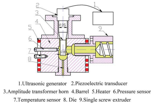
Figure I.40: Schéma du montage pour l'élaboration par extrusion utilisant les ultrasons [325]
