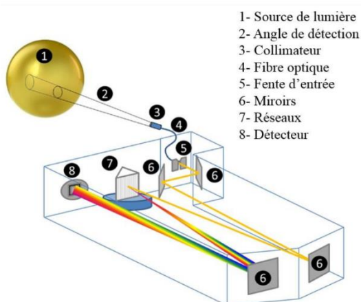
Figure I.64: Structure du monochromateur Jobin-Yvon TRIAX 550 [445].
