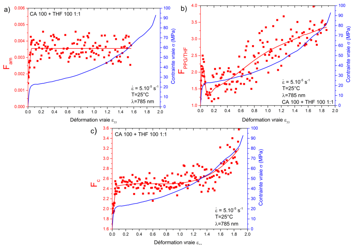
Figure II.27 : Évolution des indices Raman caractérisant l'orientation des chaînes du PP (a) de la phase amorphe, (b) des polyéthers, et (c) des lamelles cristallines lors de la déformation plastique du matériau CA 100 + THF 100 1:1.
