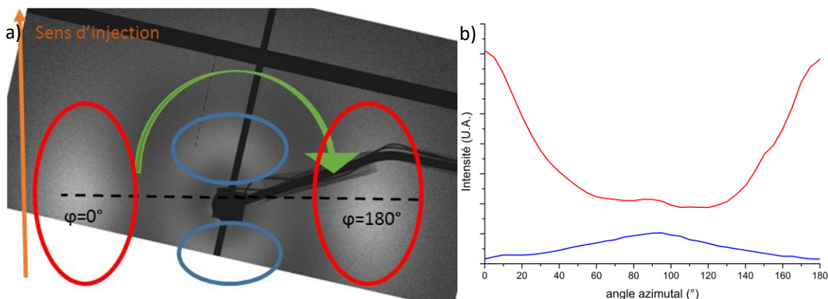
Figure II.13: A) cliché SAXS du matériau G 3015 1:1. Les paires de halos de diffusion sont indiquées en bleu et en rouge. La flèche orange indique la direction d'injection, la verte le sens de l'intégration azimutale. B) évolution de l'intensité diffusée suivant l'angle azimutal au niveau des deux halos de diffusion.
