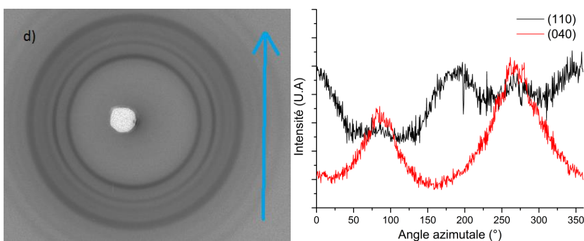
Figure A.39: Cliché WAXS 2D du CA 100 THF 100 1 :1 KNG 180 10% m et profile azimutale des plans de diffraction (110) et (040) du polypropylène.
