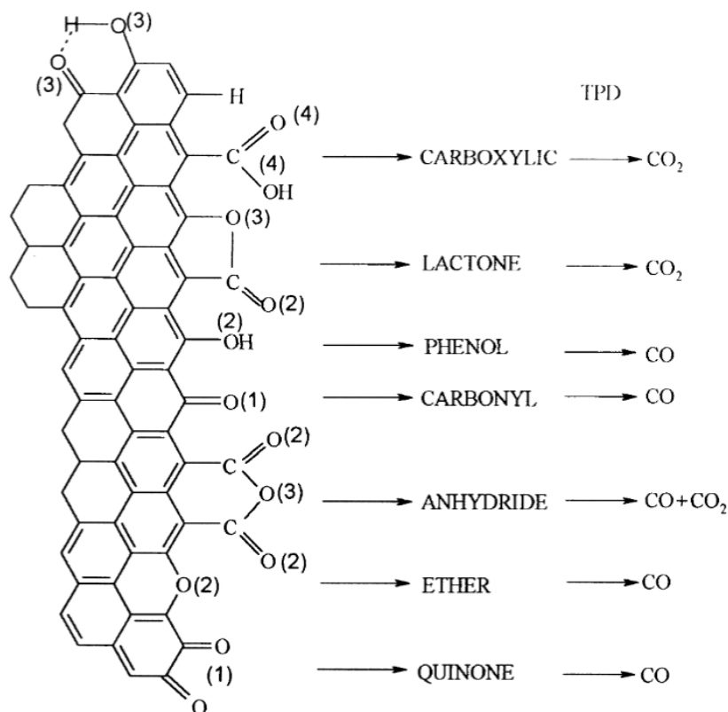
Figure I.33: les différentes fonctions oxygénées pouvant être retrouvées sur une nano-charge de graphite/graphène et les gaz d'émissions associés [291]
