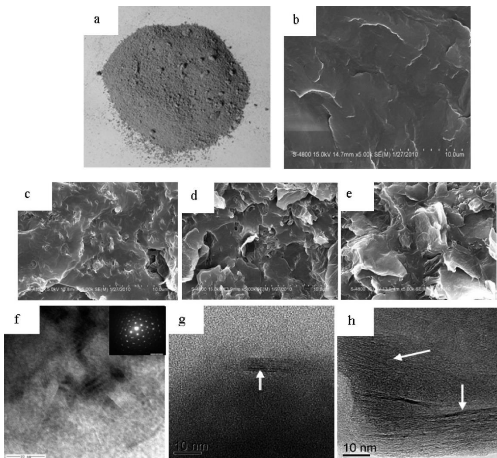
Figure I.35: a) nanocomposite PP/GO sous forme de poudre après élaboration, b) micrographies MEB d'une surface cryo-fracturée de PP vierge, c-e) du composite à respectivement 0,42, 1,52, et 4,9 %m. f-h) Micrographies TEM des composites chargés respectivement à 0,42, 1,52, et 4,9 %m[297].
