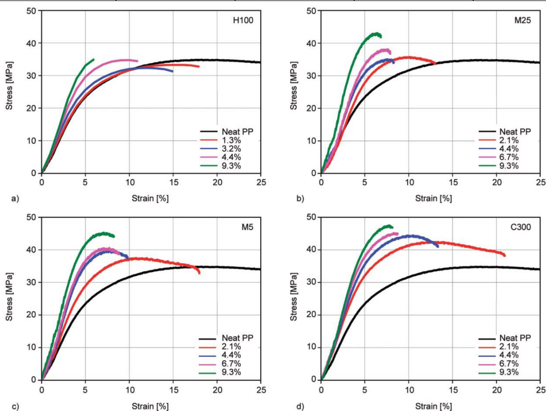
Figure I.47: Evolution contrainte/déformation de différents composites PP/GNP avec a) H100, b) M25, c) M5, et d) C300, pour une concentration volumique allant de 2,1 à 9,3%, des travaux Jun et al. , [339]
