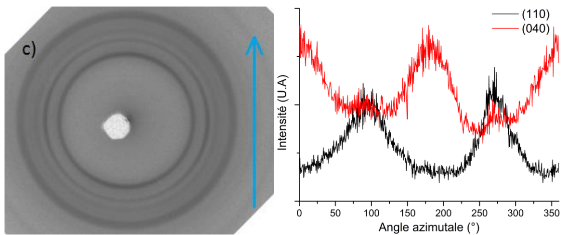
Figure A.43: Cliché WAXS 2D du CA 100 THF 100 1 :1 KNG 180 traité 5% m et profile azimutale des plans de diffraction (110) et (040) du polypropylène.
