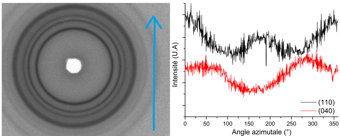
Figure A.26 : Cliché WAXS 2D du CA 100 T3000 1:2 et profile azimuthale des plans de diffraction (110) et (040) du polypropylène.
