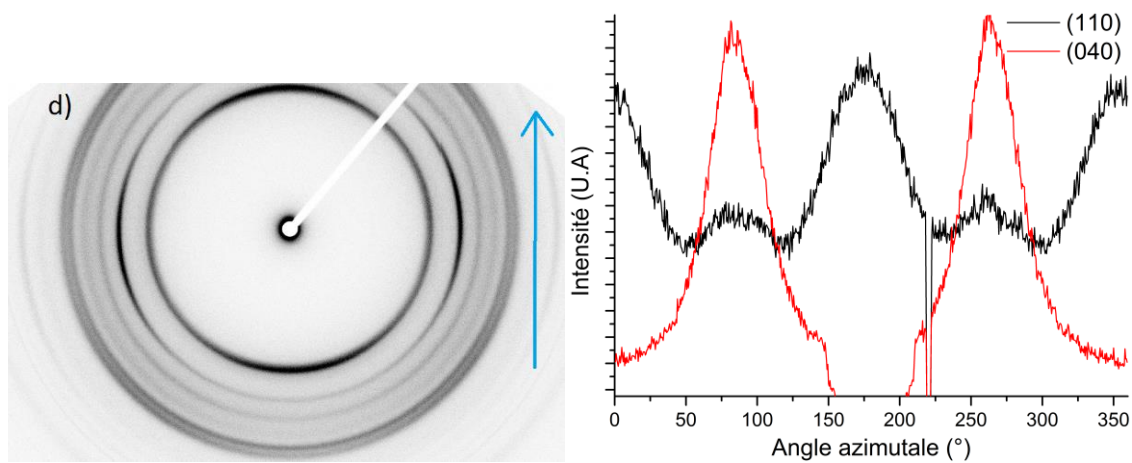
Figure A.59: Cliché WAXS 2D du CA 100 THF 100 1:1 KNG 180 3% m déformé à \epsilon_{33}=0,4 et profile azimutale des plans de diffraction (110) et (040) du polypropylène.
