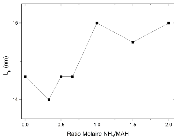
Figure II.11: Evolution de la longue période des matériaux CA 100 + THF 100 en fonction du ratio molaire NH 2 :MAH.
