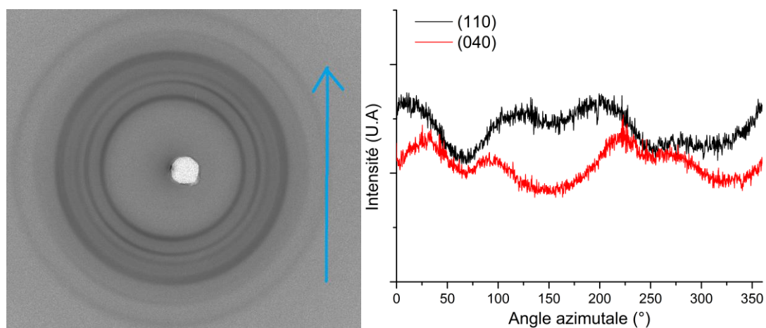
Figure A.32: Cliché WAXS 2D du G3015 THF 100 1:2 et profile azimuthale des plans de diffraction (110) et (040) du polypropylène.
