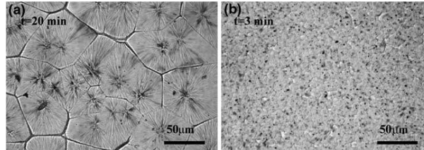
Figure I.45: Morphologie semi-cristalline a) d'un iPP vierge 20 min et b) d'un PP/GNP à 0,01 %m, 3 min après cristallisation isotherme complète à 130°C [336].
