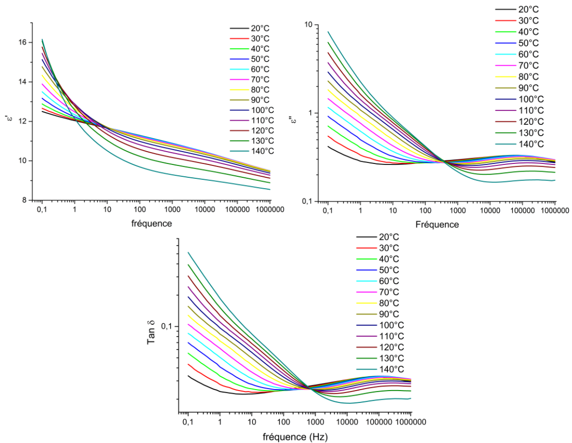
Figure A.64: Spectre diélectrique \epsilon' , \epsilon'' , et \text{Tan } \delta en fonction de la fréquence du matériau CA 100 THF 100 1:1 KNG 180 20% m
