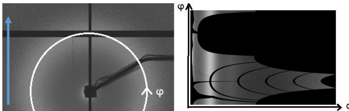
Figure II.10: Transformation polaire du cliché de diffraction SAXS en "Cakes", avec \phi l'angle azimutal, la direction d'injection est indiquée par la flèche.
