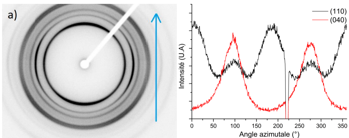
Figure A.28 : Cliché WAXS 2D du CA 100 T3000 1:1 et profile azimuthale des plans de diffraction (110) et (040) du polypropylène.
