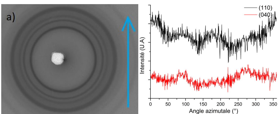
Figure A.36: Cliché WAXS 2D du CA 100 THF 100 1 :1 KNG 180 1% et profile azimutale des plans de diffraction (110) et (040) du polypropylène.
