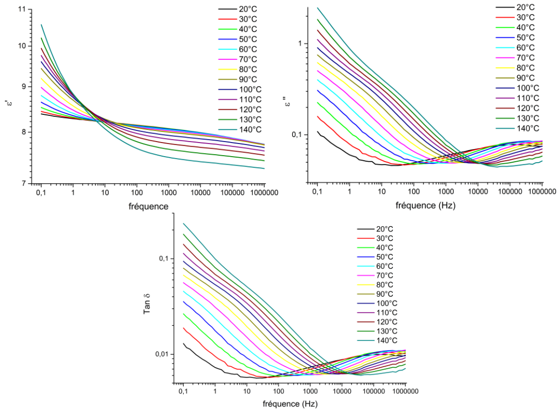
Figure A.63 : Spectre diélectrique \epsilon' , \epsilon'' , et \text{Tan } \delta en fonction de la fréquence du matériau CA 100 THF 100 1:1 KNG 180 10% m
