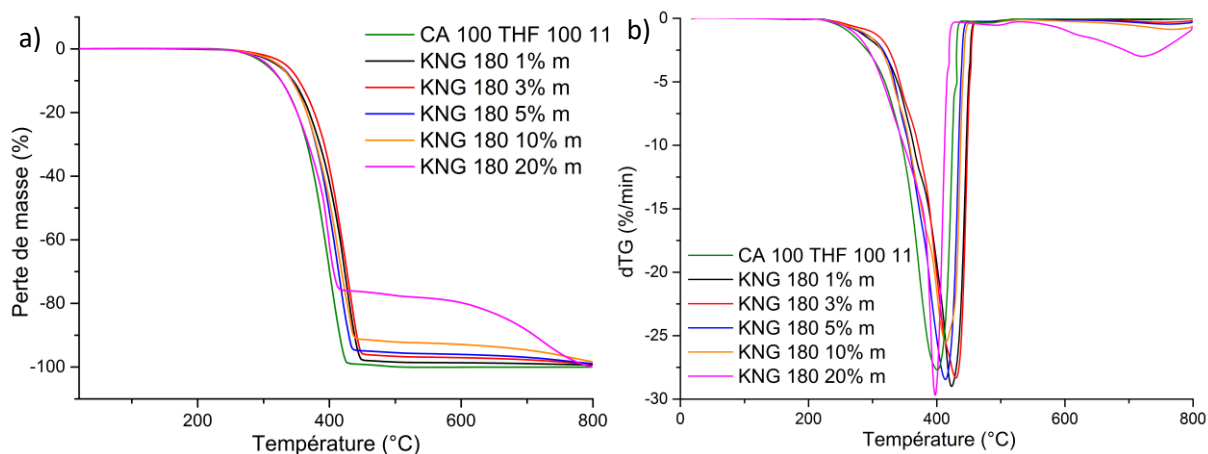
Figure III.37: Evolution de a) la perte de masse et b) dérivé de la perte de masse (droite) des différents nanocomposites chargés KNG 180 de référence.
