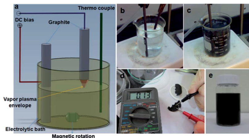
Figure I.29: a) Montage employé pour l'exfoliation du graphite par plasma, b) et c) début et fin d'expérimentation, d) mesure de conductivité du graphène formé et e) dispersion de la nano-charge en solution, tiré de Dang Van Thanh et al. , [281].
