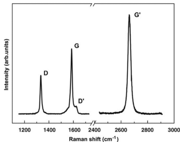
Figure I.32: Spectre Raman d'un bord Feuille de graphène [285].
