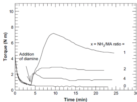
Figure I.10 : Evolution du couple appliqué lors de l'ajout de la diamine pour différents ratios NH 2 :MAH, extrait de Cui et al. , [75].
