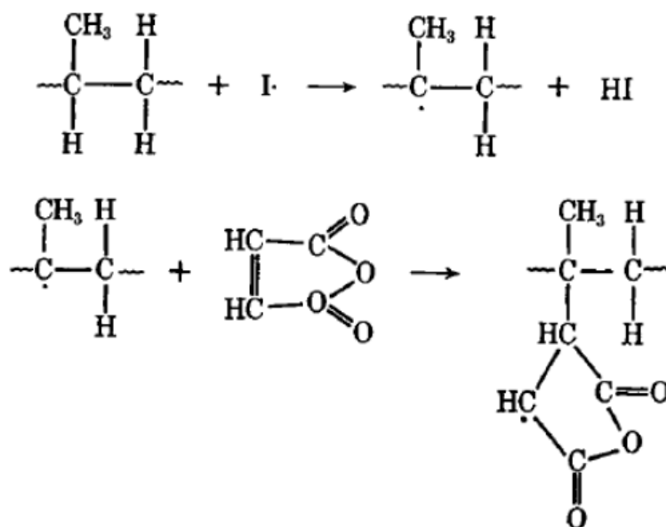
Figure I.6 : Réaction de greffage de l'anhydride maléique par attaque de peroxyde, Minoura et al., 1969 [40].
