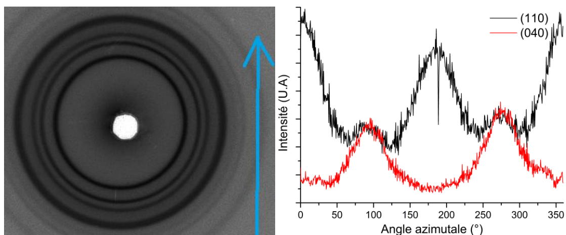
Figure A.23 : Cliché WAXS 2D du CA 100 THF 100 2:1 et profile azimutale des plans de diffraction (110) et (040) du polypropylène.
