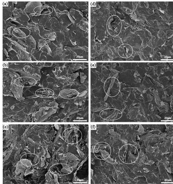
Figure I.41: Micrographies MEB de différents composites PP/GNP sans ultrason (a) à 9 %, (b) 12 %, (c) 15 %, et avec ultrasons (100 W) (d) à 9 %, (e) 12 %, (f) 15 %. [325]
