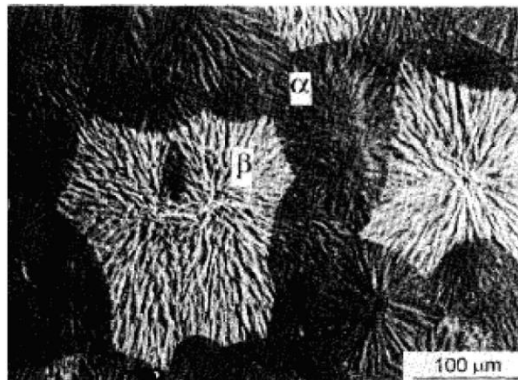
Figure 1.3: Comparaison de la morphologie des sphérolites \alpha , en sombre, et \beta , en clair, révélée par polissage et attaque chimique [25].
