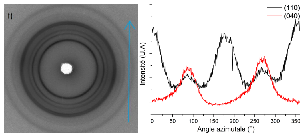
Figure A.49 : Cliché WAXS 2D du CA 100 THF 100 1:1 déformé à \epsilon_{33}=1,5 et profile azimutale des plans de diffraction (110) et (040) du polypropylène.
