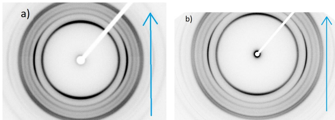
Figure III.74: cliché WAXS 2D des différentes éprouvettes pré déformées avec en a) \epsilon_{33}=0 , b) \epsilon_{33}=0,04 , c) \epsilon_{33}=0,08 , d) \epsilon_{33}=0,15 , du nanocomposite chargé à 1% de graphite KNG 180. Les flèches indiquent le sens de traction appliqué.
