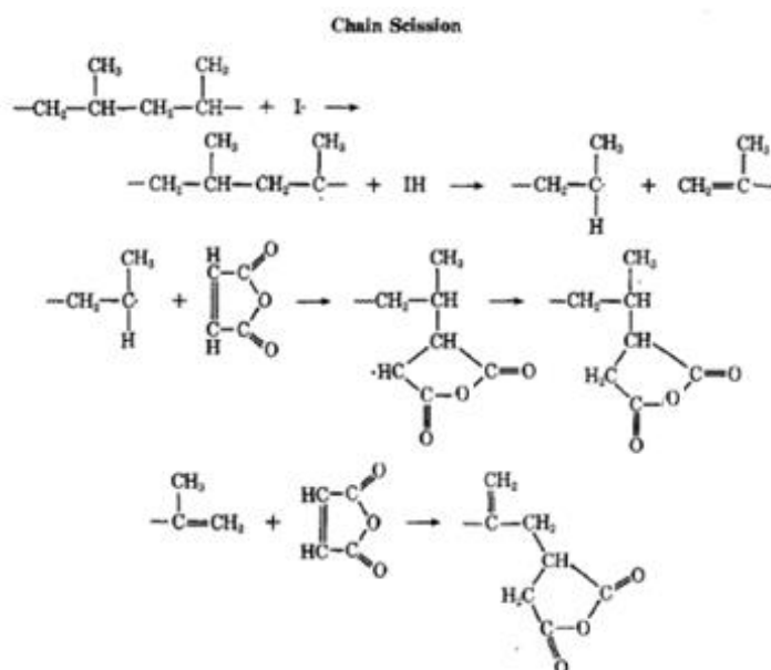
Figure I.7 : Mécanisme de scission des chaînes dû à la présence importante de radicaux libres, Minoura et al., 1969 [40].
