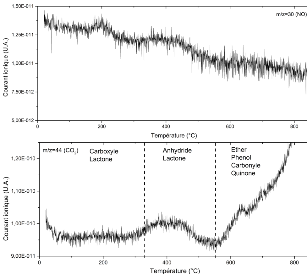
Figure III.28: Evolution de la perte de masse et du spectre de masse m/z = 28 (CO), 30 (NO) et 44 (CO 2 ) de la nano-charge KNG 180 traitée par plasma et greffée diamine lors des essais ATG sous hélium réalisé à 5 °C.min -1 .
