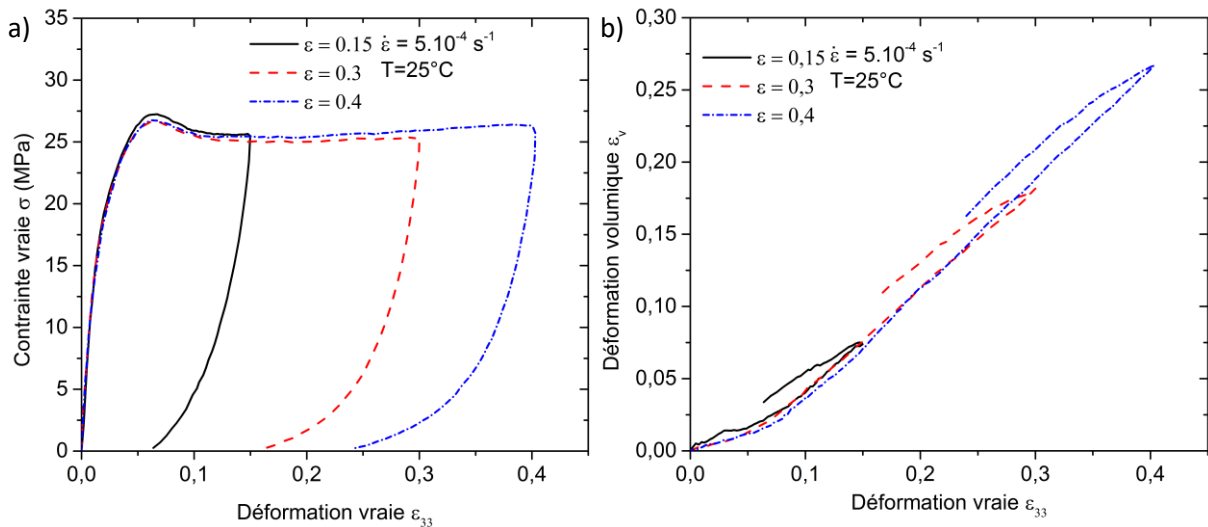
Figure III.73: Résultats mécaniques de la préparation des échantillons déformés en traction uniaxiale avec a) comportement mécanique vrai et b) déformation volumique pour le nanocomposite chargé KNG 180 3 %m.
