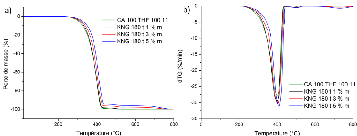
Figure III.57: Evolution de a) la perte de masse et dérivé de b) la perte de masse des différents nanocomposites chargés KNG 180 traités.
