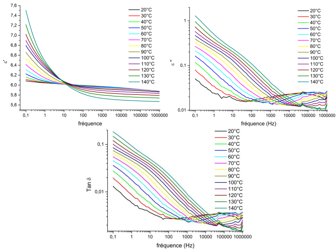
Figure A.62 : Spectre diélectrique \epsilon' , \epsilon'' , et \text{Tan } \delta en fonction de la fréquence du matériau CA 100 THF 100 1:1 KNG 180 5% m
