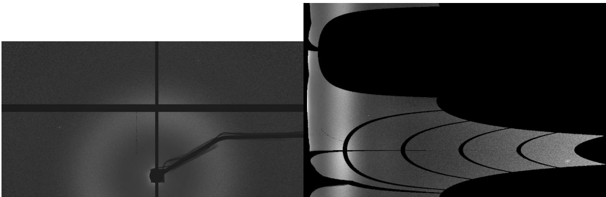
Figure A.7 : Cliché SAXS et « cake » du matériau CA 100 THF 100 2:1
