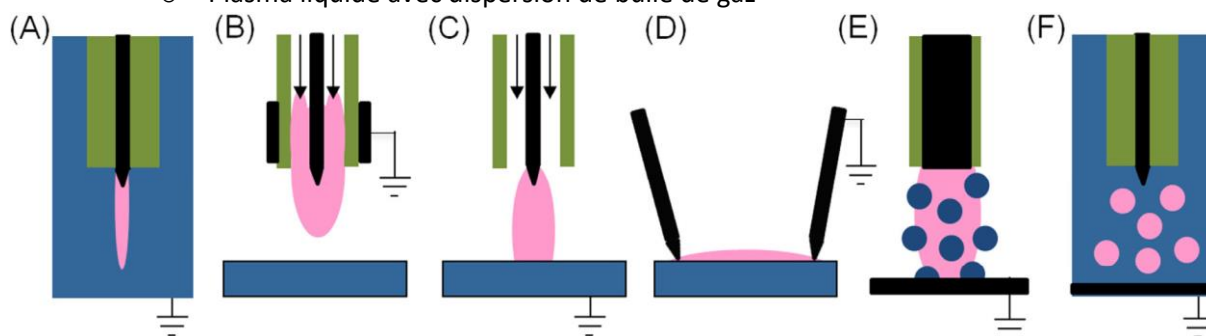
Figure 1.25: Les différents type de décharges, par Bruggeman et al. , (2016) avec en : a) décharge directe, b), c) et d) décharge d'un plasma gazeux, et e) et f), décharge multi phase. Repris de Bruggeman et al. , de 2016 [250]
