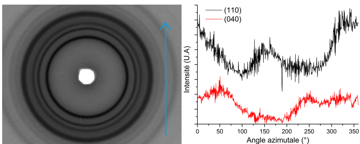
Figure A.27 : Cliché WAXS 2D du CA 100 T3000 2:3 et profile azimuthale des plans de diffraction (110) et (040) du polypropylène.
