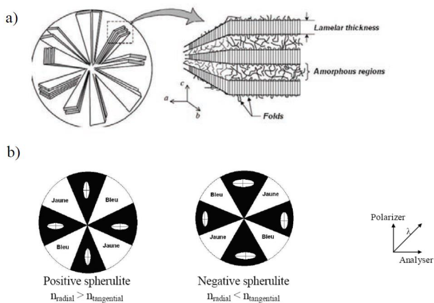
Figure I.1: a) Structure d'un sphérolite et b) représentation d'un sphérolite observé sous lumière polarisée avec lame quart d'onde jaune, n = indice de réfraction [26, 27].
