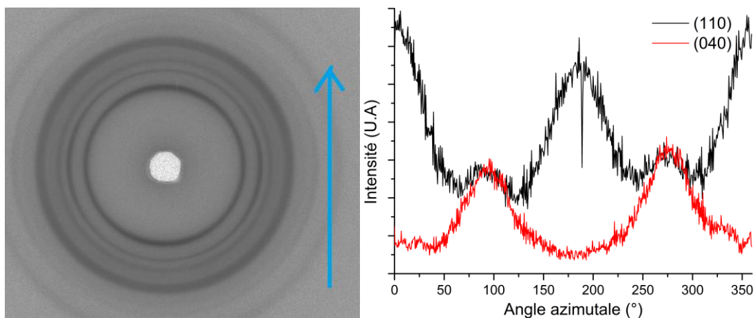
Figure A.22 : Cliché WAXS 2D du CA 100 THF 100 3:2 et profile azimutale des plans de diffraction (110) et (040) du polypropylène.
