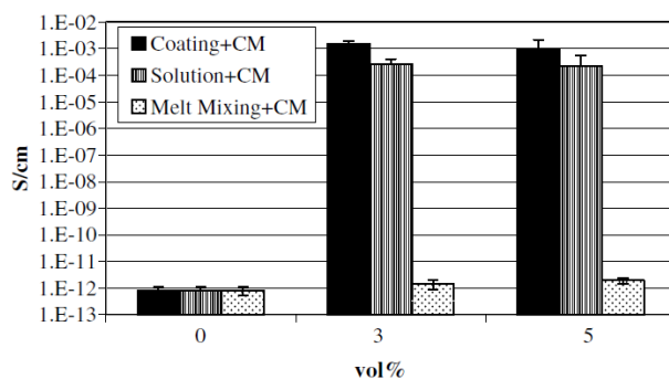
Figure I.49: Evolution de la conductivité électrique au sein de nanocomposites PP/GNP suivant la méthode d'élaboration utilisée [335].
