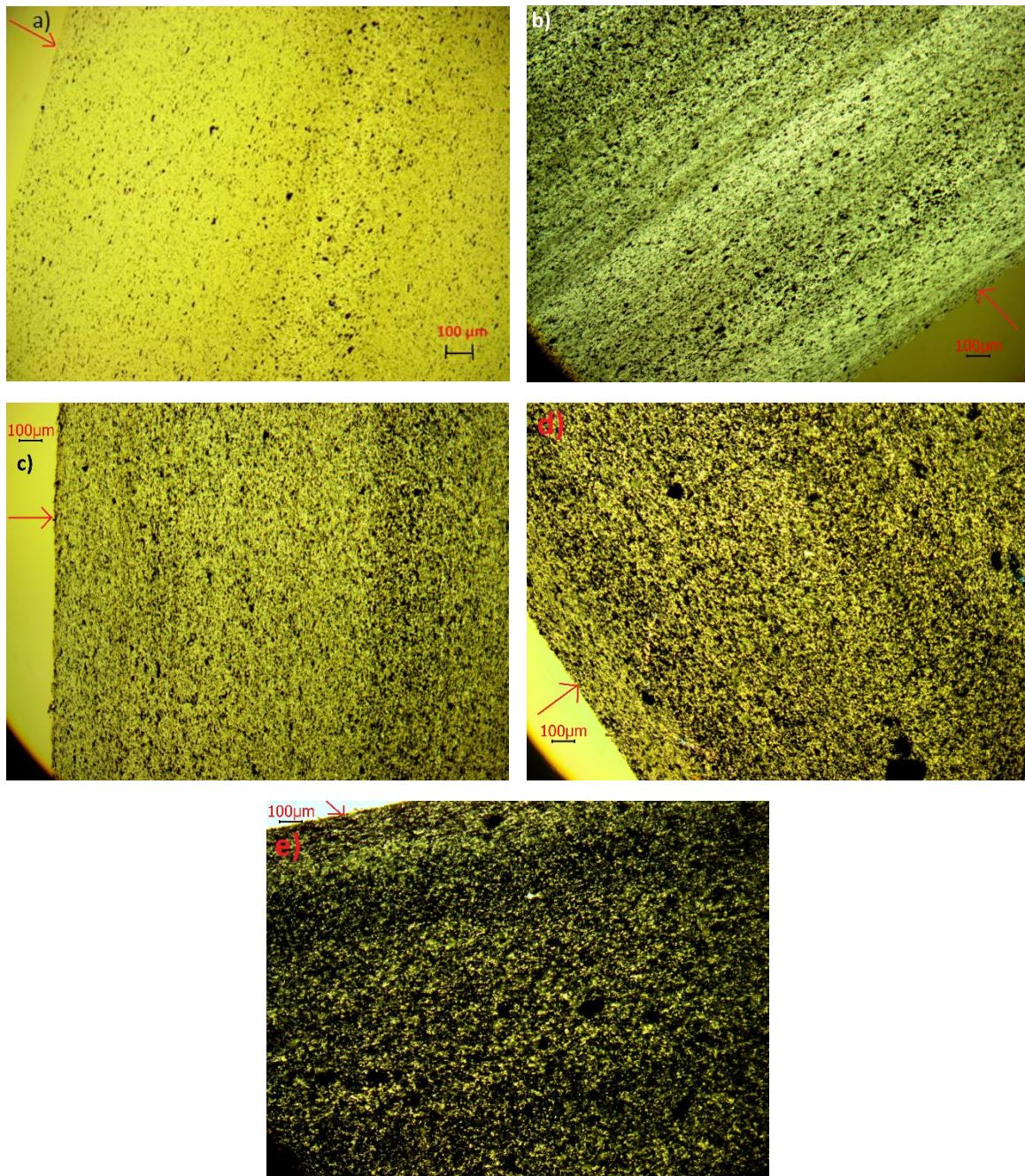
Figure III.35: Observation au microscope optique en transmission des nanocomposites chargés KNG 180 à a) 1 %, b) 3 %, c) 5 %, d) 10 %, e) 20 %. La flèche rouge indique la surface de la plaque injectée.
