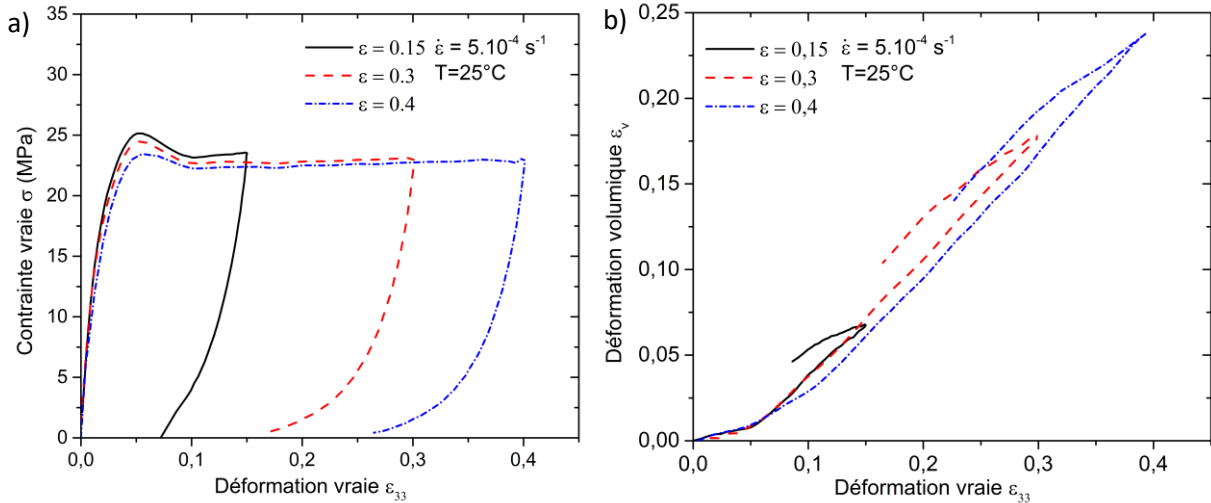
Figure III.72: Résultats mécaniques de la préparation des échantillons déformés en traction uniaxiale avec a) comportement mécanique vrai et b) déformation volumique pour le nanocomposite chargé KNG 180 1 %m.
