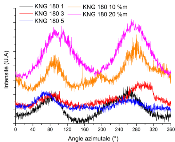
Figure A.44 : profil azimuthal du plan de diffraction (002) du graphite hexagonal des nanocomposites chargés KNG 180 non traités.
