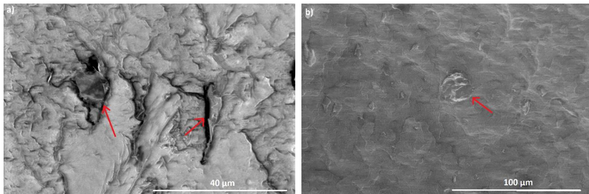
Figure III.44: Micrographies MEB de la surface cryofracturée du nanocomposite chargé à 1 %m de KNG 180. Mise en évidence de la compatibilité charge/matrice.
