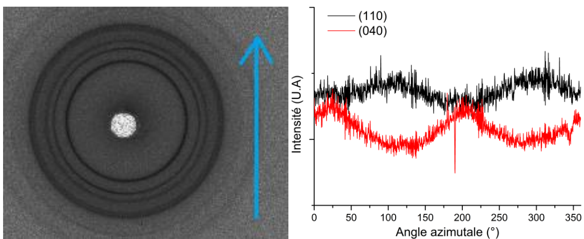
Figure A.35: Cliché WAXS 2D du G3015 THF 100 2:1 et profile azimutale des plans de diffraction (110) et (040) du polypropylène.
