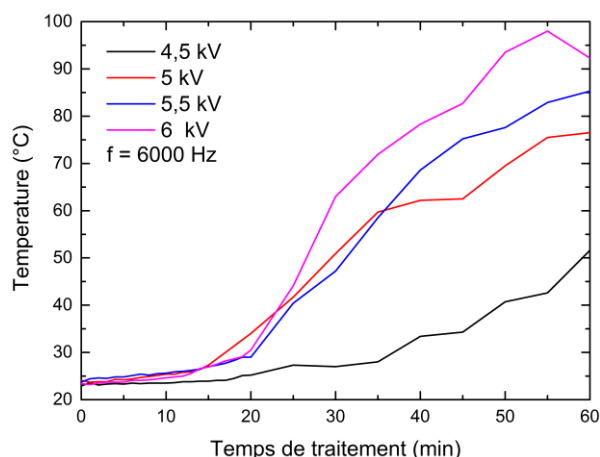
Figure III.4: Evolution de la température lors du traitement à différentes tensions.
