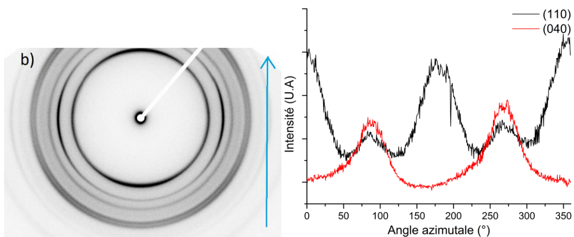
Figure A.50 : Cliché WAXS 2D du CA 100 T3000 1:1 déformé à \epsilon_{33}=0,3 et profile azimutale des plans de diffraction (110) et (040) du polypropylène.
