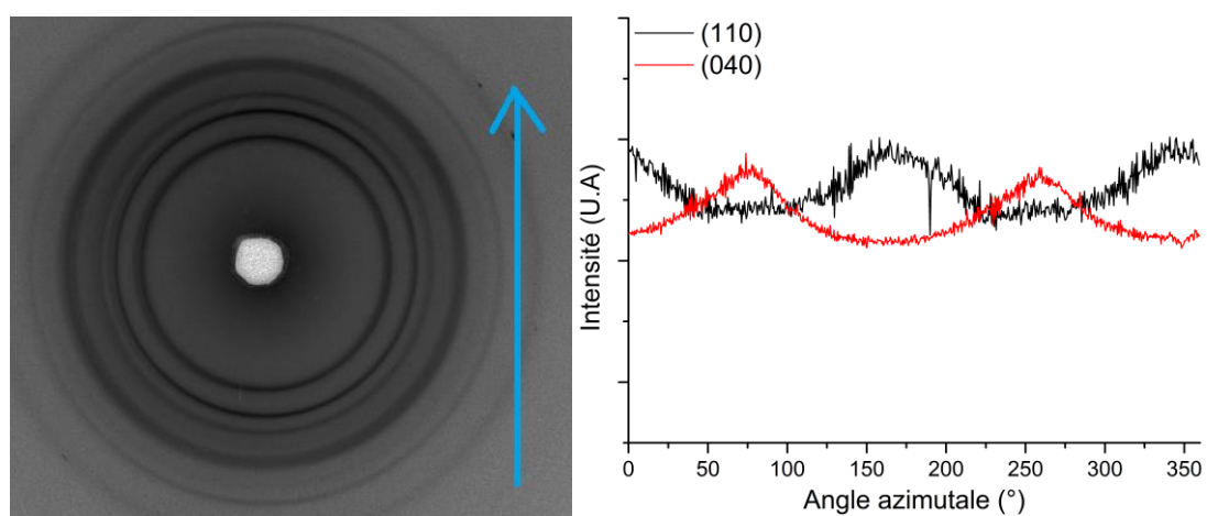
Figure A.21 : Cliché WAXS 2D du CA 100 THF 100 1:1 et profile azimutale des plans de diffraction (110) et (040) du polypropylène.
