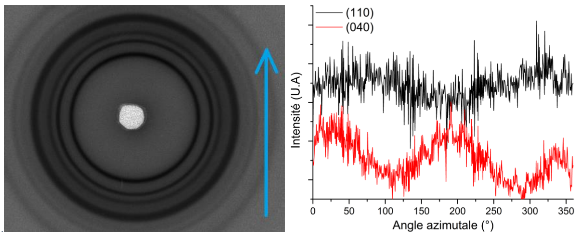
Figure A.20 : Cliché WAXS 2D du CA 100 THF 100 2:3 et profile azimutale des plans de diffraction (110) et (040) du polypropylène.
