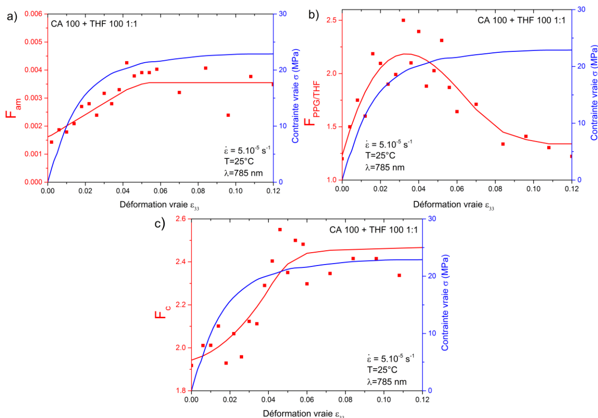
Figure II.28 : Évolution des indices Raman caractérisant l'orientation des chaînes du PP (a) de la phase amorphe, (b) des polyéthers, et (c) des lamelles cristallines lors de la déformation viscoélastique et du début de la déformation plastique du matériau CA 100 + THF 100 1:1.
