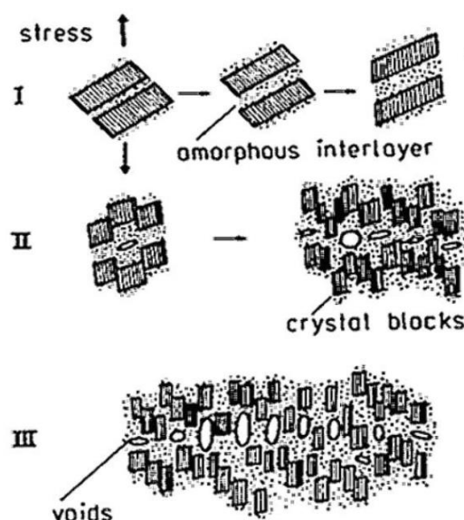
Figure I.17: Phénomène de cavitation de la phase amorphe lors d'un essai de traction [100].
