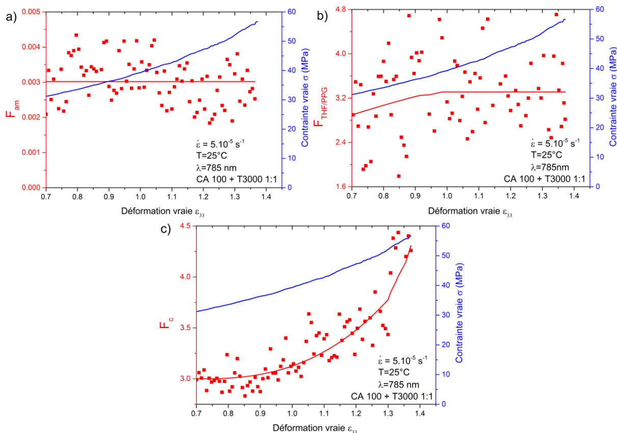
Figure II.43 : Évolution des indices Raman caractérisant l'orientation des chaînes du PP (a) de la phase amorphe, (b) des polyéthers, et (c) des lamelles cristallines en fin de durcissement structural du matériau CA 100 + T3000 1:1.
