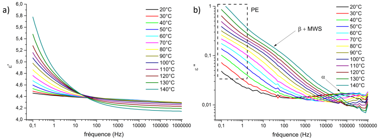
Figure III.66: Spectres diélectriques a) \epsilon' et b) \epsilon'' en fonction de la fréquence du nanocomposite chargée à 1 %m de KNG 180 traités par plasma
