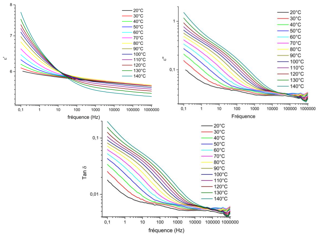
Figure A.67 : Spectre diélectrique \epsilon' , \epsilon'' , et \text{Tan } \delta en fonction de la fréquence du matériau CA 100 THF 100 1:1 KNG 180 traité 5% m
