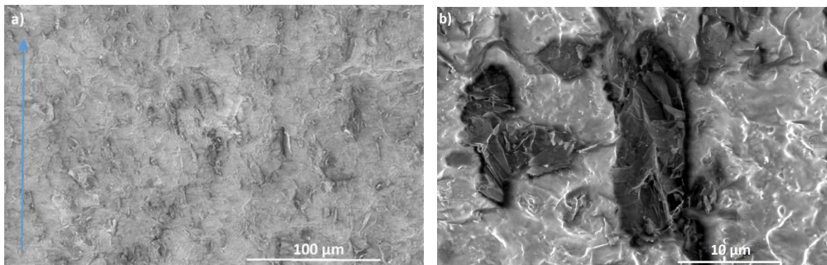
Figure III.47: Micrographie MEB du nanocomposite chargé à 5 %m de KNG 180. La flèche bleue en a) indique la direction d'injection.
